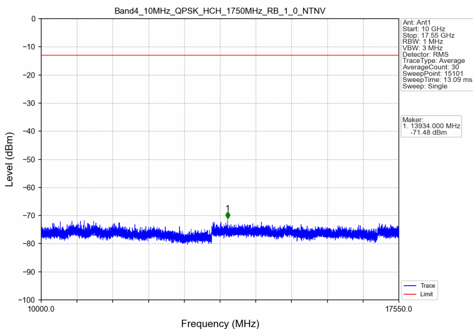
Band4_10MHz_QPSK_HCH_1750MHz_RB_1_0_NTNV
