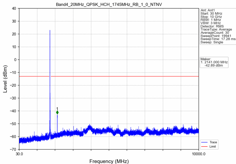
Band4_20MHz_QPSK_HCH_1745MHz_RB_1_0_NTNV
