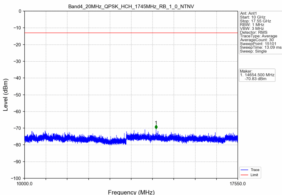
Band4_20MHz_QPSK_HCH_1745MHz_RB_1_0_NTNV
