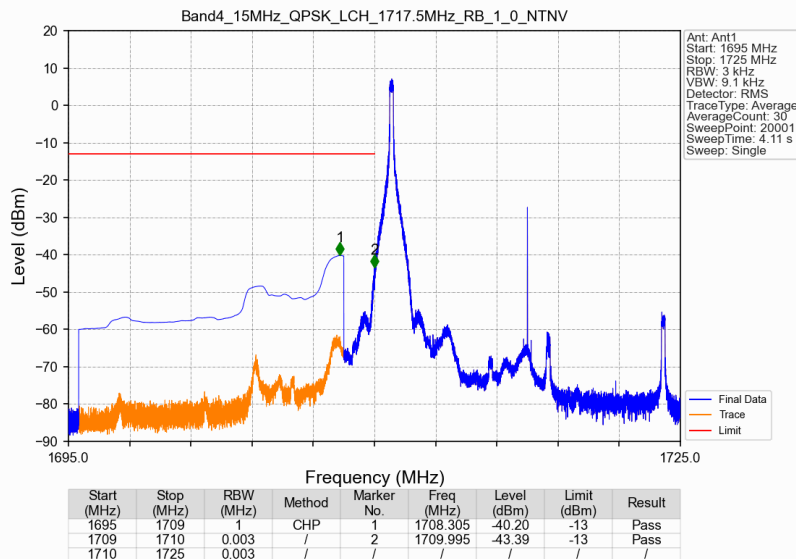
Band4_15MHz_QPSK_LCH_1717.5MHz_RB_1_0_NTNV
