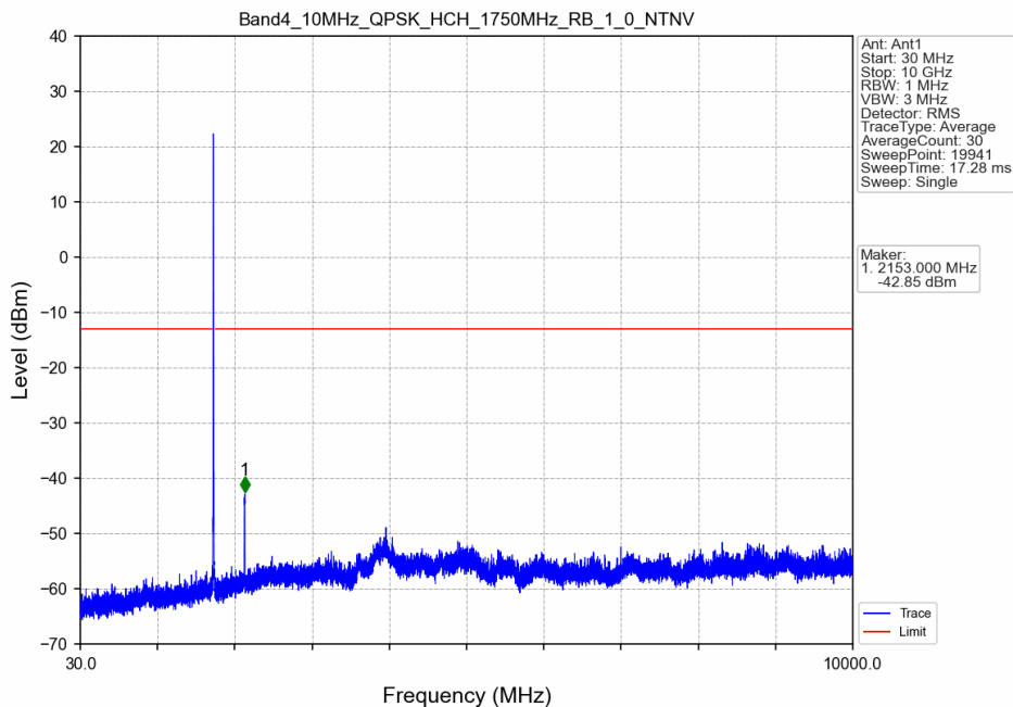
Band4_10MHz_QPSK_HCH_1750MHz_RB_1_0_NTNV
