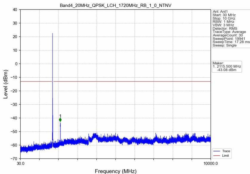
Band4_20MHz_QPSK_LCH_1720MHz_RB_1_0_NTNV
