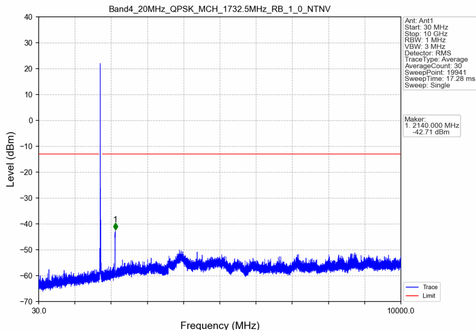
Band4_20MHz_QPSK_MCH_1732.5MHz_RB_1_0_NTNV
