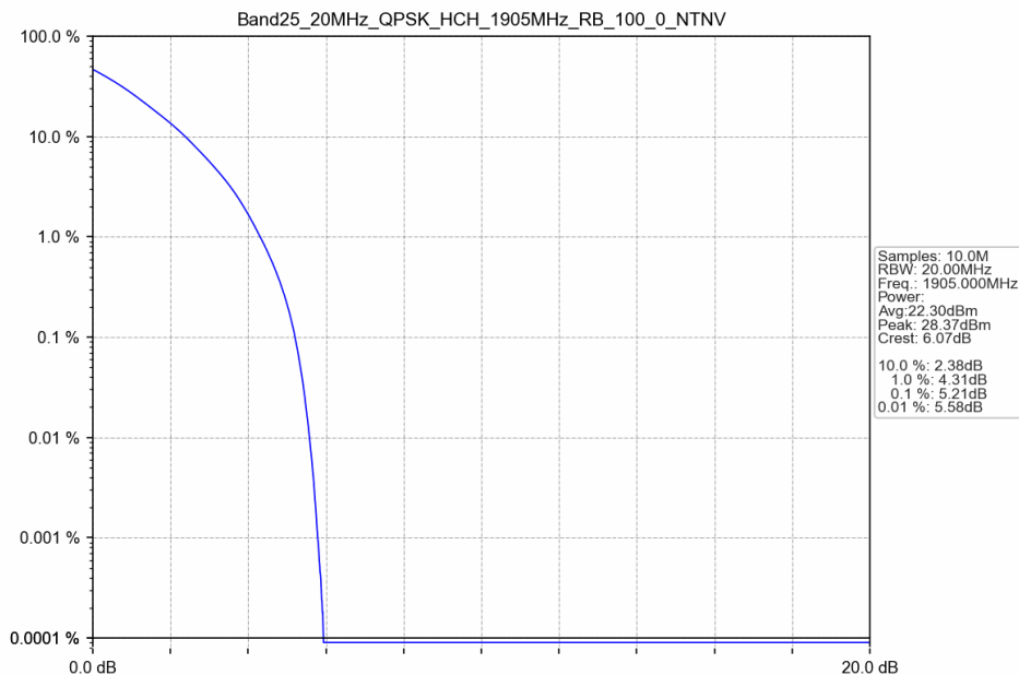
Band25_20MHz_QPSK_HCH_1905MHz_RB_100_0_NTNV
