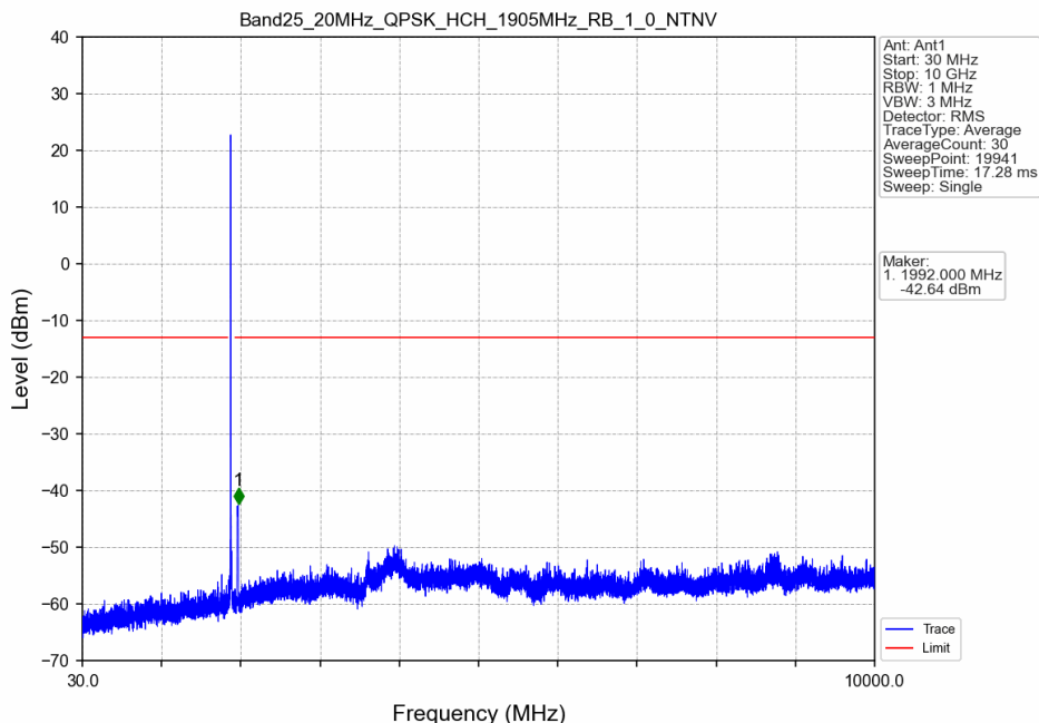
Band25_20MHz_QPSK_HCH_1905MHz_RB_1_0_NTNV
