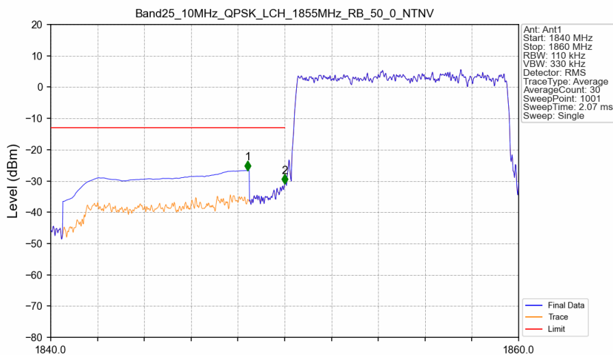
Band25_10MHz_QPSK_LCH_1855MHz_RB_50_0_NTNV
