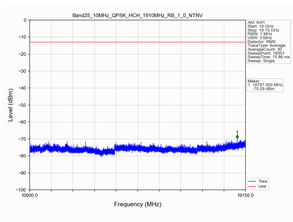
Band25_10MHz_QPSK_HCH_1910MHz_RB_1_0_NTNV
