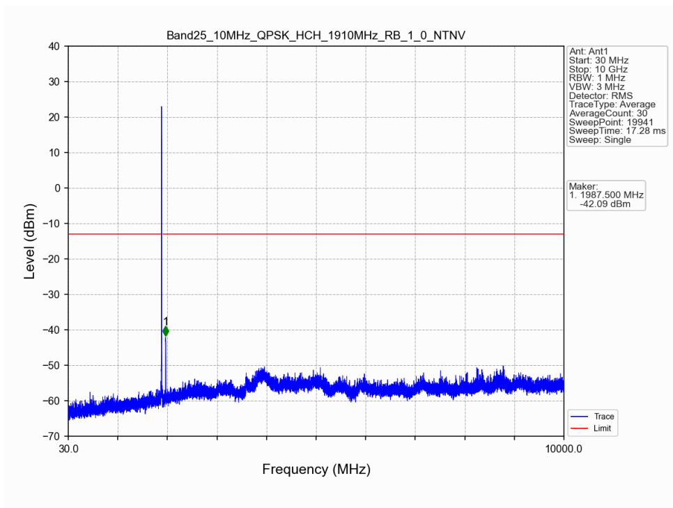
Band25_10MHz_QPSK_HCH_1910MHz_RB_1_0_NTNV
