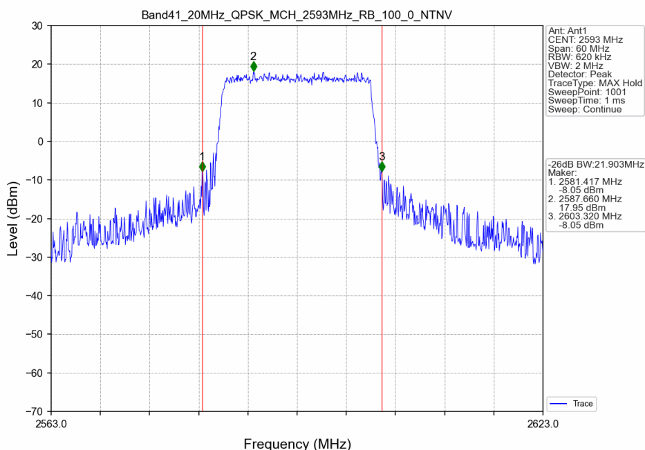
Band41_20MHz_QPSK_MCH_2593MHz_RB_100_0_NTNV
