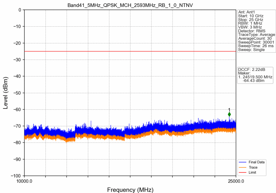
Band41_5MHz_QPSK_MCH_2593MHz_RB_1_0_NTNV
