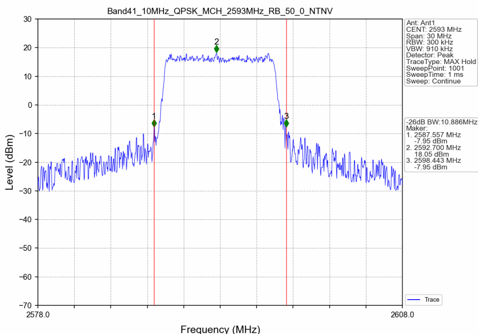
Band41_10MHz_QPSK_MCH_2593MHz_RB_50_0_NTNV
