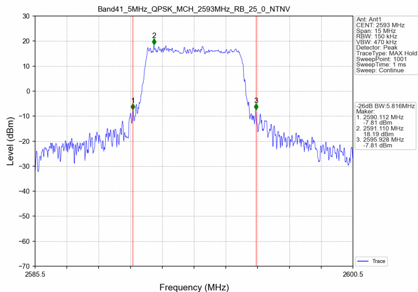
Band41_5MHz_QPSK_MCH_2593MHz_RB_25_0_NTNV
