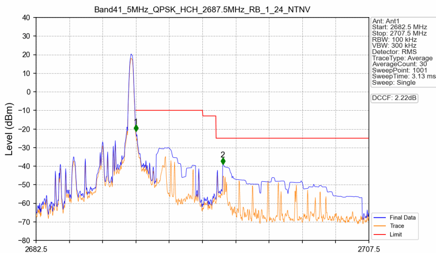
Band41_5MHz_QPSK_HCH_2687.5MHz_RB_1_24_NTNV
