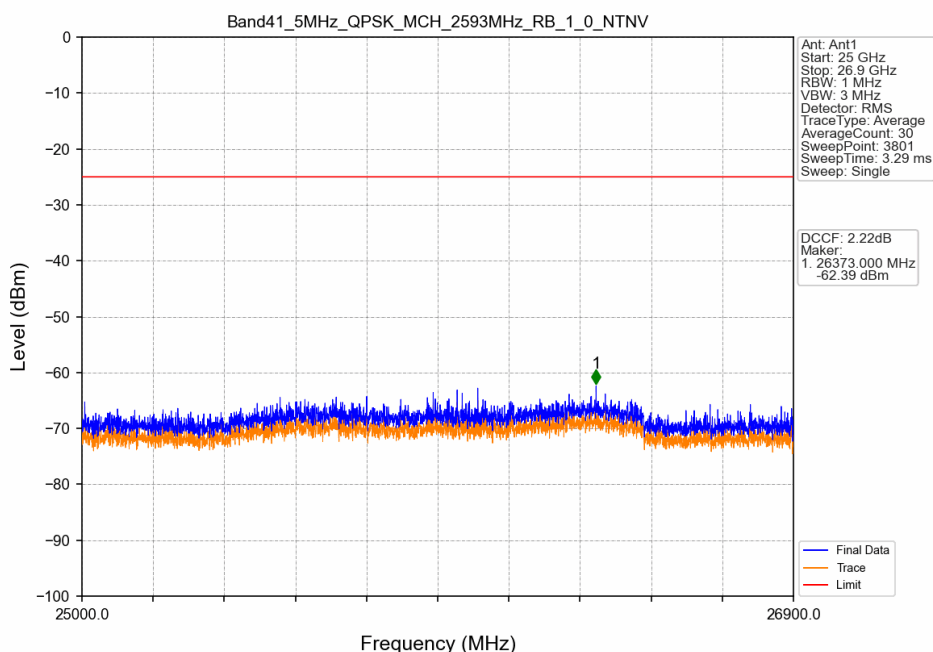
Band41_5MHz_QPSK_MCH_2593MHz_RB_1_0_NTNV
