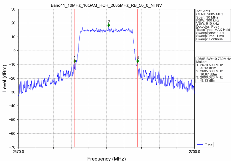
Band41_10MHz_16QAM_HCH_2685MHz_RB_50_0_NTNV
