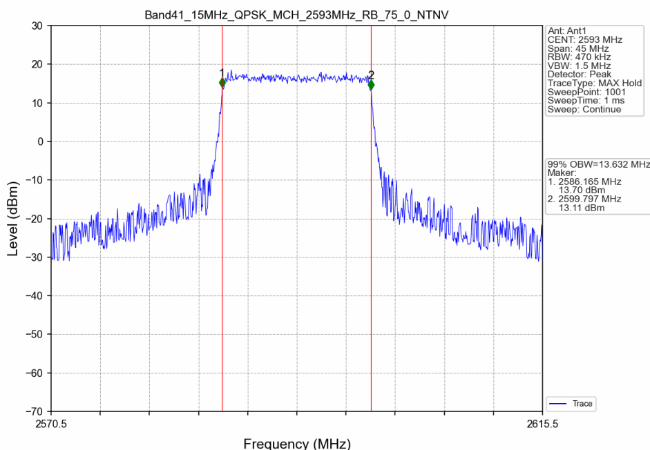
Band41_15MHz_QPSK_MCH_2593MHz_RB_75_0_NTNV
