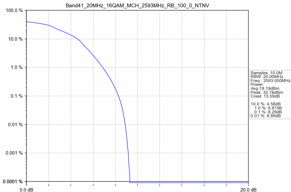
Band41_20MHz_16QAM_MCH_2593MHz_RB_100_0_NTNV
