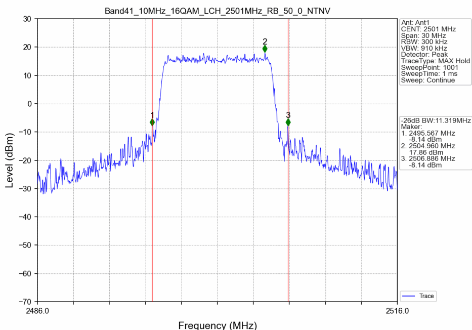
Band41_10MHz_16QAM_LCH_2501MHz_RB_50_0_NTNV
