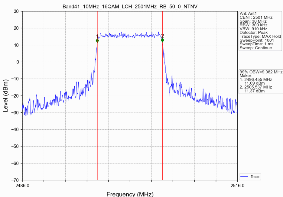
Band41_10MHz_16QAM_LCH_2501MHz_RB_50_0_NTNV
