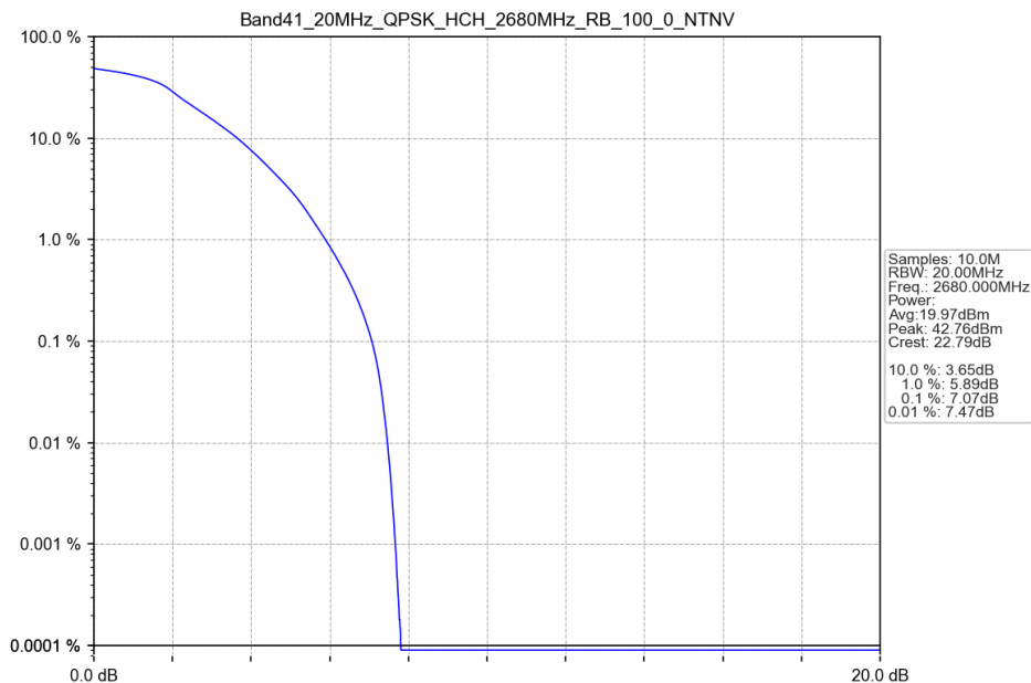
Band41_20MHz_QPSK_HCH_2680MHz_RB_100_0_NTNV
