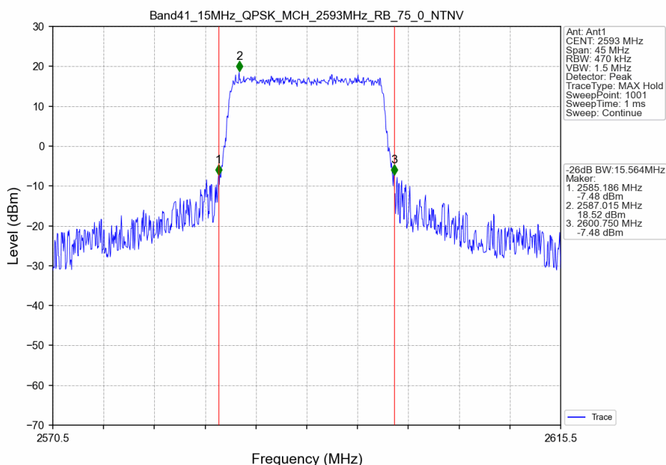
Band41_15MHz_QPSK_MCH_2593MHz_RB_75_0_NTNV
