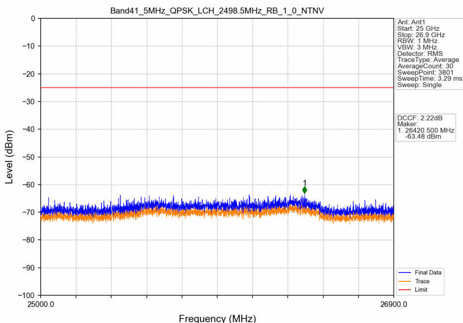
Band41_5MHz_QPSK_LCH_2498.5MHz_RB_1_0_NTNV
