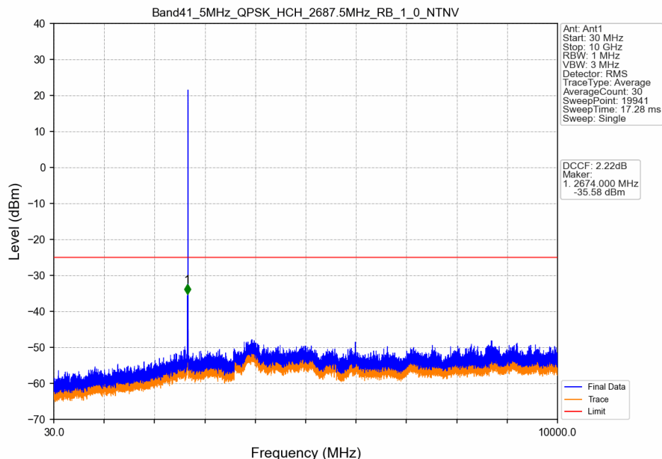
Band41_5MHz_QPSK_HCH_2687.5MHz_RB_1_0_NTNV
