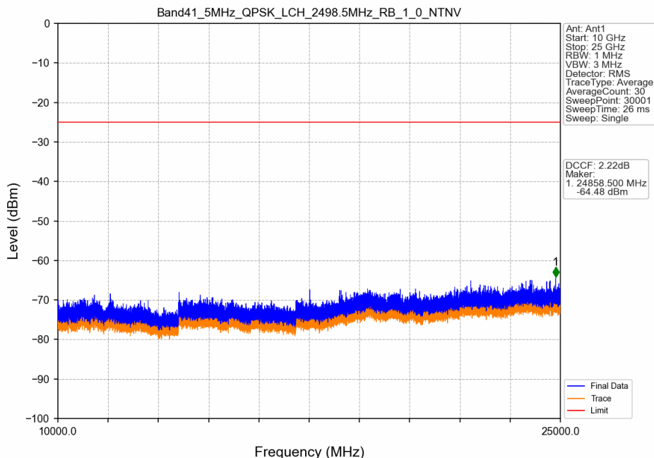
Band41_5MHz_QPSK_LCH_2498.5MHz_RB_1_0_NTNV
