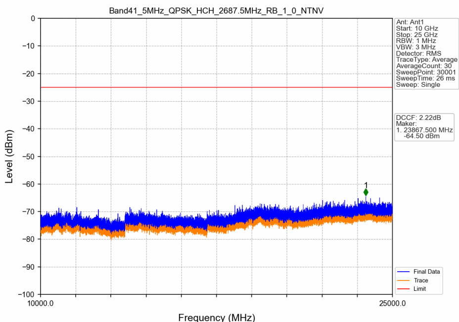
Band41_5MHz_QPSK_HCH_2687.5MHz_RB_1_0_NTNV
