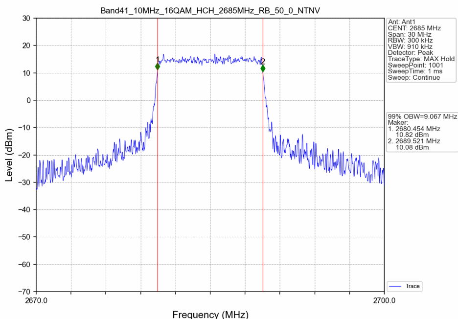
Band41_10MHz_16QAM_HCH_2685MHz_RB_50_0_NTNV
