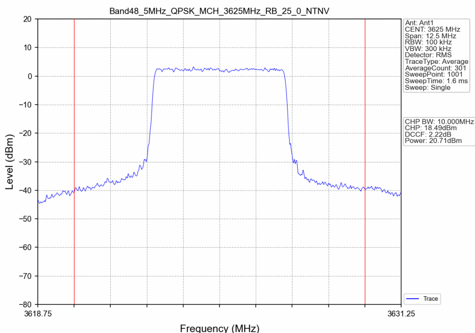
Band48_5MHz_QPSK_MCH_3625MHz_RB_25_0_NTNV
