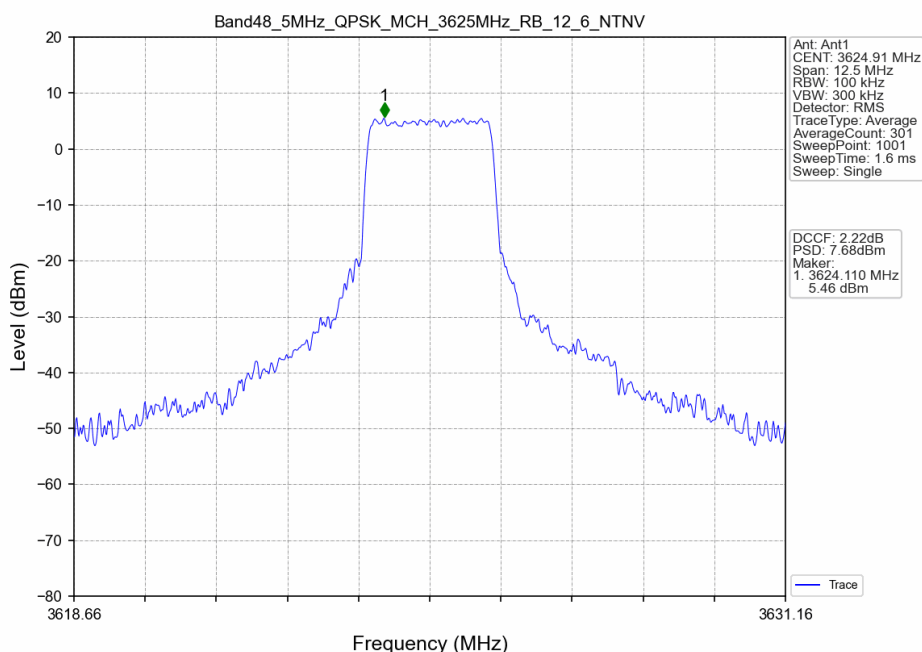
Band48_5MHz_QPSK_MCH_3625MHz_RB_12_6_NTNV
