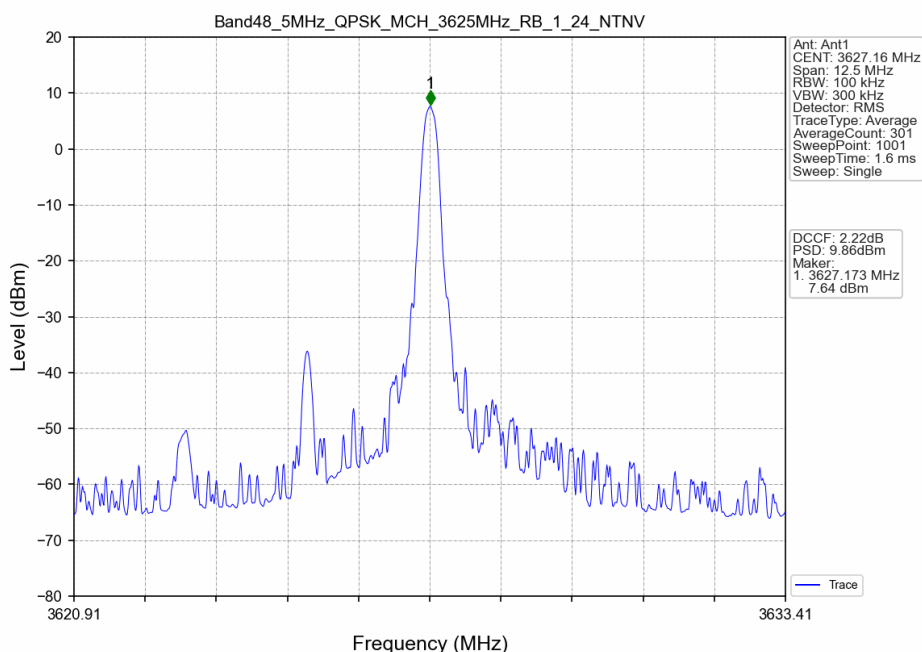
Band48_5MHz_QPSK_MCH_3625MHz_RB_1_24_NTNV
