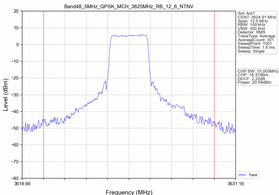
Band48_5MHz_QPSK_MCH_3625MHz_RB_12_6_NTNV
