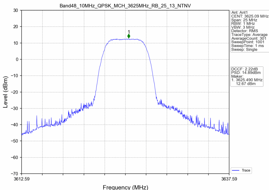
Band48_10MHz_QPSK_MCH_3625MHz_RB_25_13_NTNV
