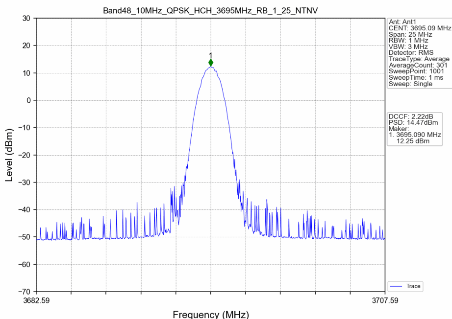
Band48_10MHz_QPSK_HCH_3695MHz_RB_1_25_NTNV
