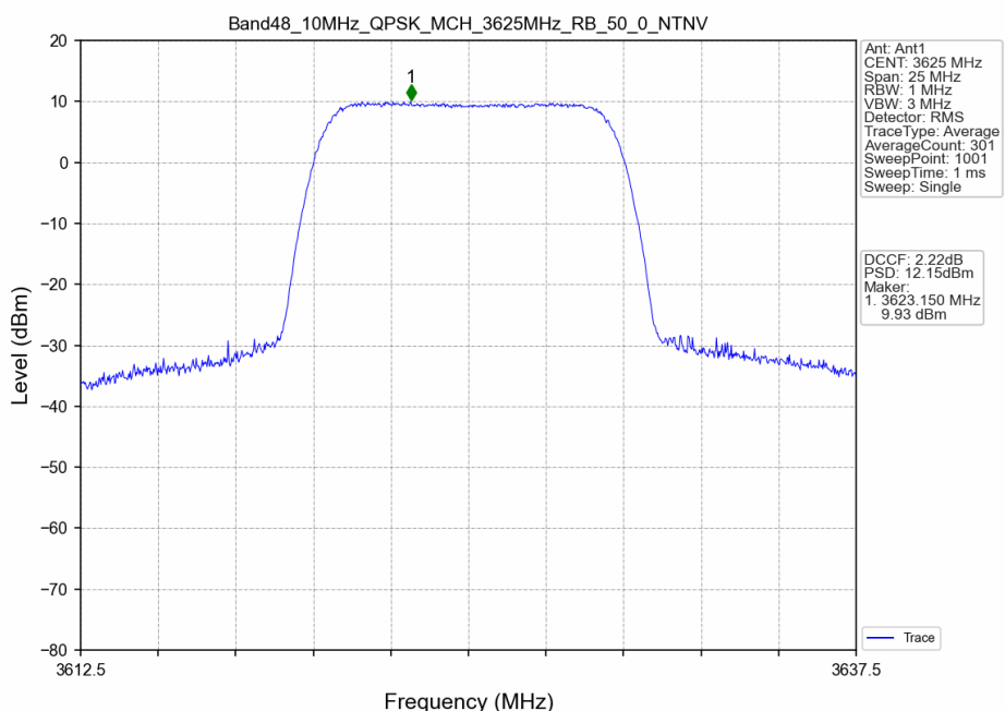
Band48_10MHz_QPSK_MCH_3625MHz_RB_50_0_NTNV
