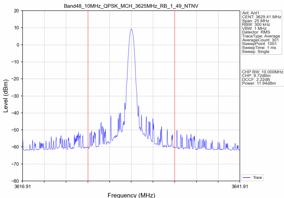
Band48_10MHz_QPSK_MCH_3625MHz_RB_1_49_NTNV
