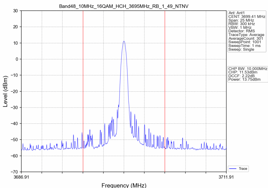
Band48_10MHz_16QAM_HCH_3695MHz_RB_1_49_NTNV
