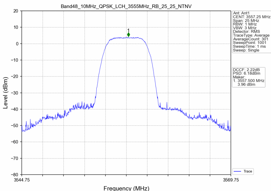
Band48_10MHz_QPSK_LCH_3555MHz_RB_25_25_NTNV
