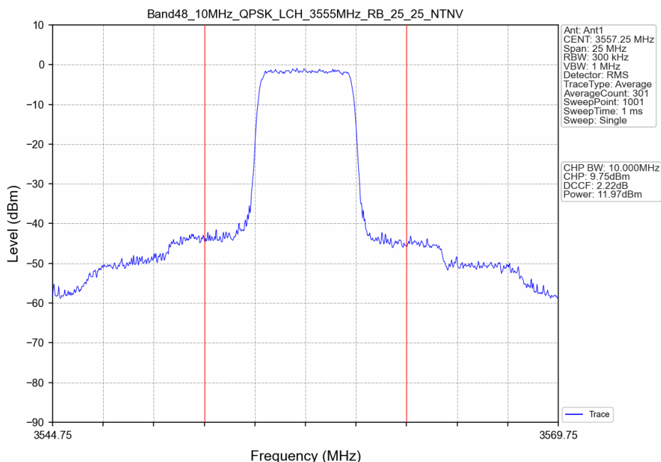
Band48_10MHz_QPSK_LCH_3555MHz_RB_25_25_NTNV
