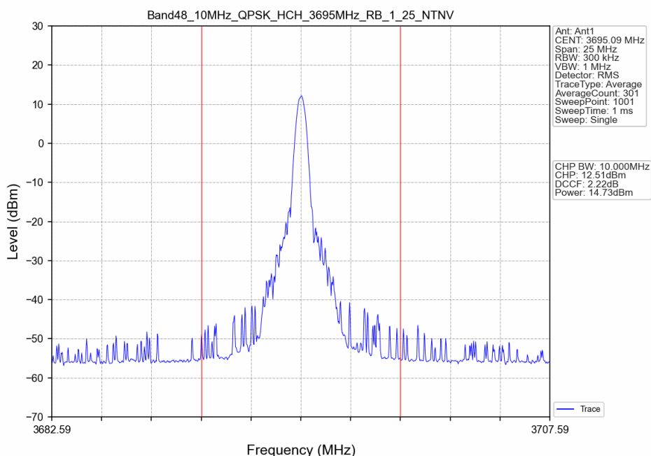
Band48_10MHz_QPSK_HCH_3695MHz_RB_1_25_NTNV
