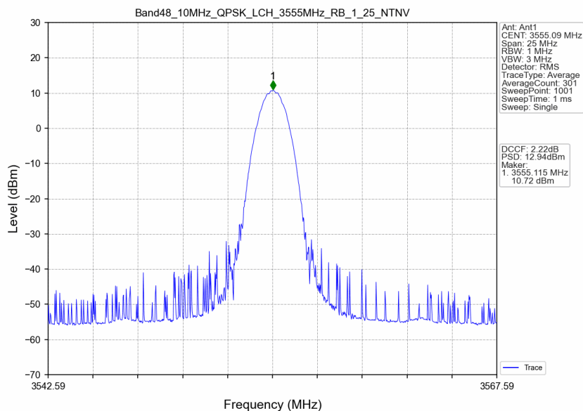
Band48_10MHz_QPSK_LCH_3555MHz_RB_1_25_NTNV
