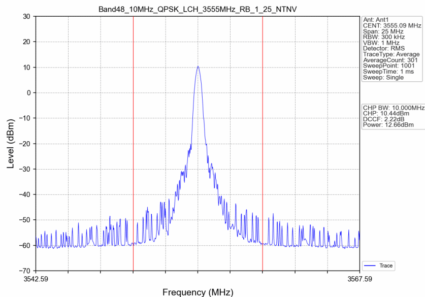
Band48_10MHz_QPSK_LCH_3555MHz_RB_1_25_NTNV
