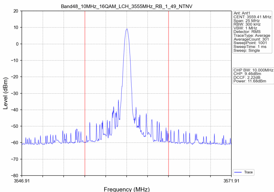
Band48_10MHz_16QAM_LCH_3555MHz_RB_1_49_NTNV
