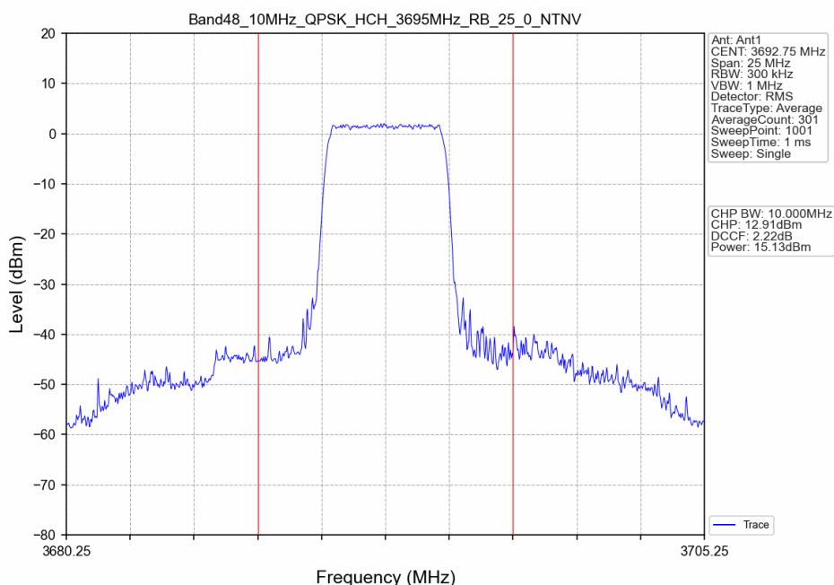
Band48_10MHz_QPSK_HCH_3695MHz_RB_25_0_NTNV
