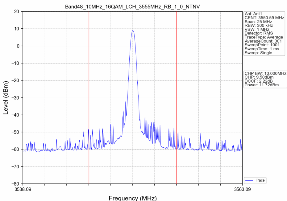
Band48_10MHz_16QAM_LCH_3555MHz_RB_1_0_NTNV
