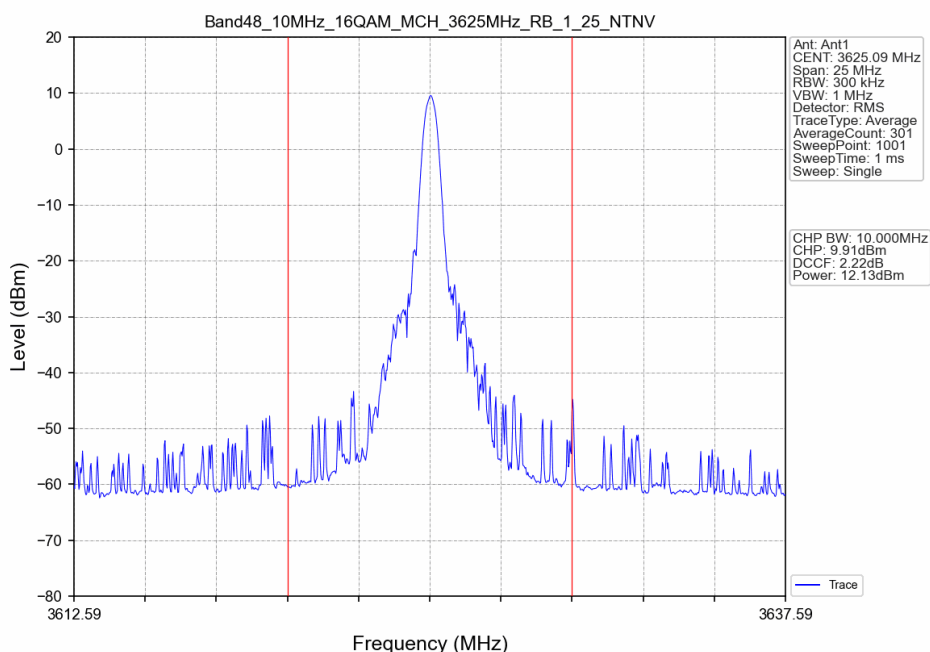
Band48_10MHz_16QAM_MCH_3625MHz_RB_1_25_NTNV
