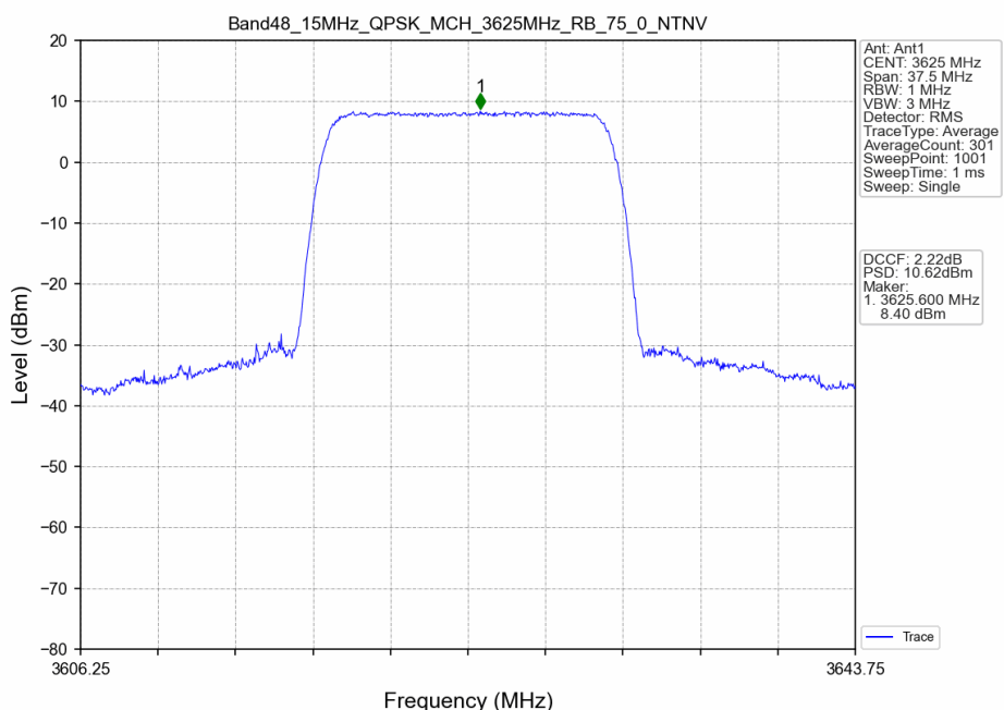
Band48_15MHz_QPSK_MCH_3625MHz_RB_75_0_NTNV
