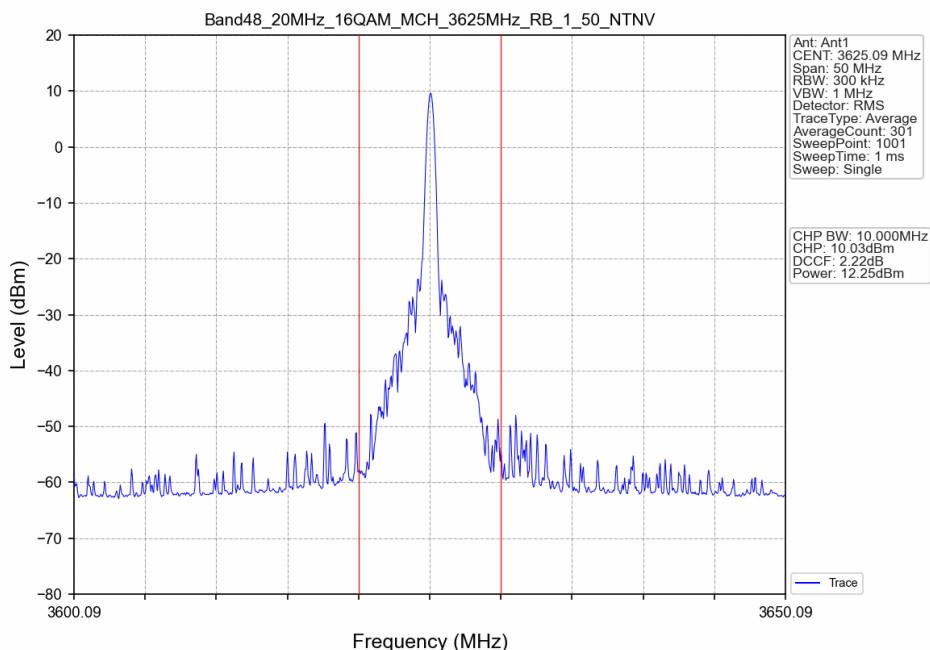
Band48_20MHz_16QAM_MCH_3625MHz_RB_1_50_NTNV
