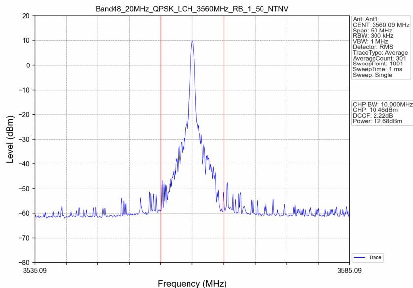
Band48_20MHz_QPSK_LCH_3560MHz_RB_1_50_NTNV
