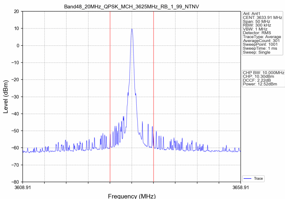
Band48_20MHz_QPSK_MCH_3625MHz_RB_1_99_NTNV
