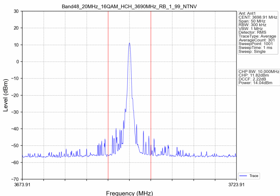
Band48_20MHz_16QAM_HCH_3690MHz_RB_1_99_NTNV
