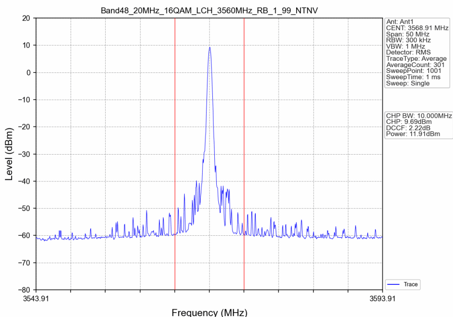
Band48_20MHz_16QAM_LCH_3560MHz_RB_1_99_NTNV
