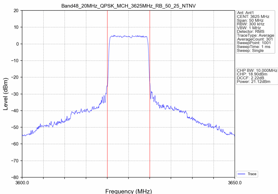
Band48_20MHz_QPSK_MCH_3625MHz_RB_50_25_NTNV
