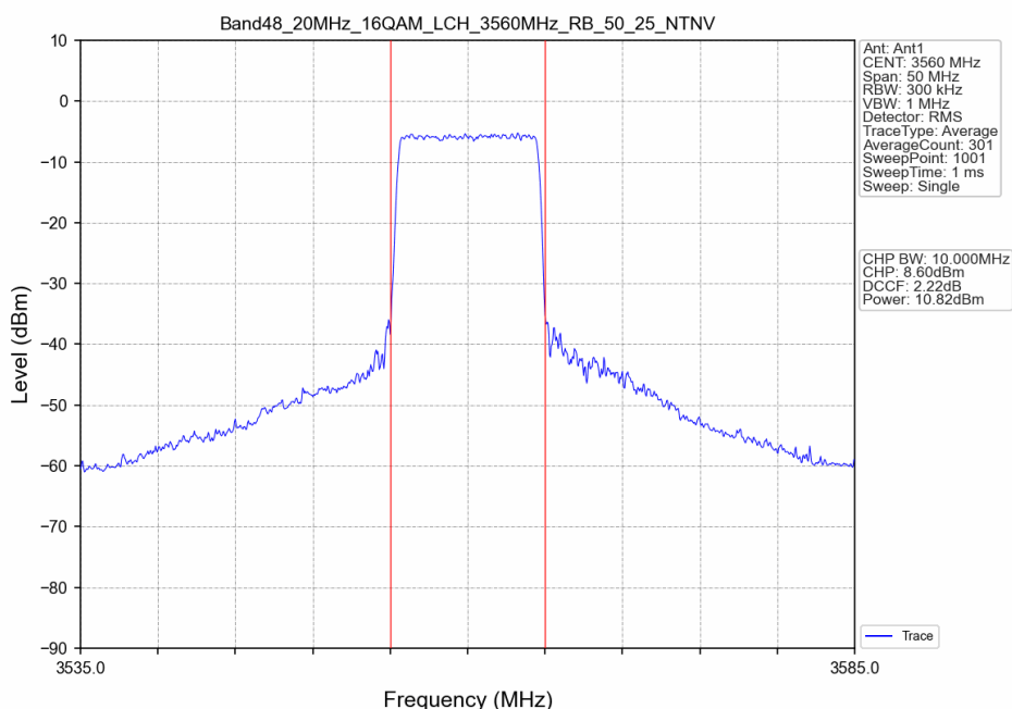
Band48_20MHz_16QAM_LCH_3560MHz_RB_50_25_NTNV
