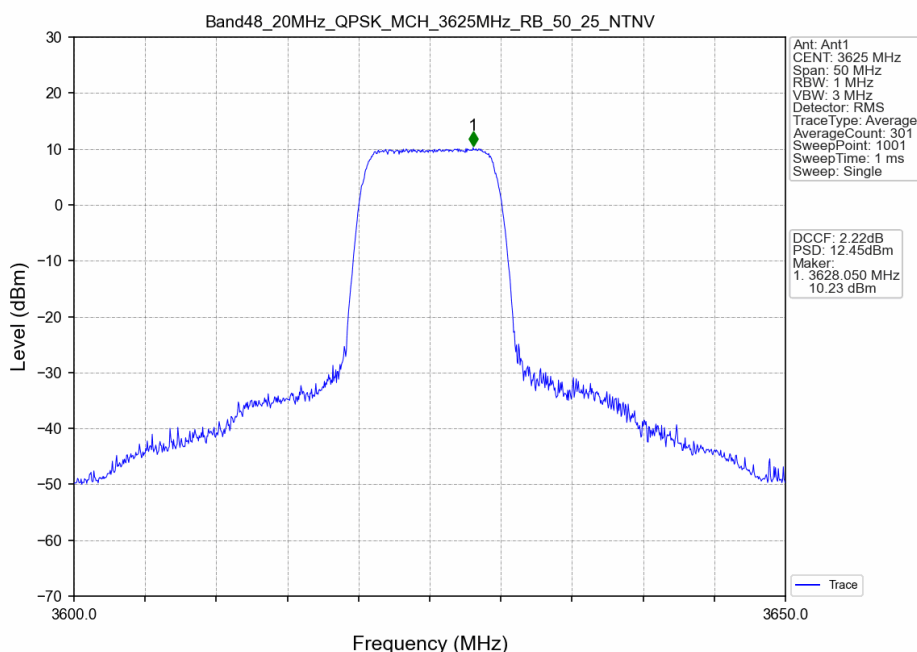
Band48_20MHz_QPSK_MCH_3625MHz_RB_50_25_NTNV
