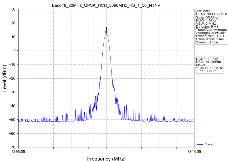
Band48_20MHz_QPSK_HCH_3690MHz_RB_1_50_NTNV
