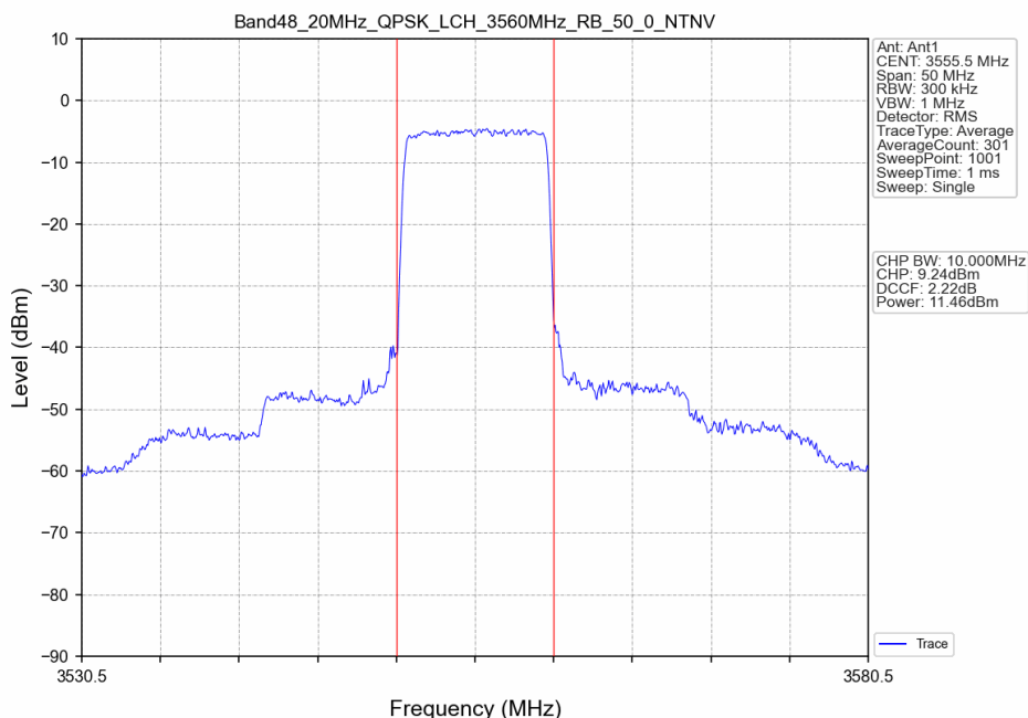
Band48_20MHz_QPSK_LCH_3560MHz_RB_50_0_NTNV
