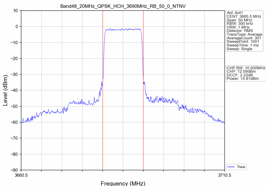
Band48_20MHz_QPSK_HCH_3690MHz_RB_50_0_NTNV
