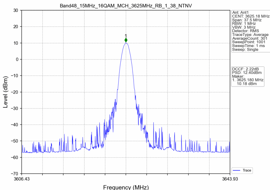
Band48_15MHz_16QAM_MCH_3625MHz_RB_1_38_NTNV
