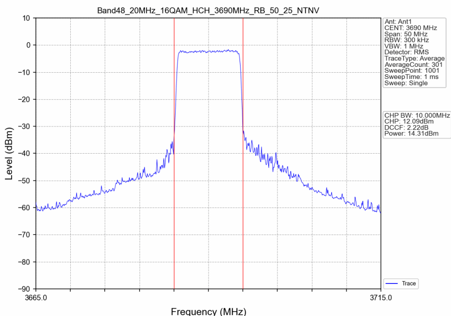
Band48_20MHz_16QAM_HCH_3690MHz_RB_50_25_NTNV
