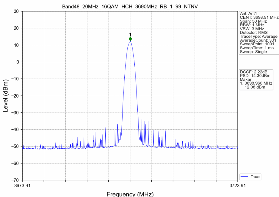
Band48_20MHz_16QAM_HCH_3690MHz_RB_1_99_NTNV
