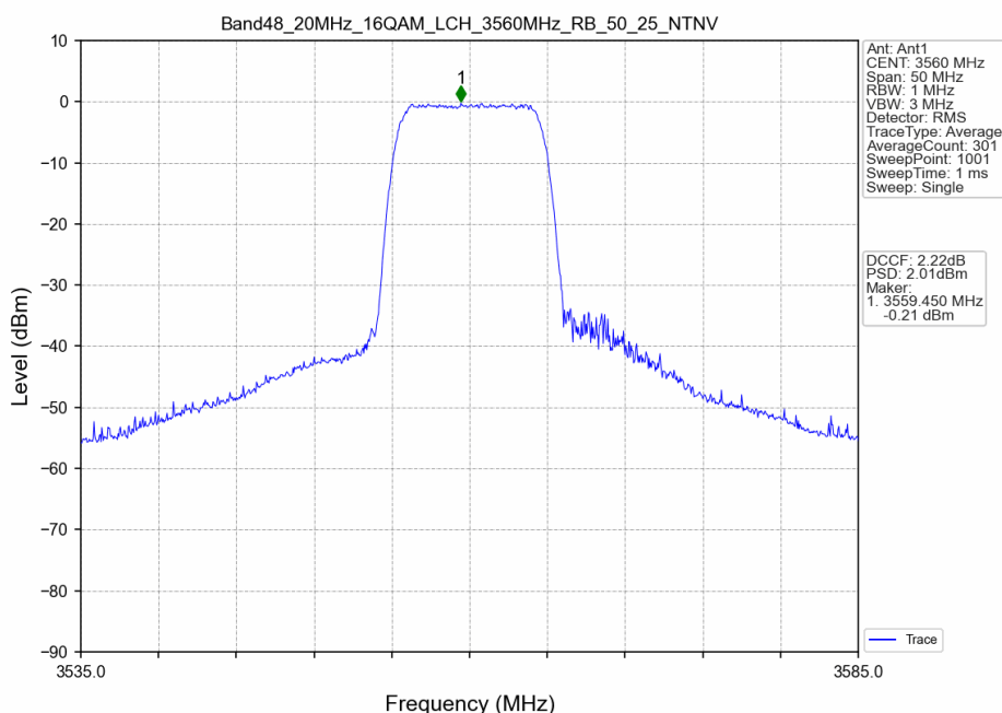
Band48_20MHz_16QAM_LCH_3560MHz_RB_50_25_NTNV
