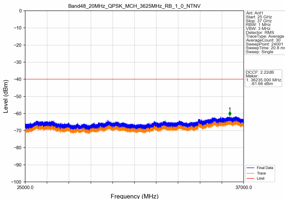
Band48_20MHz_QPSK_MCH_3625MHz_RB_1_0_NTNV
