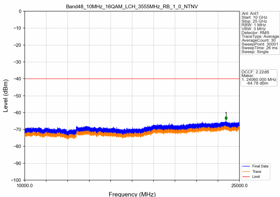
Band48_10MHz_16QAM_LCH_3555MHz_RB_1_0_NTNV
