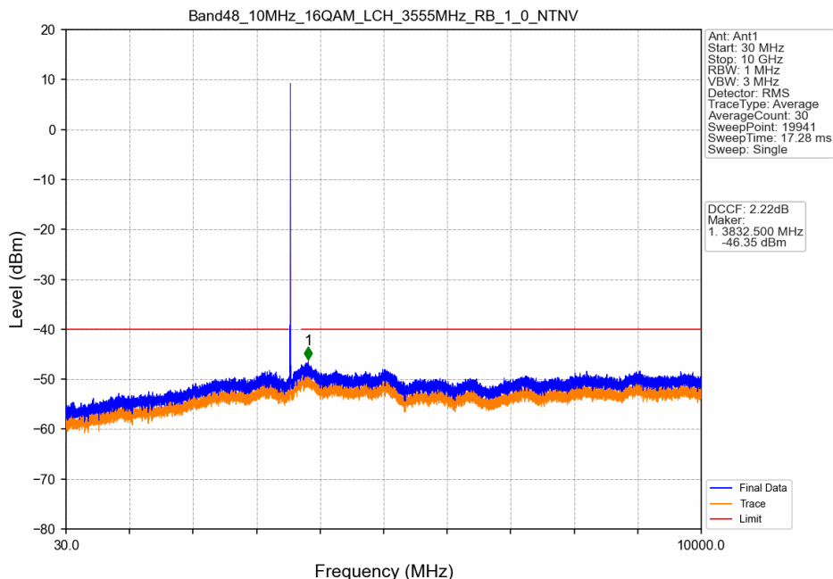
Band48_10MHz_16QAM_LCH_3555MHz_RB_1_0_NTNV
