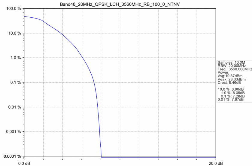
Band48_20MHz_QPSK_LCH_3560MHz_RB_100_0_NTNV
