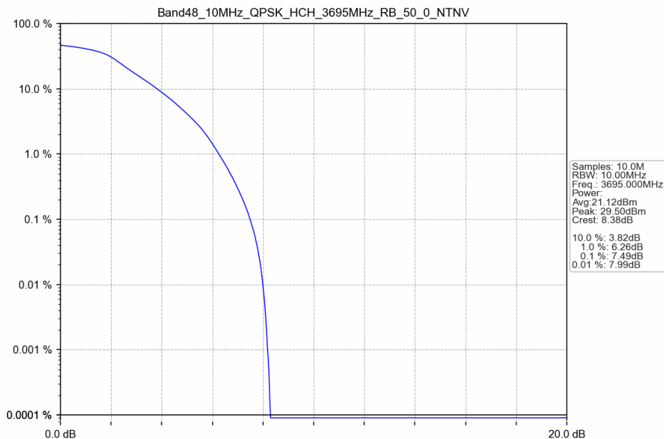
Band48_10MHz_QPSK_HCH_3695MHz_RB_50_0_NTNV
