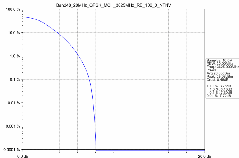
Band48_20MHz_QPSK_MCH_3625MHz_RB_100_0_NTNV
