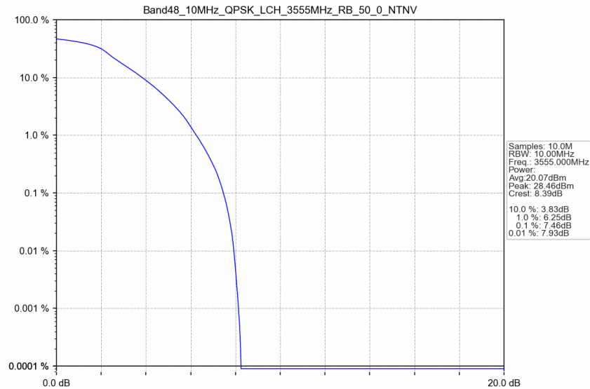
Band48_10MHz_QPSK_LCH_3555MHz_RB_50_0_NTNV
