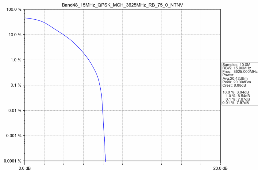
Band48_15MHz_QPSK_MCH_3625MHz_RB_75_0_NTNV
