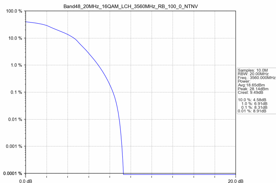
Band48_20MHz_16QAM_LCH_3560MHz_RB_100_0_NTNV
