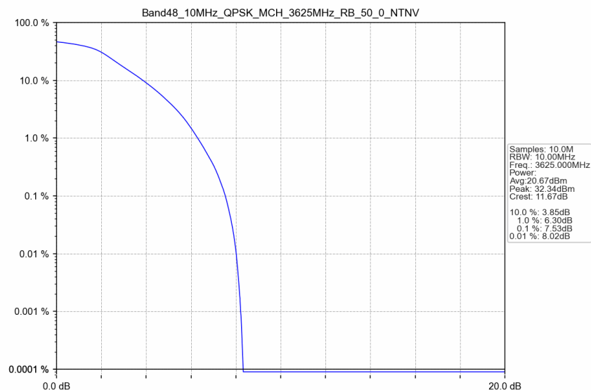
Band48_10MHz_QPSK_MCH_3625MHz_RB_50_0_NTNV
