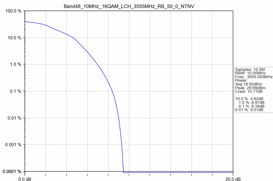
Band48_10MHz_16QAM_LCH_3555MHz_RB_50_0_NTNV
