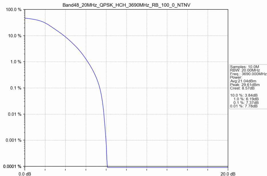
Band48_20MHz_QPSK_HCH_3690MHz_RB_100_0_NTNV
