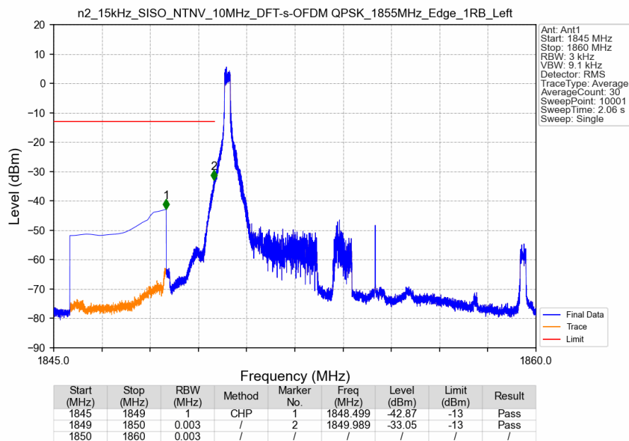
n2_15kHz_SISO_NTNV_10MHz_DFT-s-OFDM QPSK_1855MHz_Edge_1RB_Left
