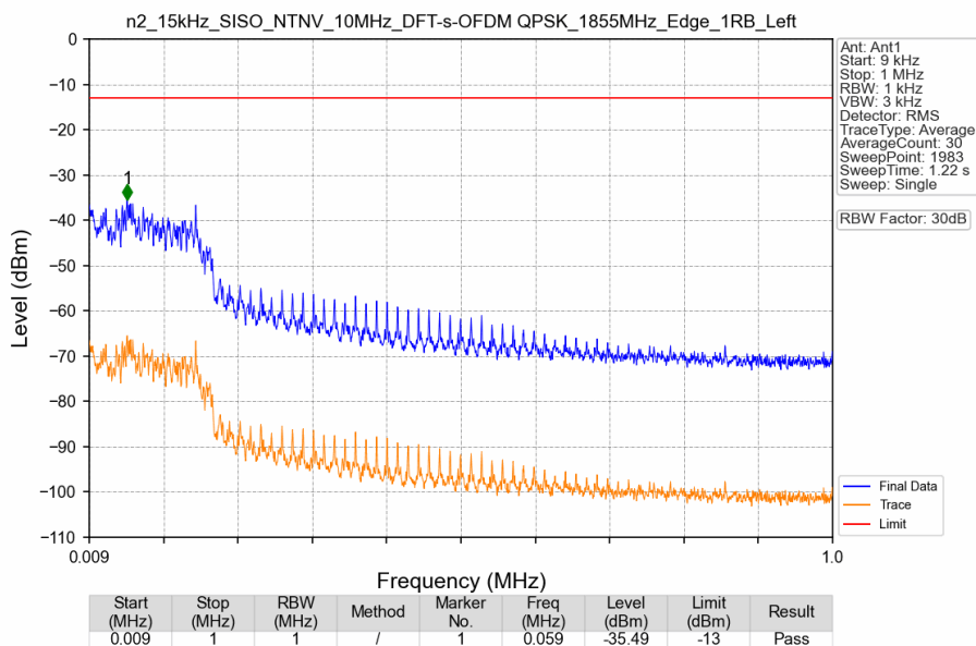
n2_15kHz_SISO_NTNV_10MHz_DFT-s-OFDM QPSK_1855MHz_Edge_1RB_Left
