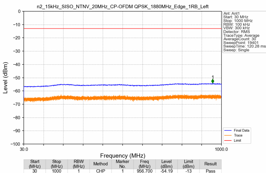
n2_15kHz_SISO_NTNV_20MHz_CP-OFDM QPSK_1880MHz_Edge_1RB_Left
