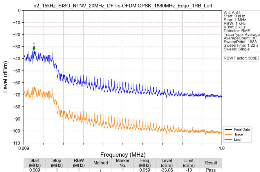
n2_15kHz_SISO_NTNV_20MHz_DFT-s-OFDM QPSK_1880MHz_Edge_1RB_Left
