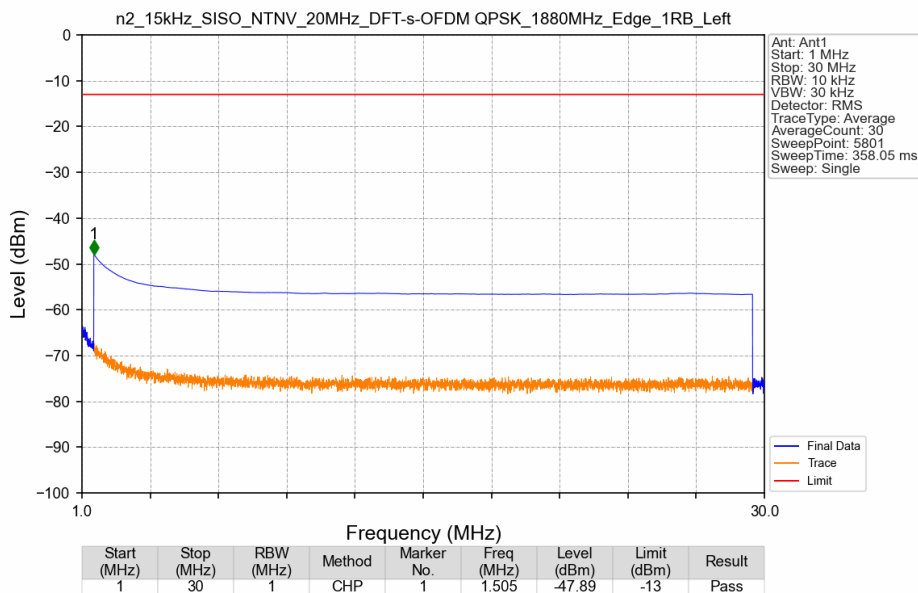
n2_15kHz_SISO_NTNV_20MHz_DFT-s-OFDM QPSK_1880MHz_Edge_1RB_Left
