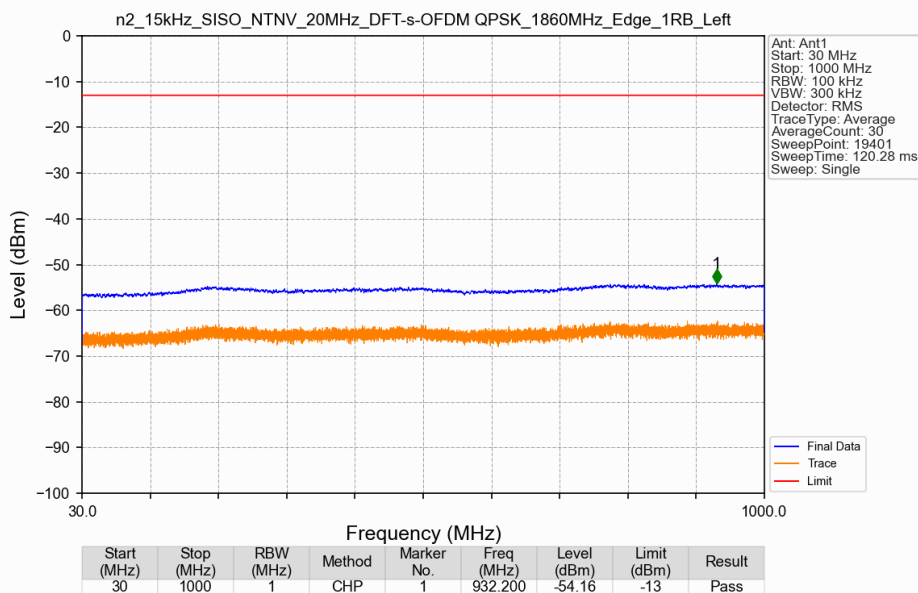
n2_15kHz_SISO_NTNV_20MHz_DFT-s-OFDM QPSK_1860MHz_Edge_1RB_Left
