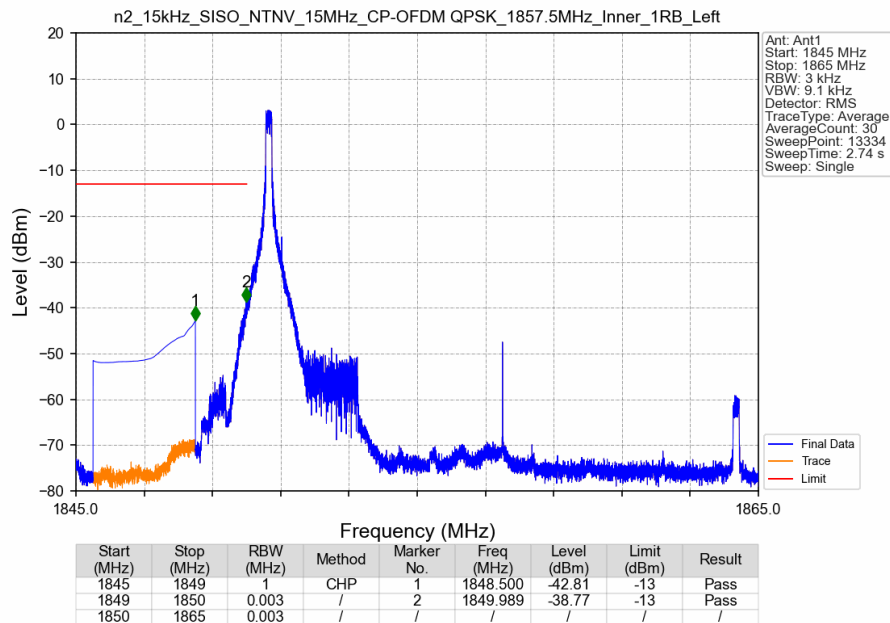
n2_15kHz_SISO_NTNV_15MHz_CP-OFDM QPSK_1857.5MHz_Inner_1RB_Left
