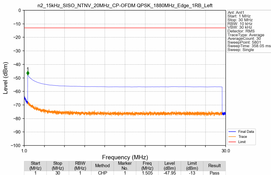
n2_15kHz_SISO_NTNV_20MHz_CP-OFDM QPSK_1880MHz_Edge_1RB_Left
