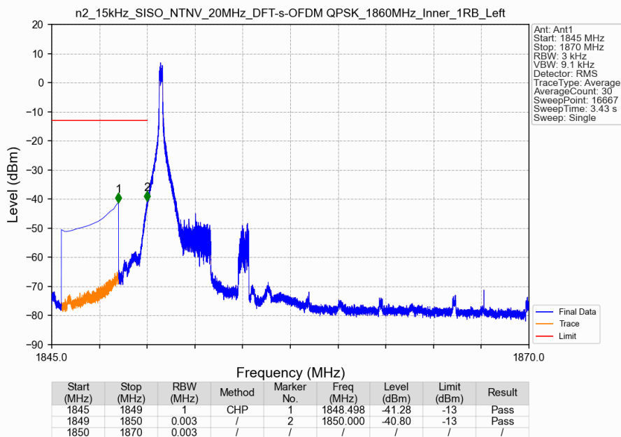
n2_15kHz_SISO_NTNV_20MHz_DFT-s-OFDM QPSK_1860MHz_Inner_1RB_Left
