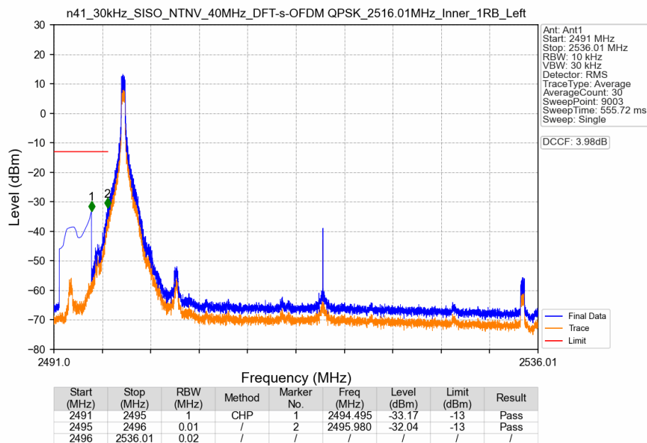
n41_30kHz_SISO_NTNV_40MHz_DFT-s-OFDM QPSK_2516.01MHz_Inner_1RB_Left
