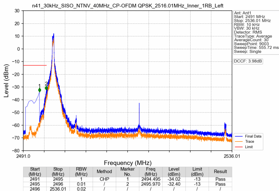
n41_30kHz_SISO_NTNV_40MHz_CP-OFDM QPSK_2516.01MHz_Inner_1RB_Left
