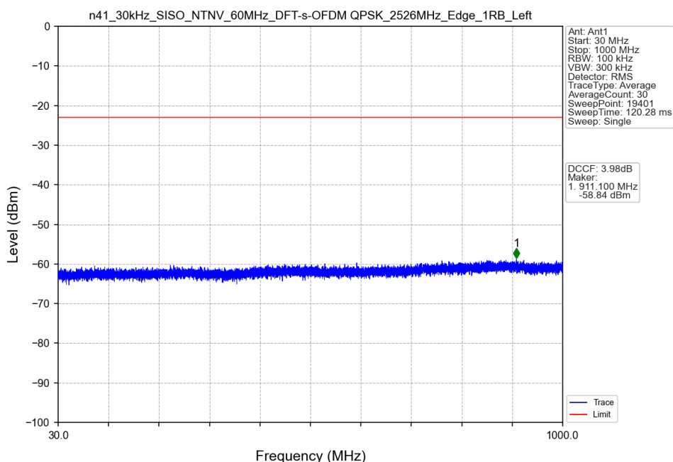
n41_30kHz_SISO_NTNV_60MHz_DFT-s-OFDM QPSK_2526MHz_Edge_1RB_Left
