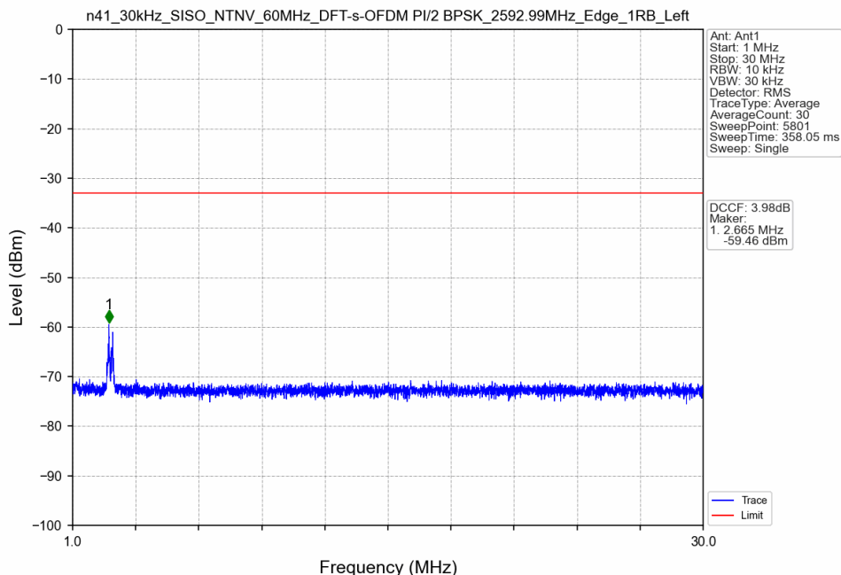
n41_30kHz_SISO_NTNV_60MHz_DFT-s-OFDM PI/2 BPSK_2592.99MHz_Edge_1RB_Left
