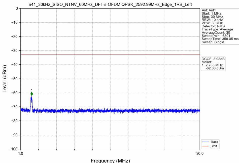
n41_30kHz_SISO_NTNV_60MHz_DFT-s-OFDM QPSK_2592.99MHz_Edge_1RB_Left
