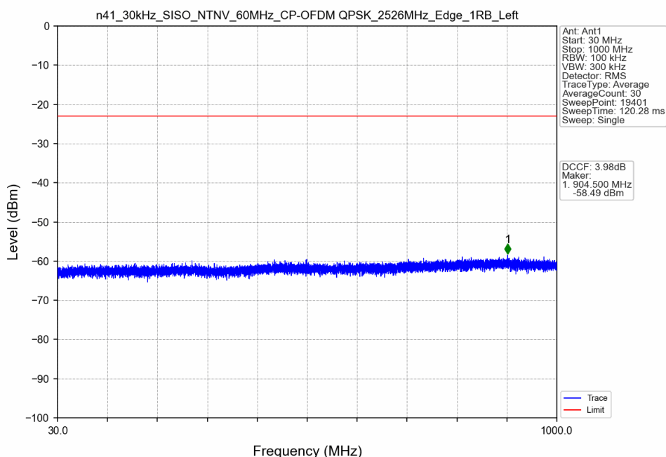
n41_30kHz_SISO_NTNV_60MHz_CP-OFDM QPSK_2526MHz_Edge_1RB_Left
