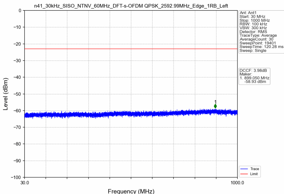
n41_30kHz_SISO_NTNV_60MHz_DFT-s-OFDM QPSK_2592.99MHz_Edge_1RB_Left
