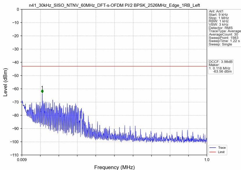
n41_30kHz_SISO_NTNV_60MHz_DFT-s-OFDM PI/2 BPSK_2526MHz_Edge_1RB_Left
