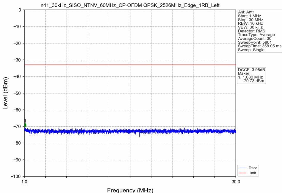
n41_30kHz_SISO_NTNV_60MHz_CP-OFDM QPSK_2526MHz_Edge_1RB_Left
