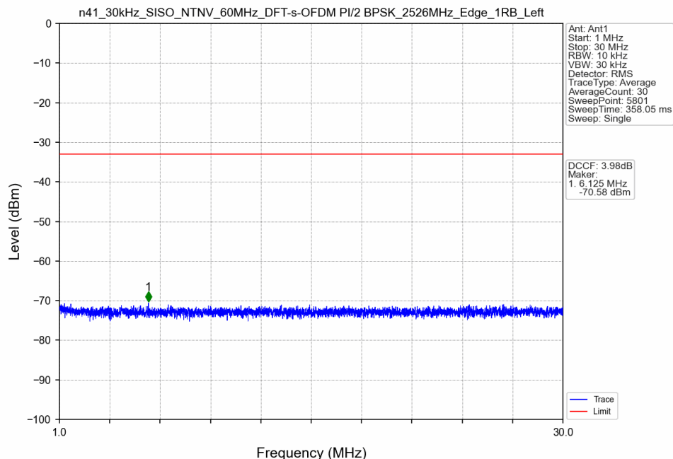
n41_30kHz_SISO_NTNV_60MHz_DFT-s-OFDM PI/2 BPSK_2526MHz_Edge_1RB_Left
