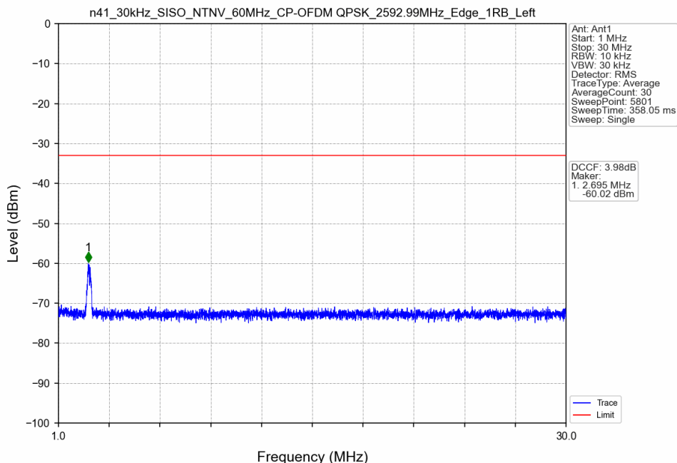
n41_30kHz_SISO_NTNV_60MHz_CP-OFDM QPSK_2592.99MHz_Edge_1RB_Left
