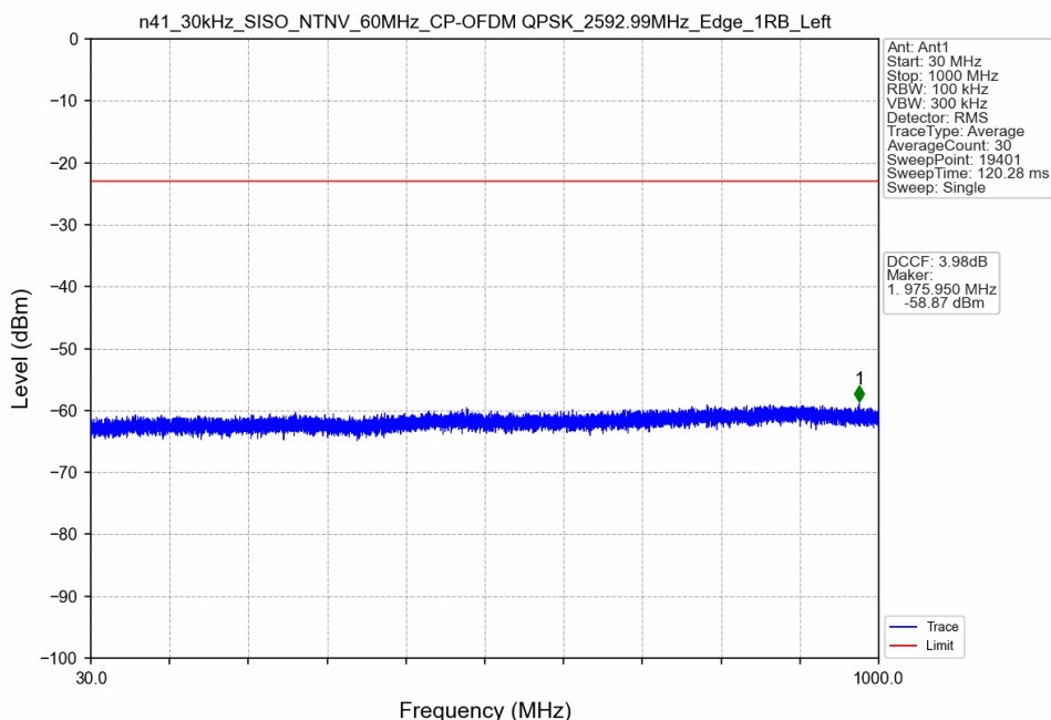
n41_30kHz_SISO_NTNV_60MHz_CP-OFDM QPSK_2592.99MHz_Edge_1RB_Left
