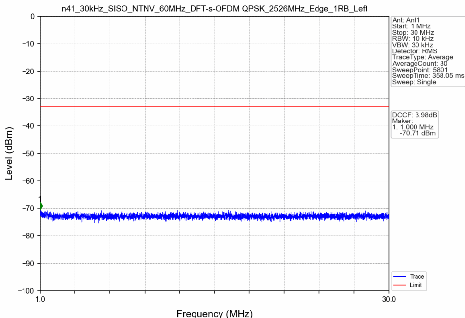
n41_30kHz_SISO_NTNV_60MHz_DFT-s-OFDM QPSK_2526MHz_Edge_1RB_Left
