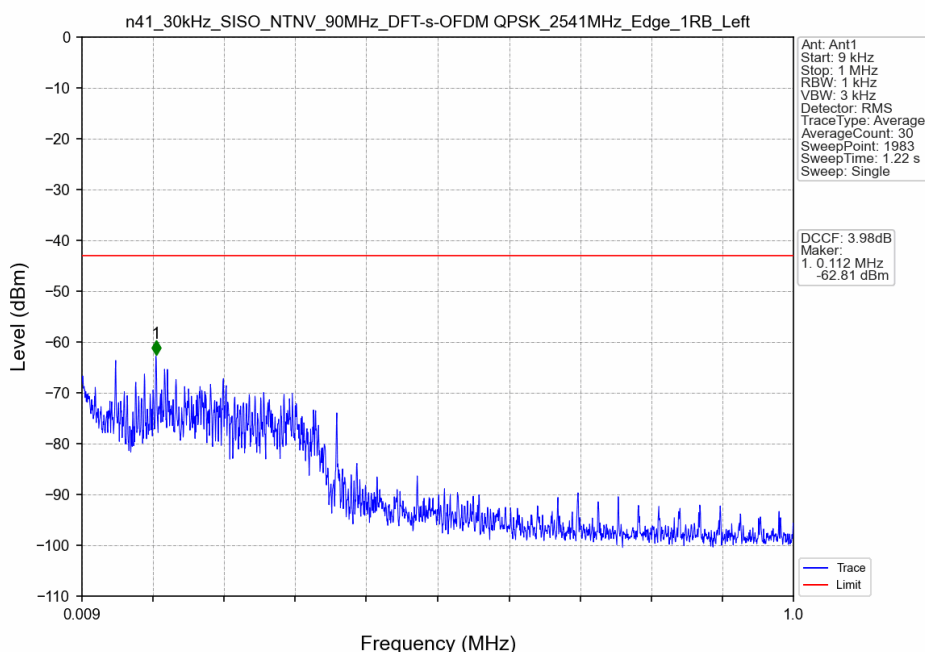
n41_30kHz_SISO_NTNV_90MHz_DFT-s-OFDM QPSK_2541MHz_Edge_1RB_Left
