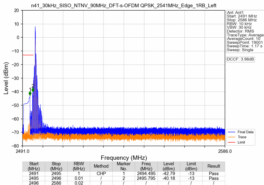
n41_30kHz_SISO_NTNV_90MHz_DFT-s-OFDM QPSK_2541MHz_Edge_1RB_Left
