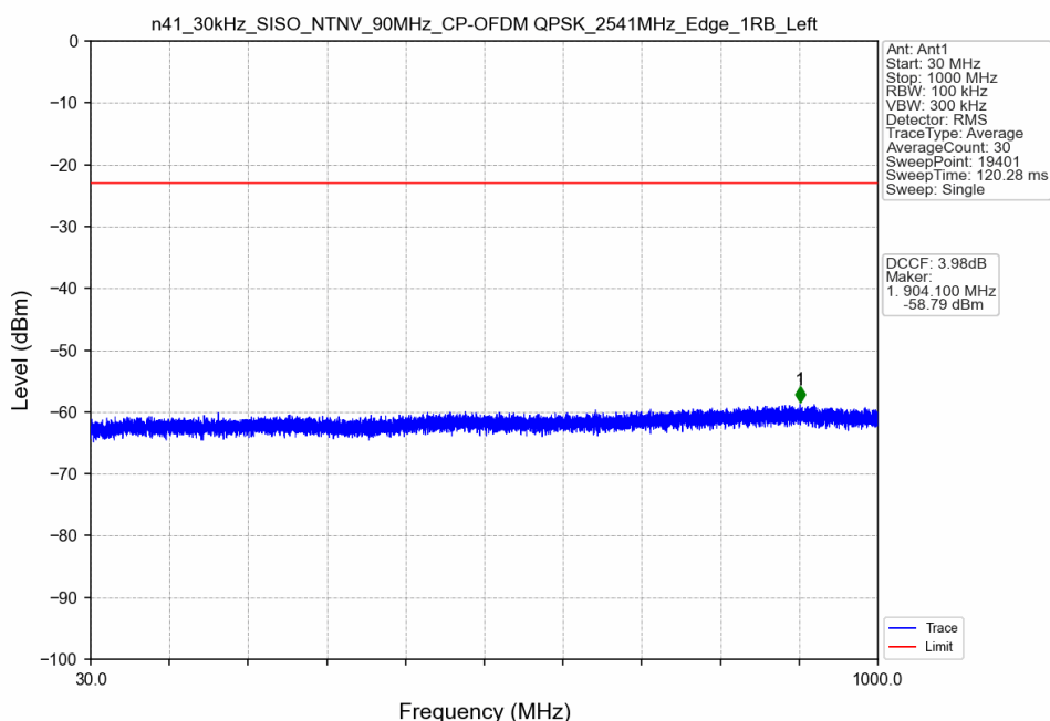
n41_30kHz_SISO_NTNV_90MHz_CP-OFDM QPSK_2541MHz_Edge_1RB_Left
