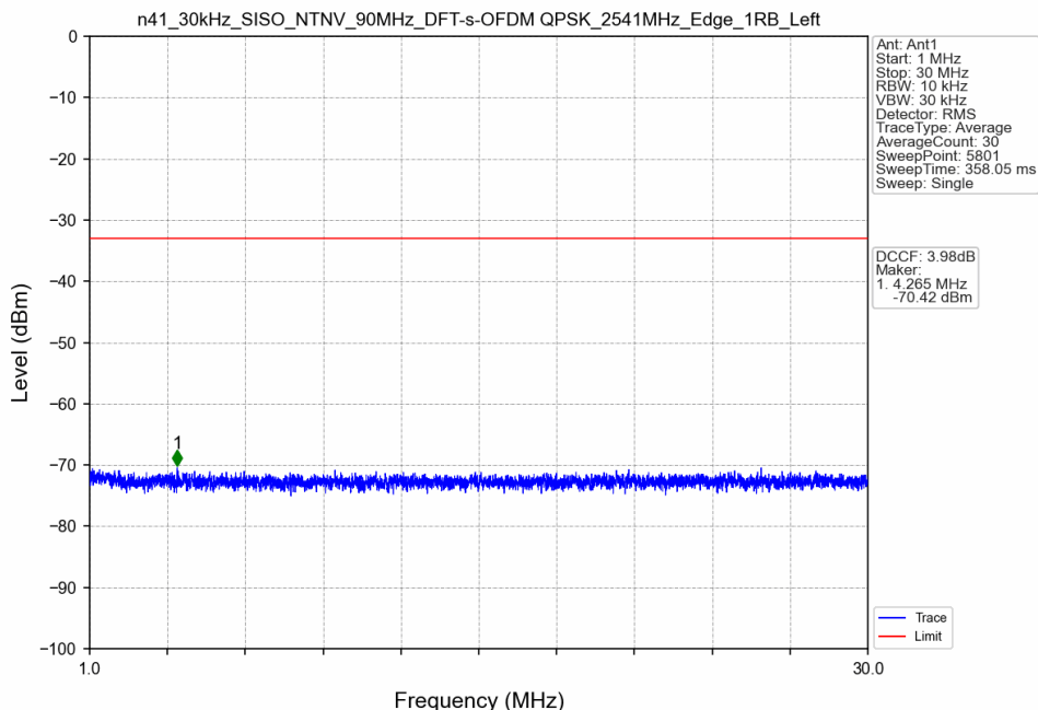
n41_30kHz_SISO_NTNV_90MHz_DFT-s-OFDM QPSK_2541MHz_Edge_1RB_Left
