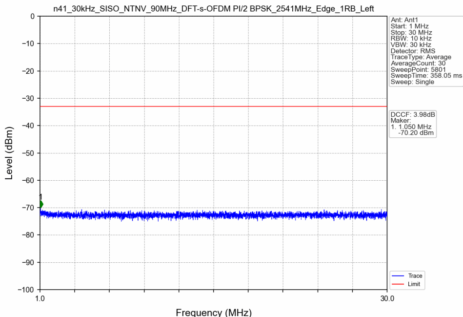
n41_30kHz_SISO_NTNV_90MHz_DFT-s-OFDM PI/2 BPSK_2541MHz_Edge_1RB_Left
