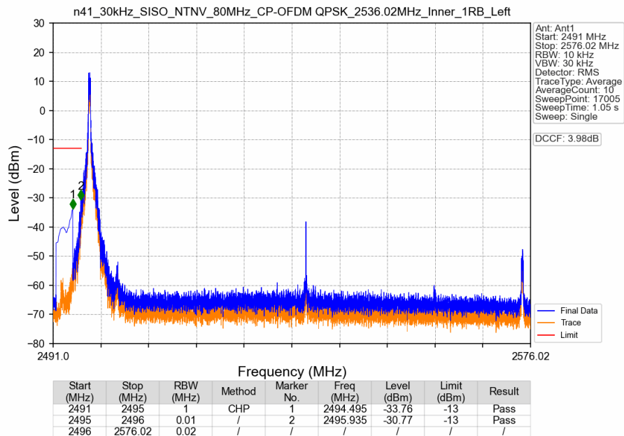
n41_30kHz_SISO_NTNV_80MHz_CP-OFDM QPSK_2536.02MHz_Inner_1RB_Left
