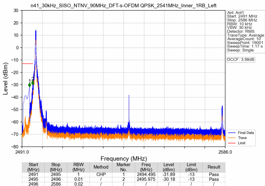
n41_30kHz_SISO_NTNV_90MHz_DFT-s-OFDM QPSK_2541MHz_Inner_1RB_Left
