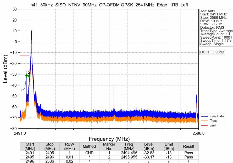
n41_30kHz_SISO_NTNV_90MHz_CP-OFDM QPSK_2541MHz_Edge_1RB_Left
