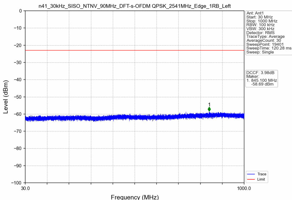
n41_30kHz_SISO_NTNV_90MHz_DFT-s-OFDM QPSK_2541MHz_Edge_1RB_Left
