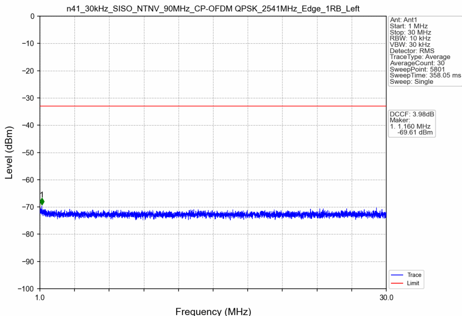
n41_30kHz_SISO_NTNV_90MHz_CP-OFDM QPSK_2541MHz_Edge_1RB_Left
