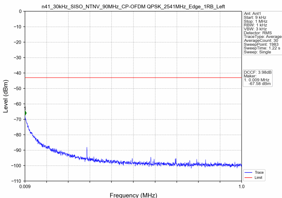
n41_30kHz_SISO_NTNV_90MHz_CP-OFDM QPSK_2541MHz_Edge_1RB_Left
