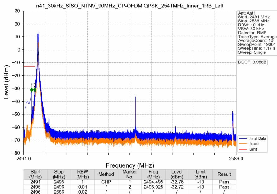
n41_30kHz_SISO_NTNV_90MHz_CP-OFDM QPSK_2541MHz_Inner_1RB_Left
