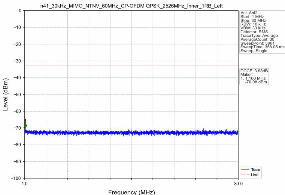
n41_30kHz_MIMO_NTNV_60MHz_CP-OFDM QPSK_2526MHz_Inner_1RB_Left
