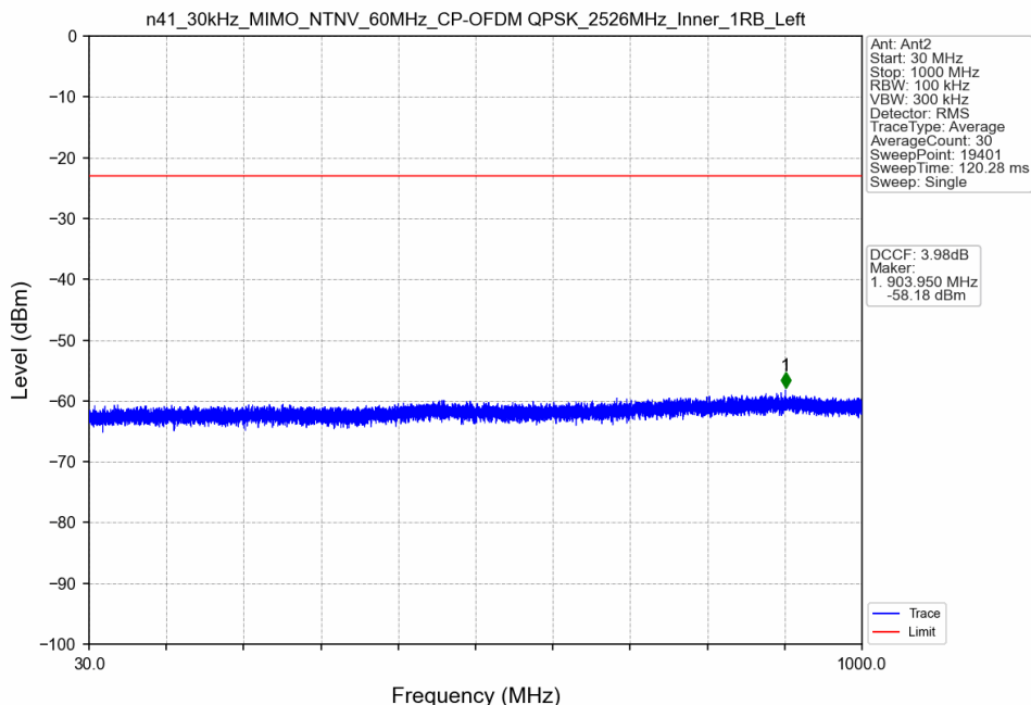
n41_30kHz_MIMO_NTNV_60MHz_CP-OFDM QPSK_2526MHz_Inner_1RB_Left
