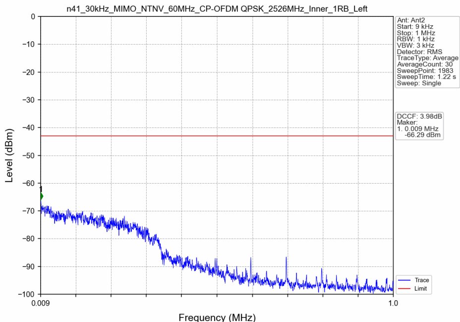
n41_30kHz_MIMO_NTNV_60MHz_CP-OFDM QPSK_2526MHz_Inner_1RB_Left
