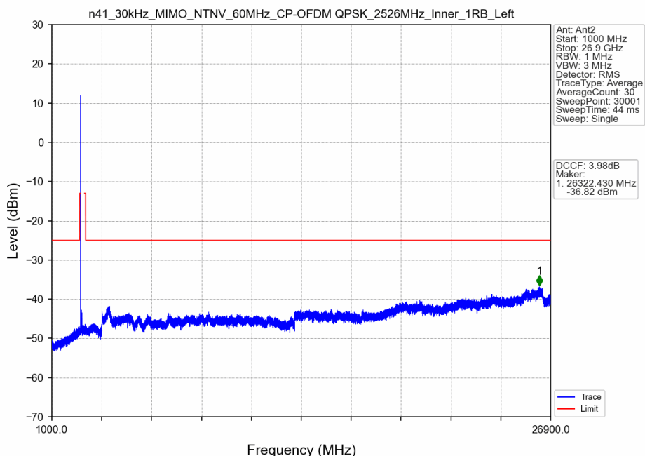
n41_30kHz_MIMO_NTNV_60MHz_CP-OFDM QPSK_2526MHz_Inner_1RB_Left
