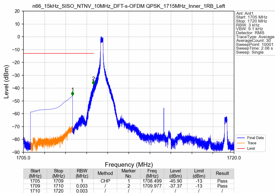
n66_15kHz_SISO_NTNV_10MHz_DFT-s-OFDM QPSK_1715MHz_Inner_1RB_Left
