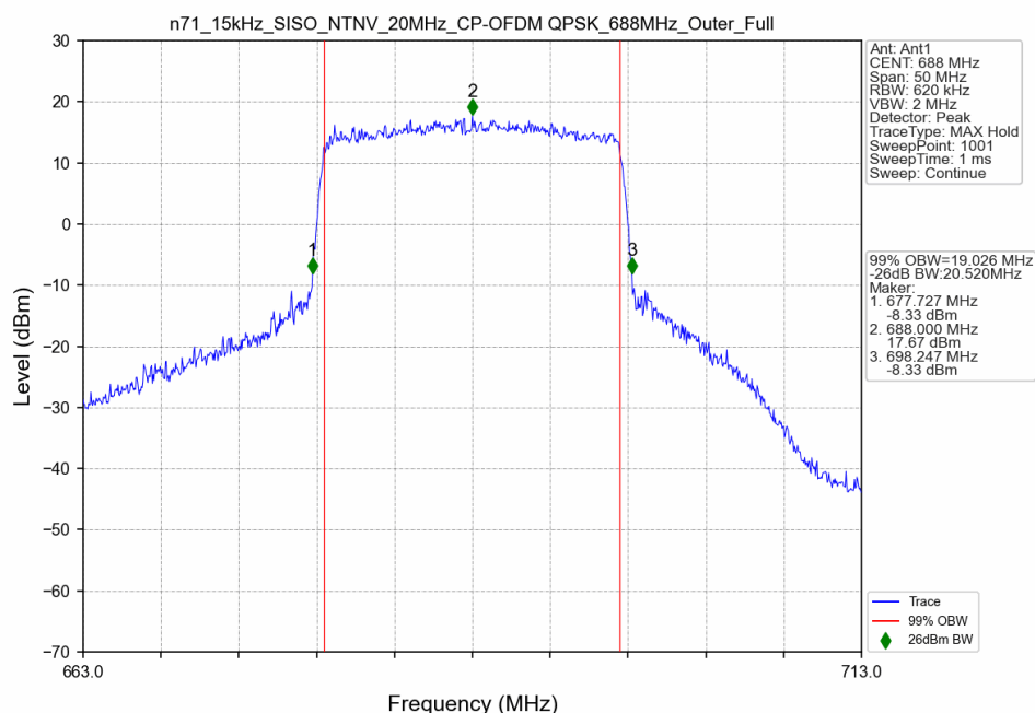
n71_15kHz_SISO_NTNV_20MHz_CP-OFDM QPSK_688MHz_Outer_Full
