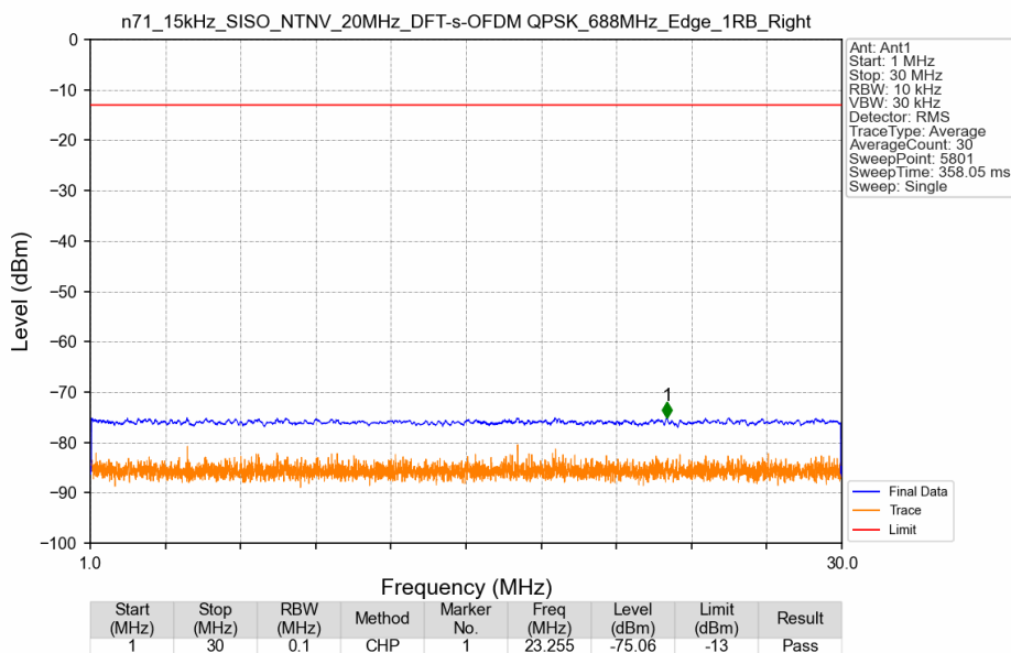
n71_15kHz_SISO_NTNV_20MHz_DFT-s-OFDM QPSK_688MHz_Edge_1RB_Right
