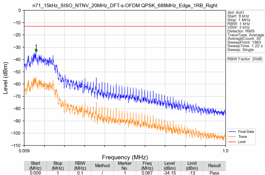
n71_15kHz_SISO_NTNV_20MHz_DFT-s-OFDM QPSK_688MHz_Edge_1RB_Right
