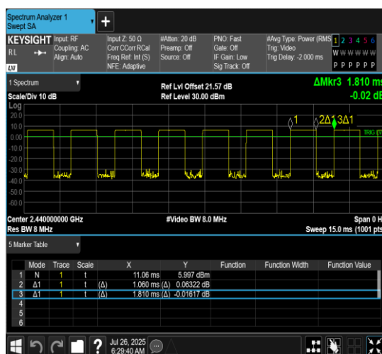
NTNV-BLE_500K-Ant7-2440
