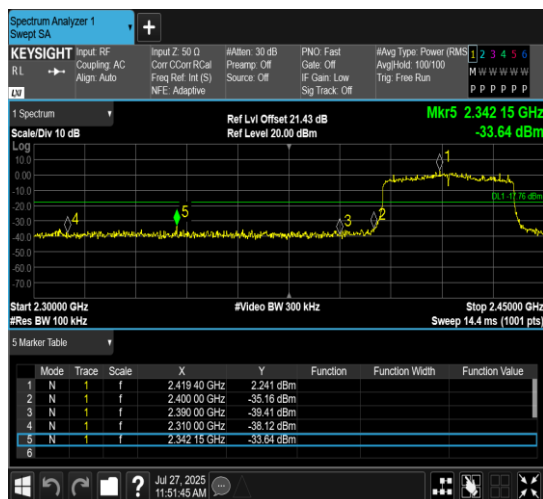
11AX40MIMO-Ant10-2452-PASS
