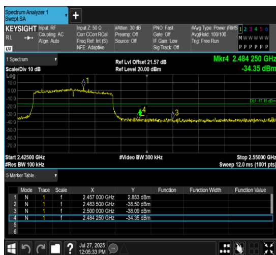
11AX40MIMO-Ant10-2452-PASS
