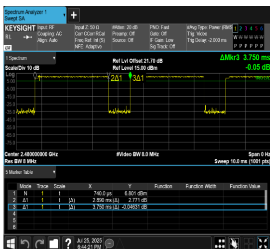
NTNV-3DH5-Ant10-2480
