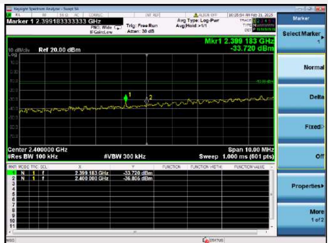
802.11n-20 MHz CH3, BAND EDGE
