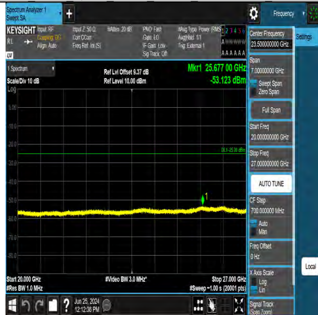
Band41 5MHz QPSK 40620 1RB#0 20000~27000 20000~27000
