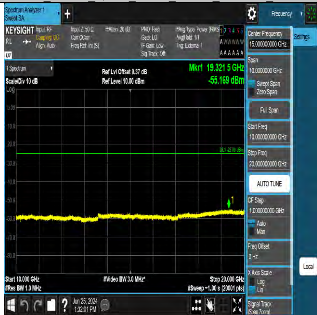
Band41 20MHz QPSK 41490 1RB#0 10000~20000 10000~20000
