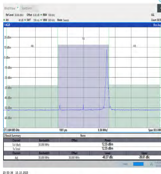
NTVN_N48_PC3_30_30_H_TID18_#1_-30_30
