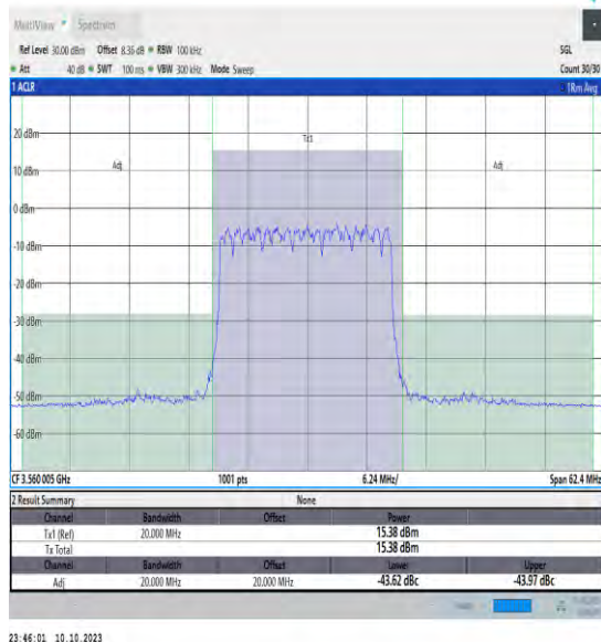
NTVN_N48_PC3_30_20_L_TID1_#1_-20_20
