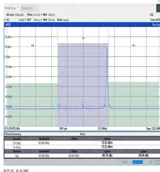
NTNV_N48_PC3_30_40_H_TID18_#1_-40_40
