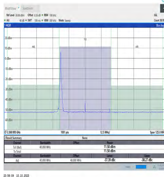
NTVN_N48_PC3_30_40_L_TID17_#1_-40_40
