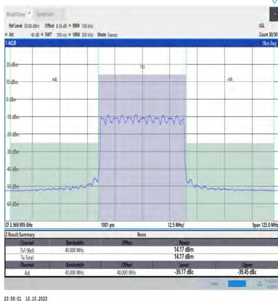
NTVN_N48_PC3_30_40_L_TID16_#1_-40_40
