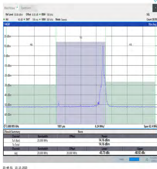
NTVN_N48_PC3_30_20_H_TID18_#1_-20_20
