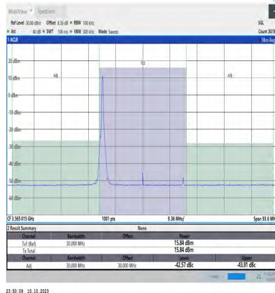
NTVN_N48_PC3_30_30_L_TID2_#1_-30_30
