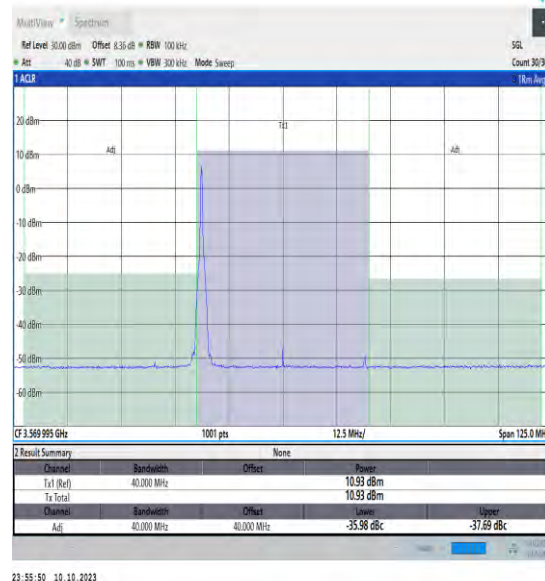
NTVN_N48_PC3_30_40_L_TID2_#1_-40_40
