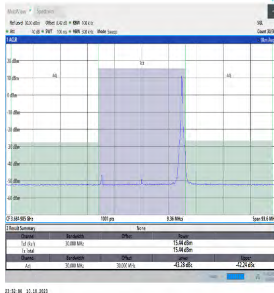
NTVN_N48_PC3_30_30_H_TID3_#1_-30_30
