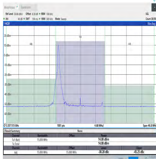
NTVN_N48_PC3_30_15_L_TID17_#1_-15_15
