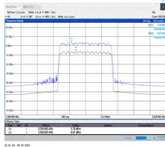
1-N48-PC3-30-40-L-2-CP-256QAM-Outer_Full-106@ 0-Ant7-9.45-100%-0.00-9.45-PASS-≤13
