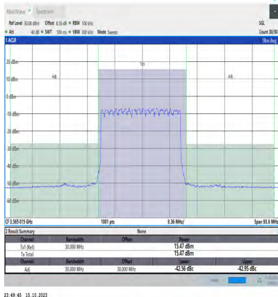
NTVN_N48_PC3_30_30_L_TID1_#1_-30_30
