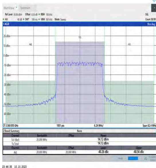
NTVN_N48_PC3_30_20_L_TID16_#1_-20_20
