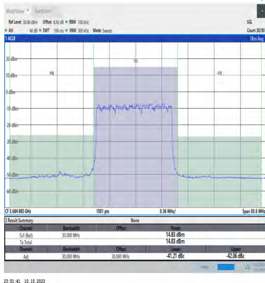
NTVN_N48_PC3_30_30_H_TID1_#1_-30_30
