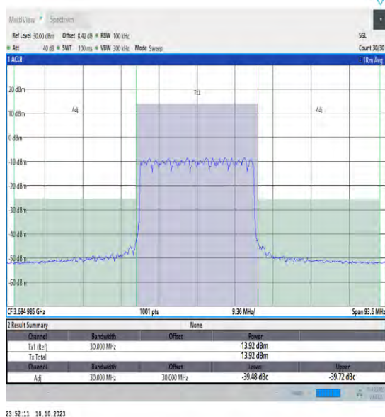
NTVN_N48_PC3_30_30_H_TID16_#1_-30_30
