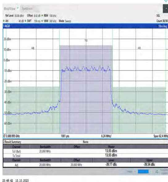
NTVN_N48_PC3_30_20_H_TID16_#1_-20_20
