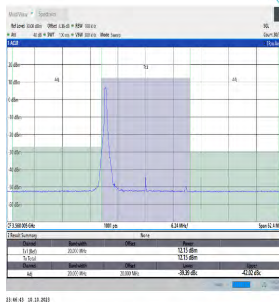
NTVN_N48_PC3_30_20_L_TID17_#1_-20_20
