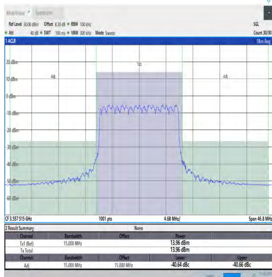
NTVN_N48_PC3_30_15_L_TID16_#1_-15_15
