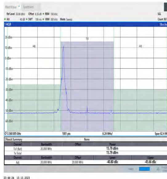
NTVN_N48_PC3_30_20_L_TID2_#1_-20_20
