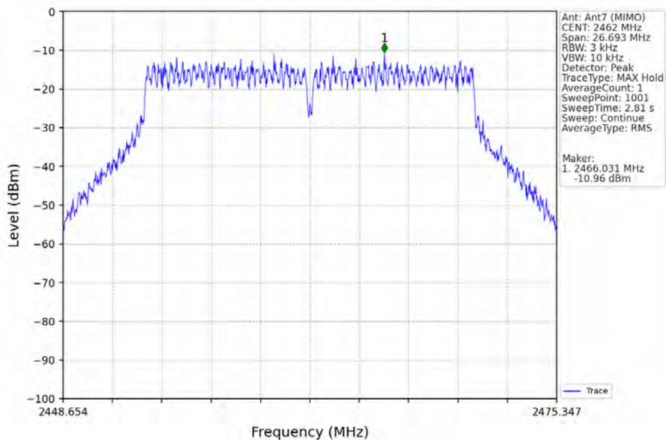
802.11n(HT20)_HCH_2462MHz_Ant7 (MIMO)_NTNV
