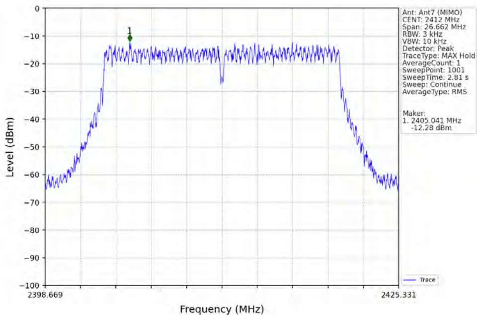
802.11n(HT20)_LCH_2412MHz_Ant7 (MIMO)_NTNV
