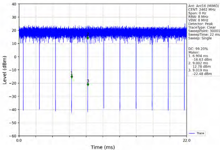
802.11g_HCH_2462MHz_Ant16 (MIMO)_NTNV
