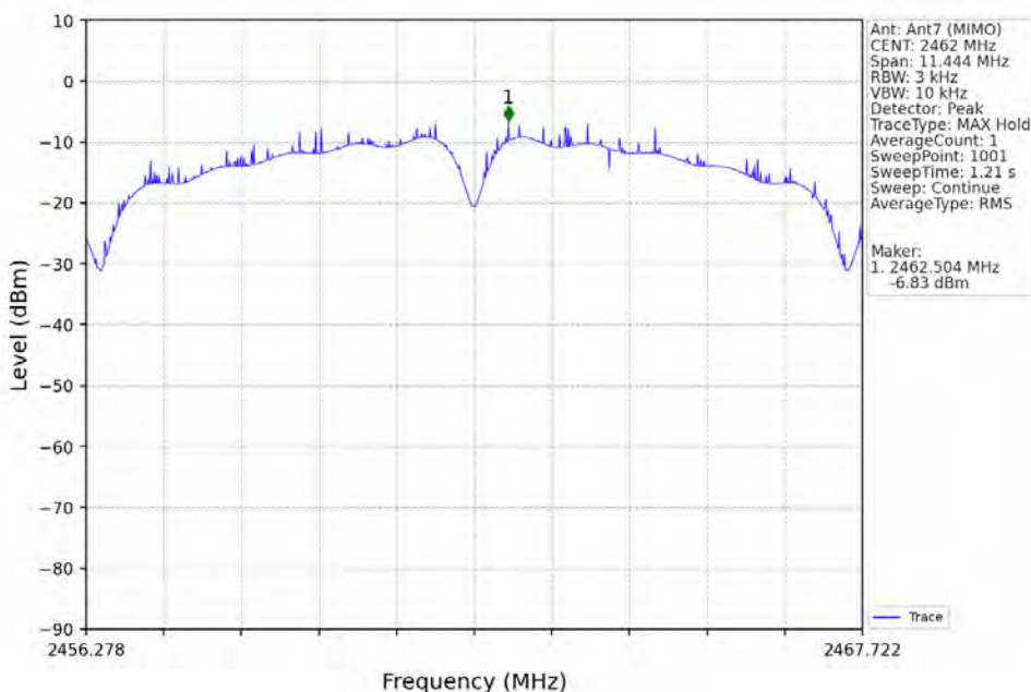
802.11b_HCH_2462MHz_Ant7 (MIMO)_NTNV
