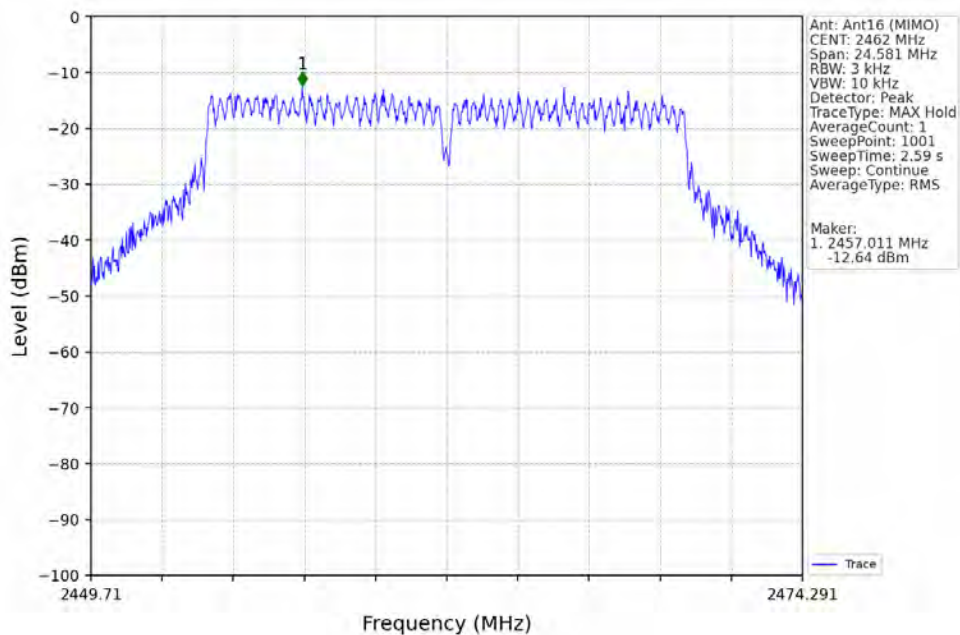
802.11g_HCH_2462MHz_Ant16 (MIMO)_NTNV
