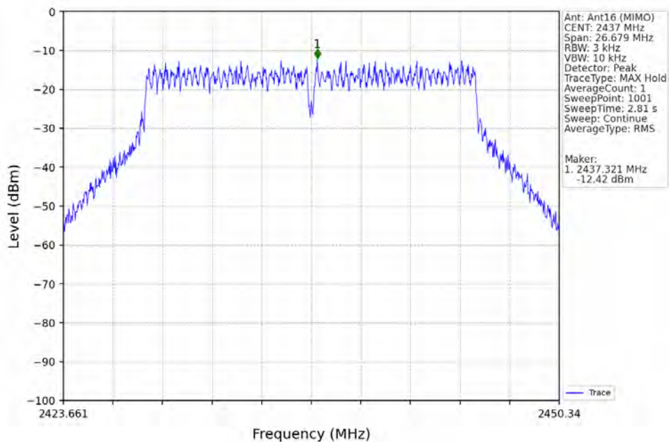
802.11n(HT20)_MCH_2437MHz_Ant16 (MIMO)_NTNV
