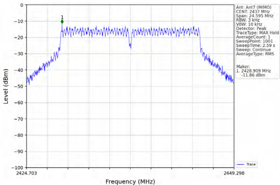
802.11g_MCH_2437MHz_Ant7 (MIMO)_NTNV
