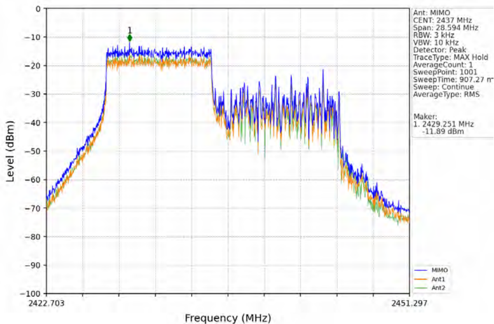
802.11be(EHT20)_MCH_2437MHz_RU106_Left_MIMO_NTNV
