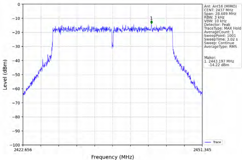
802.11ax(HEW20)_MCH_2437MHz_RU242_Left_Ant16 (MIMO)_NTNV
