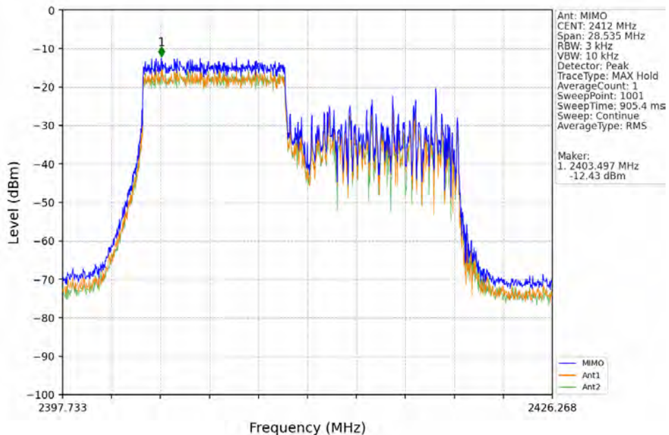
802.11be(EHT20) LCH 2412MHz RU106 Left MIMO NTNV
