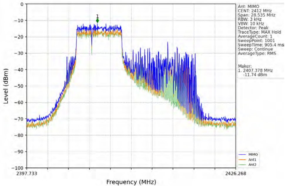
802.11be(EHT20)_LCH_2412MHz_RU106_Left_Ant16(MIMO)_NTNV
