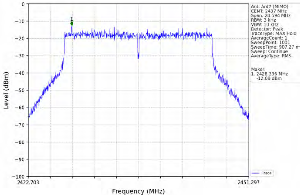
802.11be(EHT20)_MCH_2437MHz_RU242_Left_MIMO_NTNV
