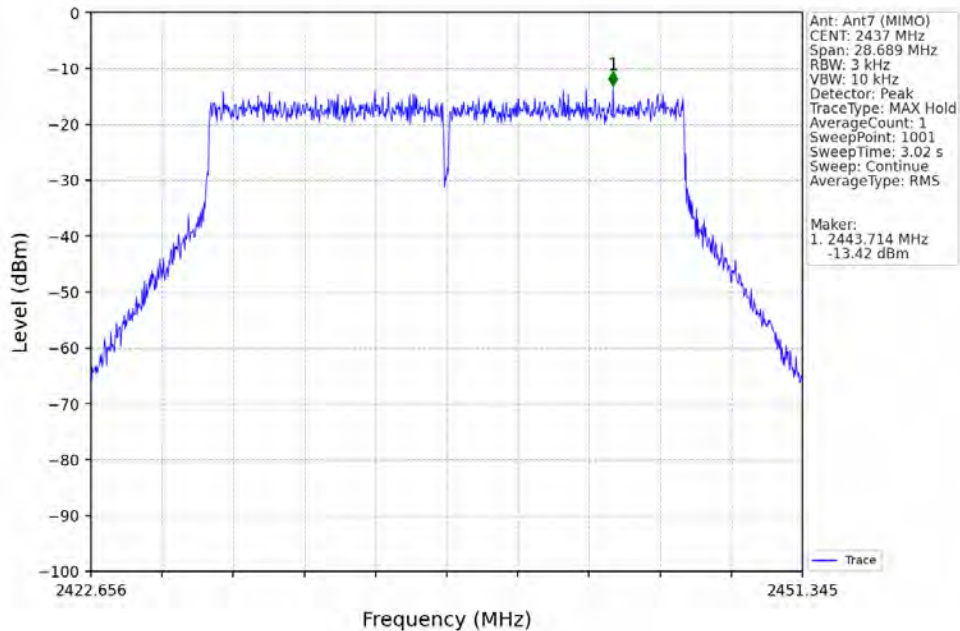
802.11ax(HEW20)_MCH_2437MHz_RU242_Left_MIMO_NTNV
