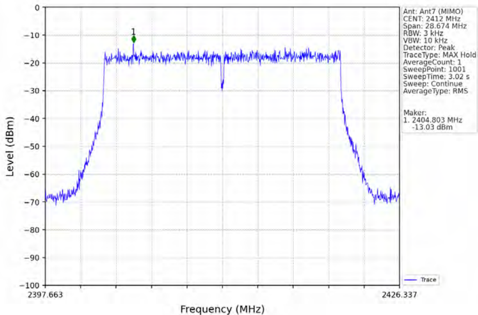
802.11ax(HEW20)_LCH_2412MHz_RU242_Left_Ant7 (MIMO)_NTNV
