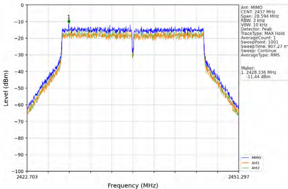
802.11be(EHT20)_MCH_2437MHz_RU242_Left_MIMO_NTNV
