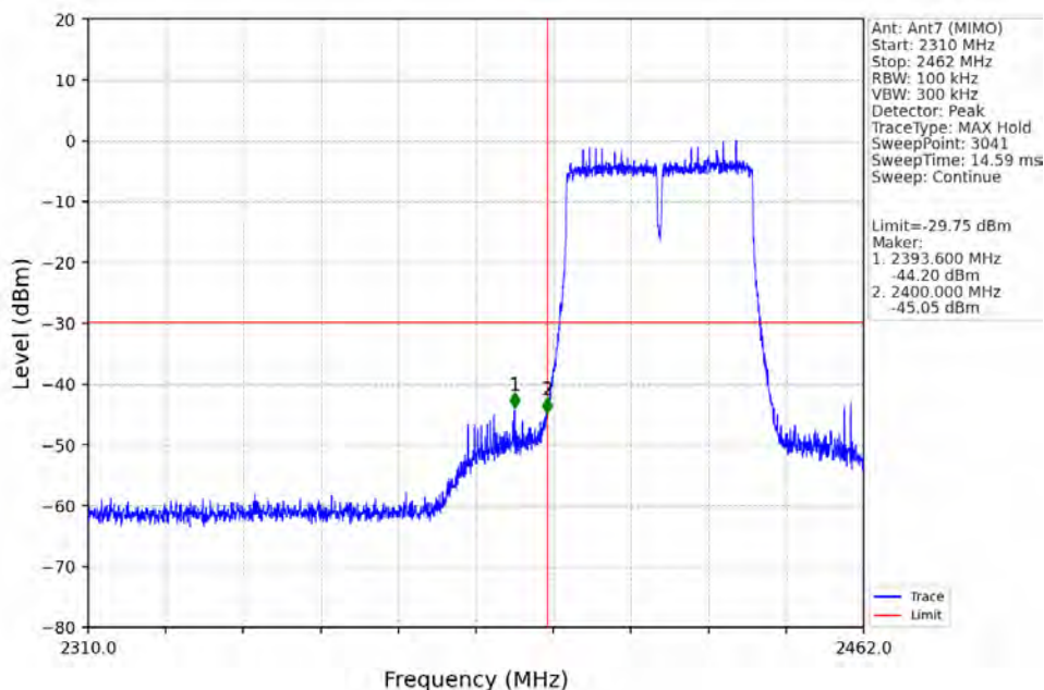
802.11n(HT40)_LCH_2422MHz_Ant7 (MIMO)_NTNV
