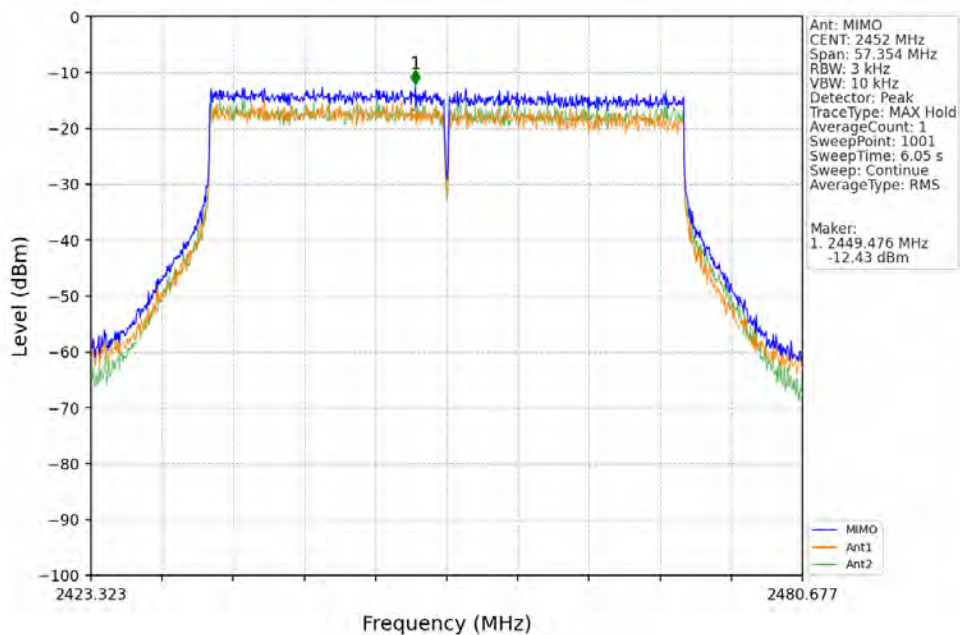
802.11be(EHT40)_HCH_2452MHz_RU484_Left_MIMO_NTNV
