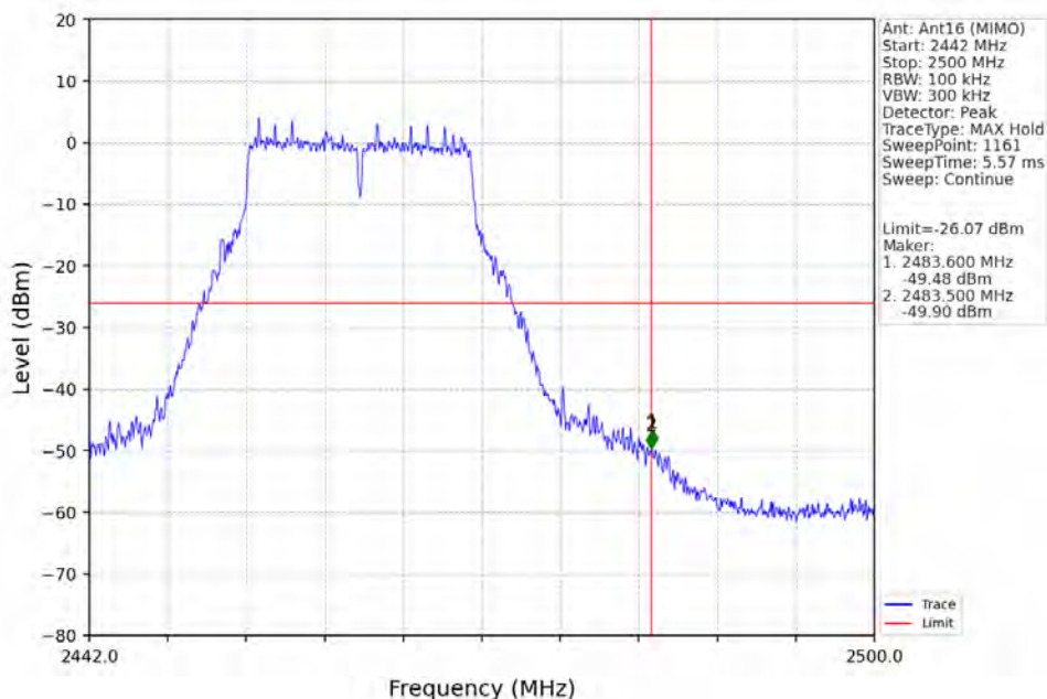
802.11g_HCH_2462MHz_Ant16 (MIMO)_NTNV
