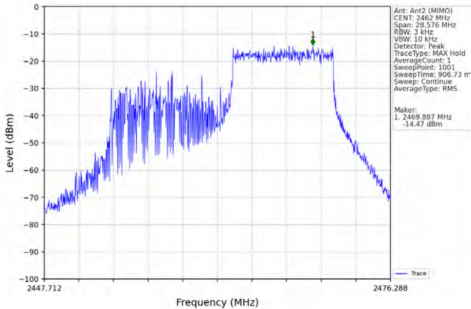
802.11be(EHT20) HCH 2462MHz RU106 Right MIMO NTN
