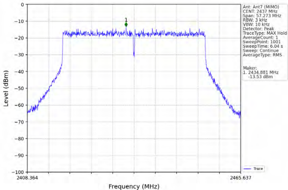
802.11ax(HEW40)_MCH_2437MHz_RU484_Left_Ant7 (MIMO)_NTNV
