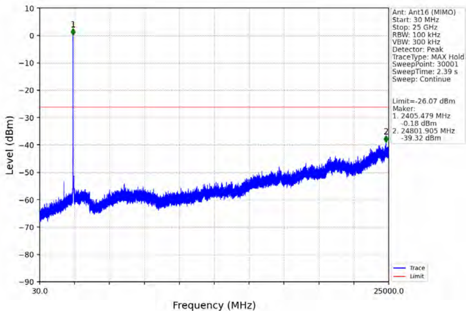
802.11g_LCH_2412MHz_Ant16 (MIMO)_NTNV
