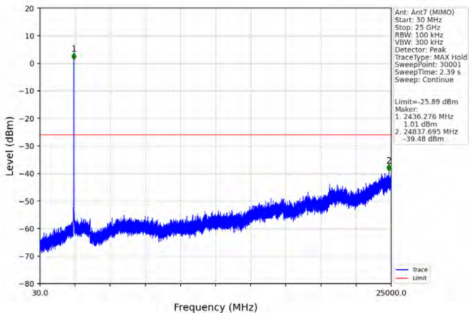
802.11g_MCH_2437MHz_Ant7 (MIMO)_NTNV
