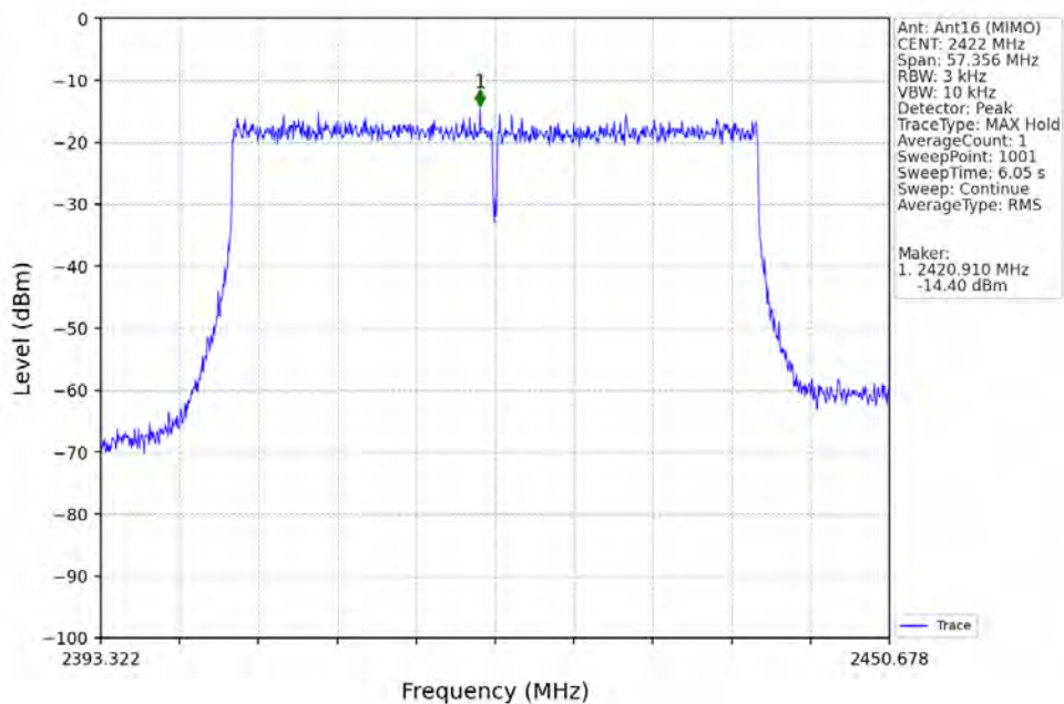
802.11ax(HEW40)_LCH_2422MHz_RU484_Left_Ant16 (MIMO)_NTNV
