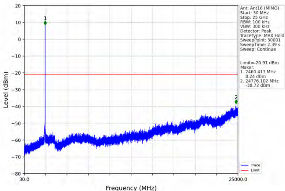
802.11b_HCH_2462MHz_Ant16 (MIMO)_NTNV
