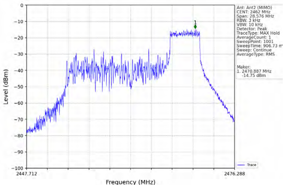
802.11be(EHT20)_HCH_2462MHz_RU52_Right_MIMO_NTNV
