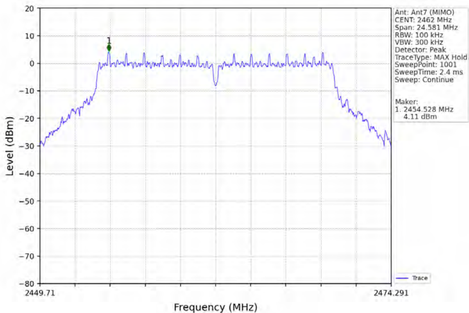
802.11g_HCH_2462MHz_Ant7 (MIMO)_NTNV
