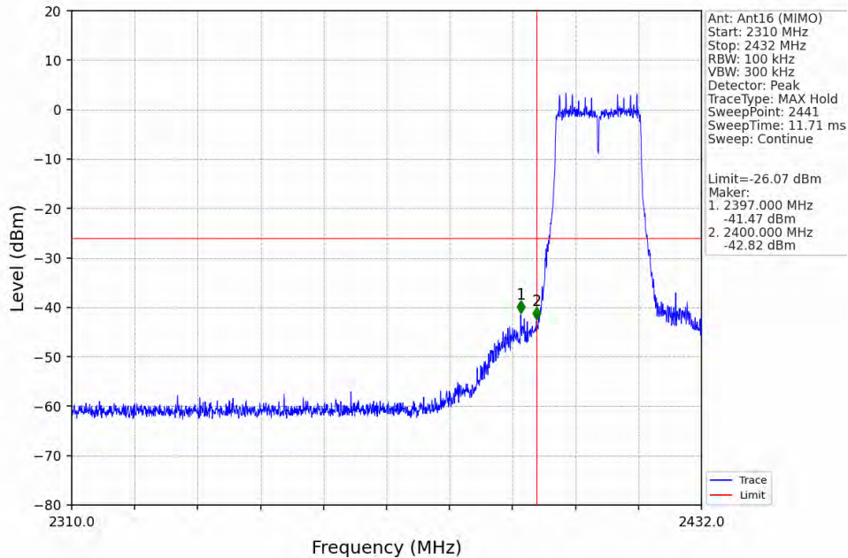
802.11g_LCH_2412MHz_Ant16 (MIMO)_NTNV
