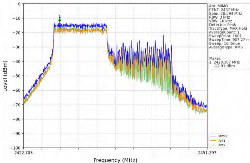
802.11be(EHT20) MCH 2437MHz RU106 Right MIMO NTN
