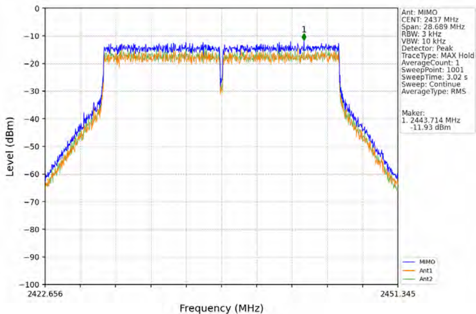
802.11ax(HEW20)_MCH_2437MHz_RU242_Left_MIMO_NTNV
