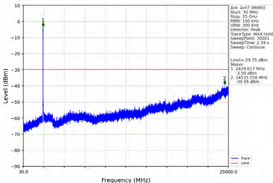
802.11n(HT40)_LCH_2422MHz_Ant7 (MIMO)_NTNV
