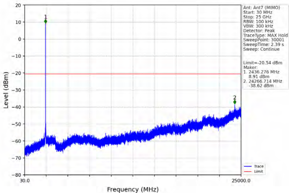
802.11b_MCH_2437MHz_Ant7 (MIMO)_NTNV
