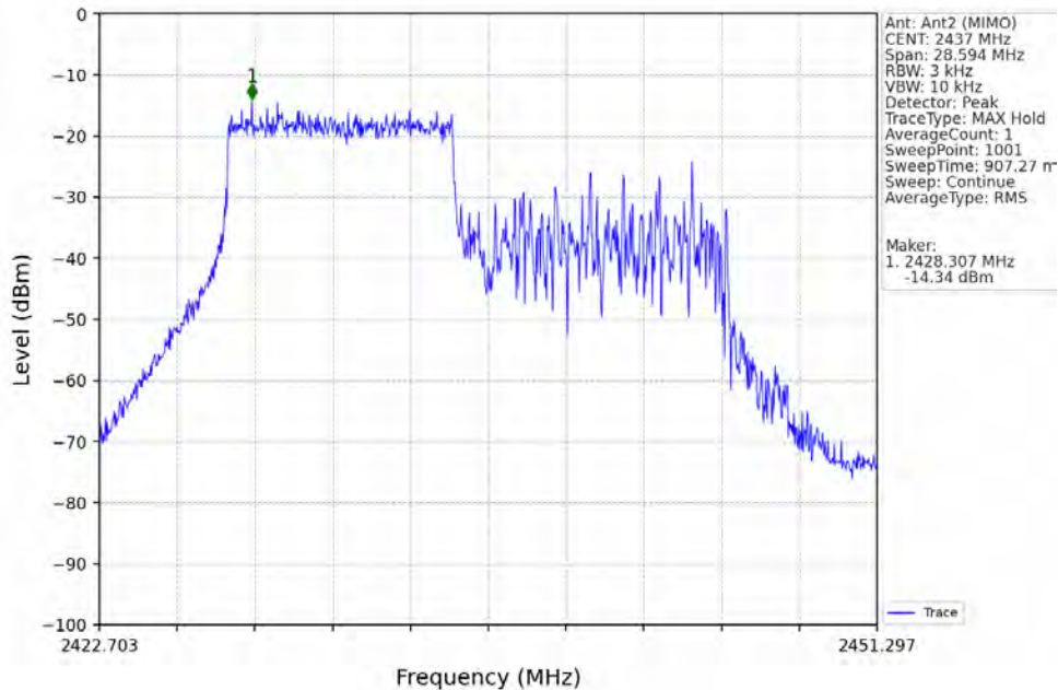
802.11be(EHT20)_MCH_2437MHz_RU106_Left_MIMO_NTNV
