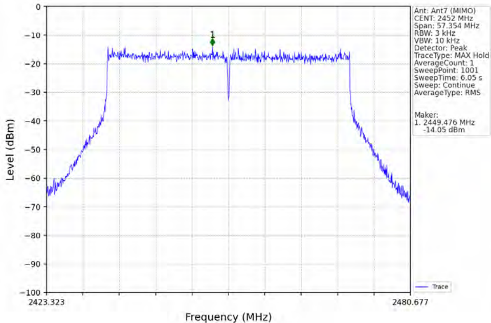
802.11be(EHT40)_HCH_2452MHz_RU484_Left_MIMO_NTNV
