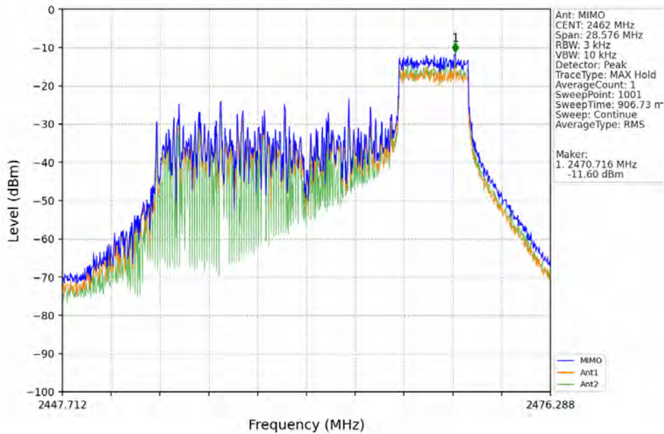
802.11be(EHT20) HCH 2462MHz RU106 Right Ant16 (MIMO) NTN
