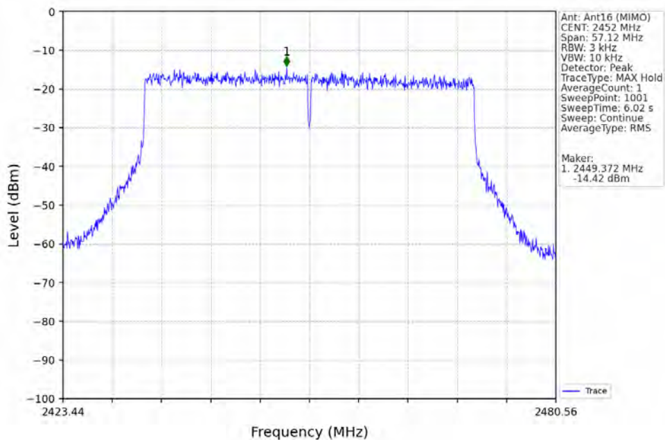
802.11ax(HEW40)_HCH_2452MHz_RU484_Left_Ant16 (MIMO)_NTNV
