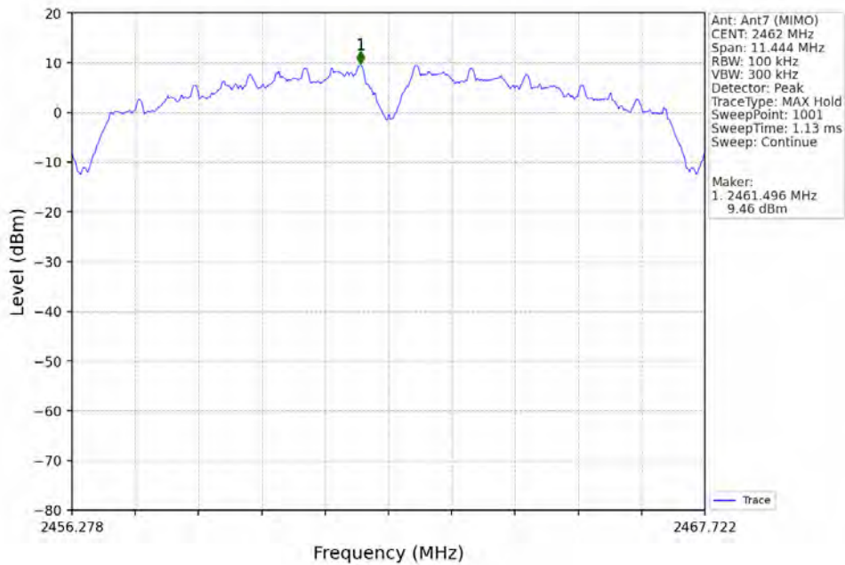
802.11b_HCH_2462MHz_Ant7 (MIMO)_NTNV
