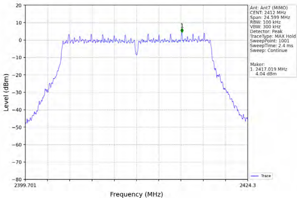
802.11g_LCH_2412MHz_Ant7 (MIMO)_NTNV
