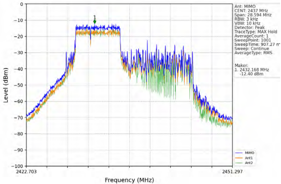
802.11be(EHT20) MCH 2437MHz RU106 Right Ant16 (MIMO) NTN
