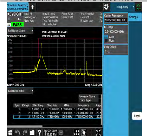
Band66-20MHz-QPSK-132572-1RB#99-PASS
