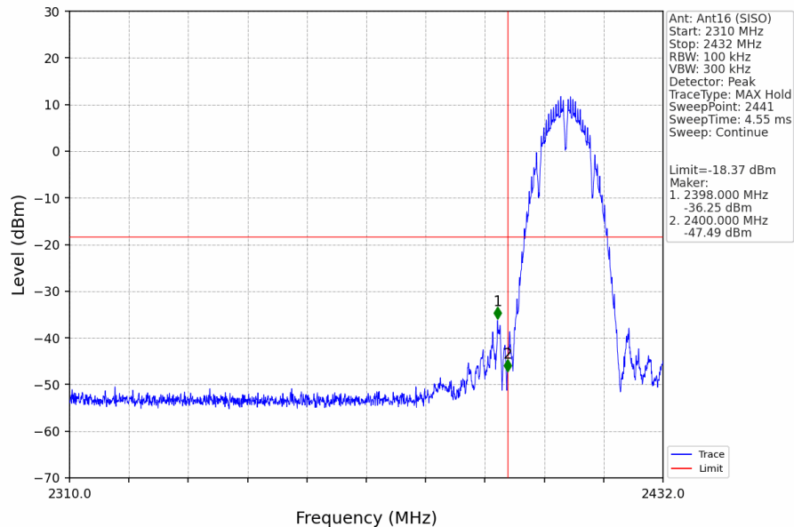
802.11b_LCH_2412MHz_Ant16 (SISO)_NTNV
