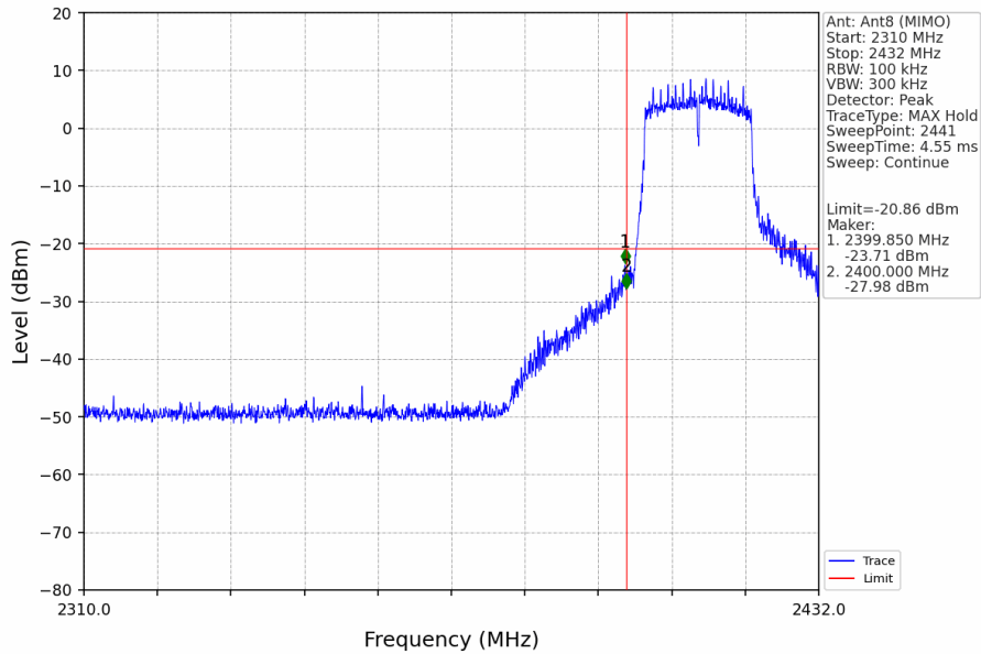
802.11n(HT20)_LCH_2412MHz_Ant8 (MIMO)_NTNV
