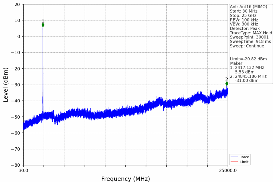
802.11g_LCH_2412MHz_Ant16 (MIMO)_NTNV
