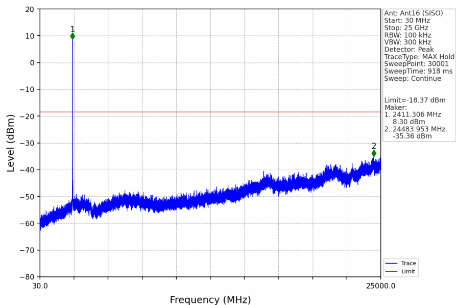
802.11b_LCH_2412MHz_Ant16 (SISO)_NTNV
