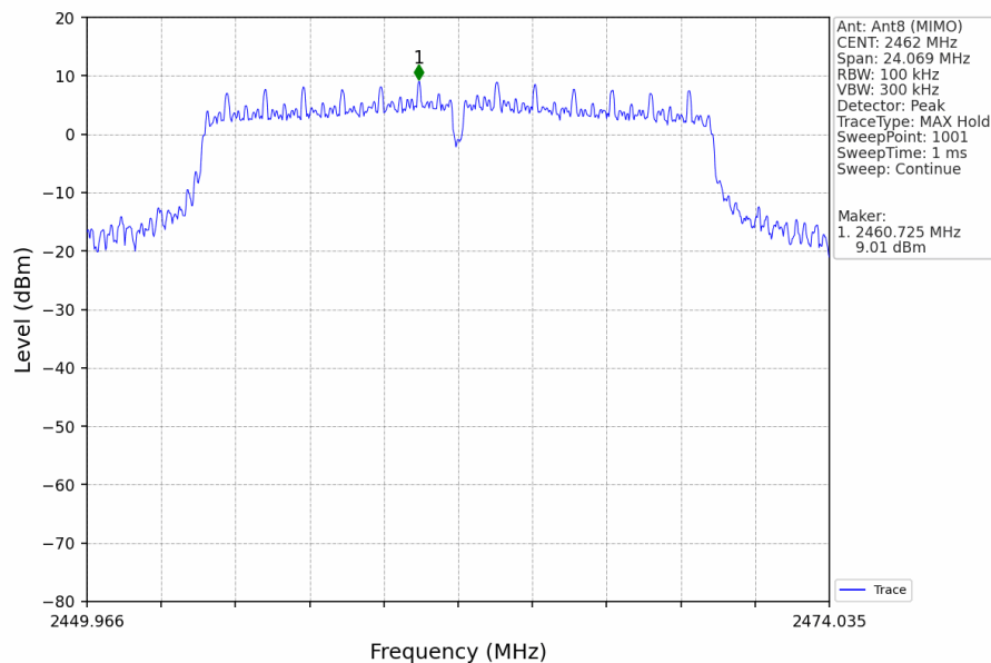
802.11g_HCH_2462MHz_Ant8 (MIMO)_NTNV
