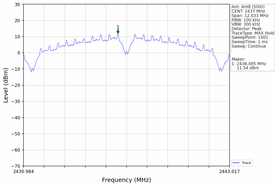
802.11b_MCH_2437MHz_Ant8 (SISO)_NTNV
