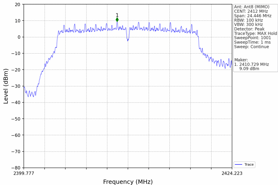
802.11g_LCH_2412MHz_Ant8 (MIMO)_NTNV
