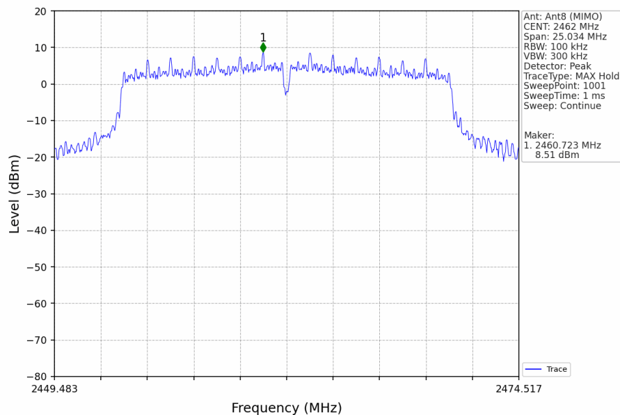
802.11n(HT20)_HCH_2462MHz_Ant8 (MIMO)_NTNV
