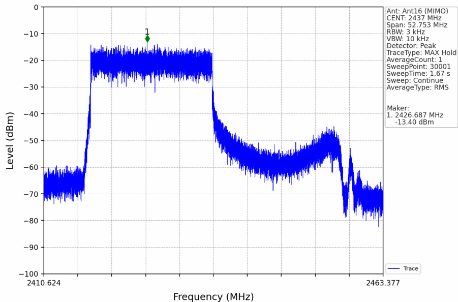
802.11ax(HEW40)_MCH_2437MHz_RU242_Left_Ant16 (MIMO)_NTNV
