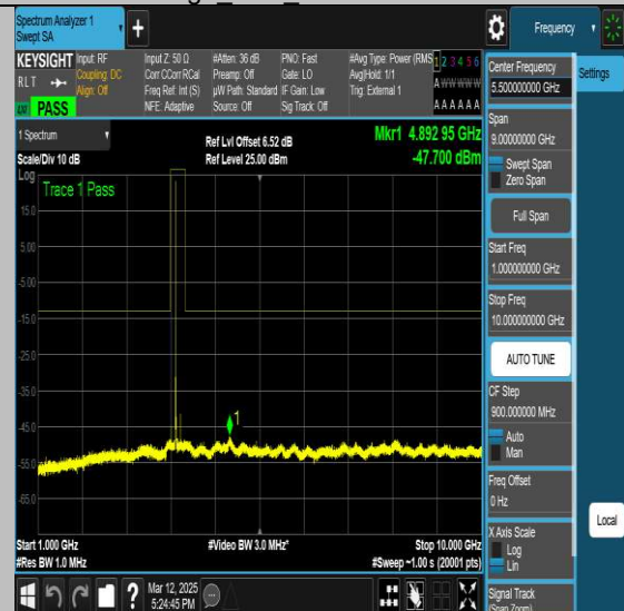
NTNV-N77-3700-3980-PC2-30-100-M-DFT-QPSK- Edge 1RB Left-Ant1-PASS
