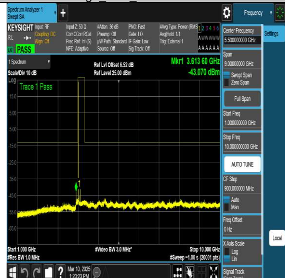
NTNV-N77-3700-3980-PC2-30-90-L-DFT-QPSK- Edge 1RB Left-Ant1-PASS
