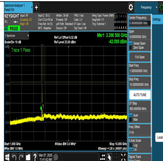
NTNV-N77-3450-3550-PC2-30-70-M-DFT-QPSK- Edge 1RB Left-Ant1-PASS
