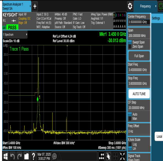
NTNV-N77-3450-3550-PC2-30-50-L-DFT-QPSK- Edge 1RB Left-Ant1-PASS
