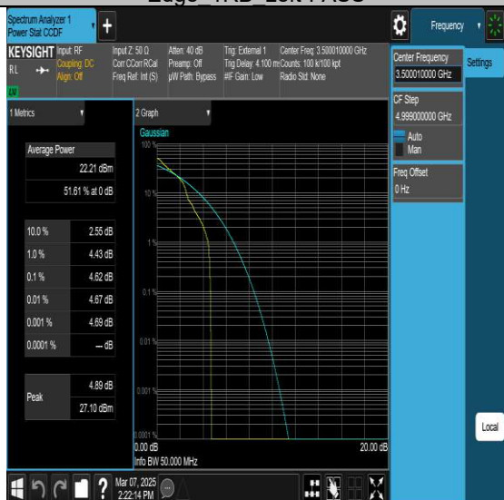
NTNV-N77-3450-3550-PC2-30-50-M-DFT-QPSK-Edge 1RB Left-PASS
