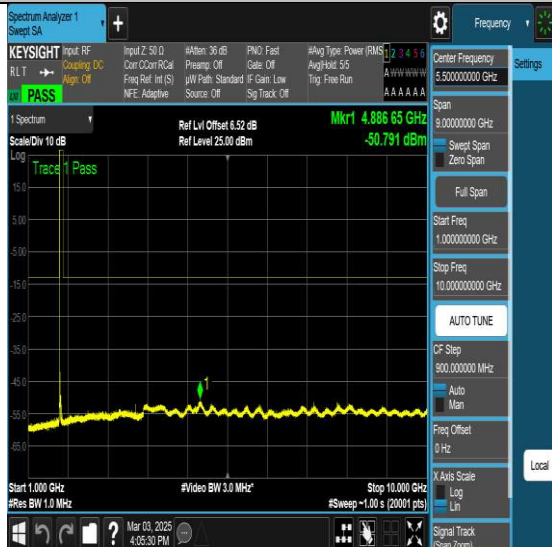
NTVN-N66-PC3-15-20-L-DFT-QPSK-Edge_1RB_Left-Ant1-PASS
