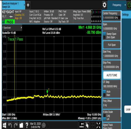
NTVN-N66-PC3-15-5-M-DFT-QPSK-Edge_1RB_Left-Ant1-PASS
