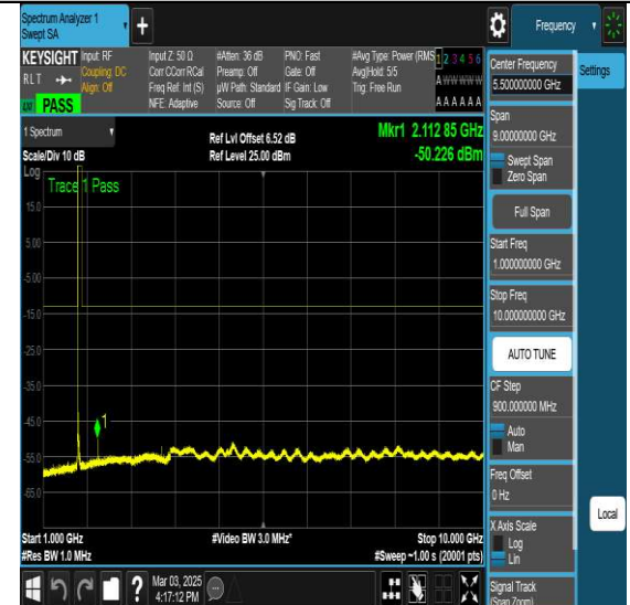
NTVN-N66-PC3-15-40-L-DFT-QPSK-Edge_1RB_Left-Ant1-PASS
