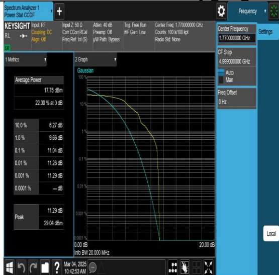
NTNV-N66-PC3-15-20-H-DFT-QPSK-Edge 1RB Left-PASS
