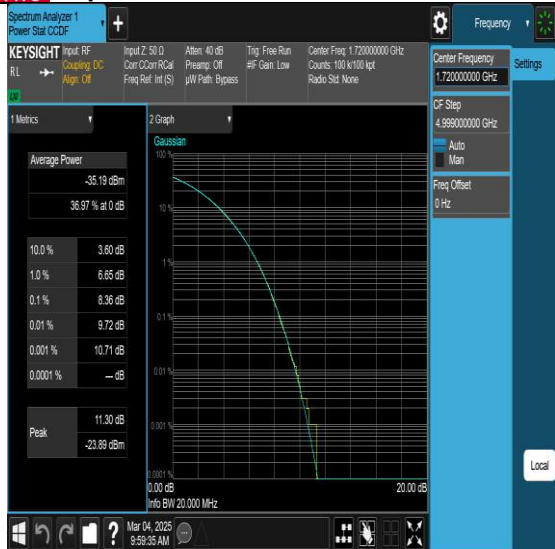
NTNV-N66-PC3-15-20-L-DFT-QPSK-Edge 1RB Left-PASS
