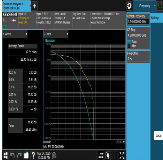
NTNV-N66-PC3-15-20-M-DFT-QPSK-Edge 1RB Left-PASS
