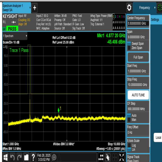
NTVN-N41-PC3-30-30-H-DFT-QPSK-Edge_1RB_Left-Ant1-PASS
