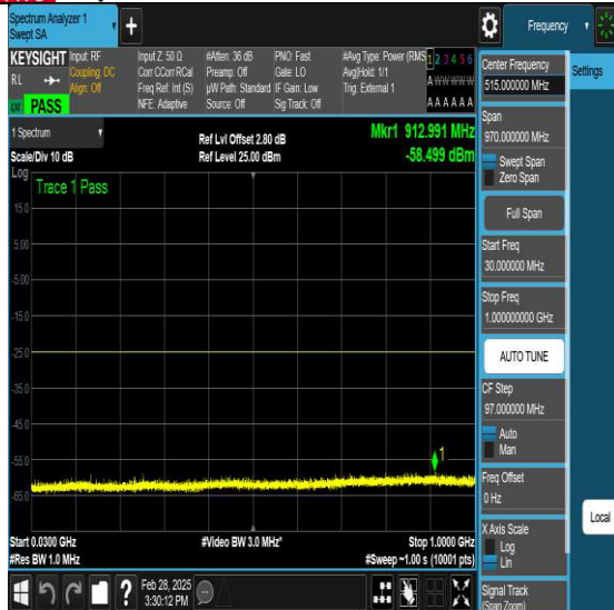
NTVN-N41-PC3-30-30-M-DFT-QPSK-Edge_1RB_Left-Ant1-PASS
