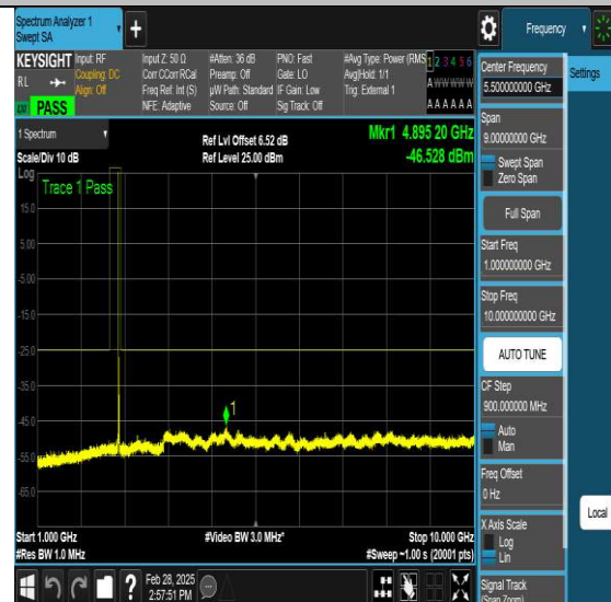
NTVN-N41-PC3-30-20-H-DFT-QPSK-Edge_1RB_Left-Ant1-PASS
