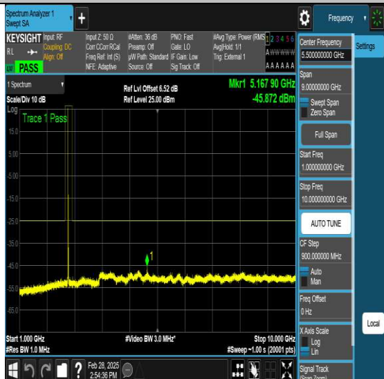
NTVN-N41-PC3-30-20-M-DFT-QPSK-Edge_1RB_Left-Ant1-PASS
