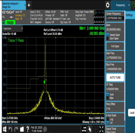
NTNV-N7-PC3-15-40-L-DFT-QPSK-Edge_1RB_Left-Ant1-PASS
