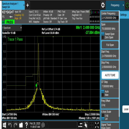
NTNV-N7-PC3-15-50-L-DFT-QPSK-Edge_1RB_Left-Ant1-
