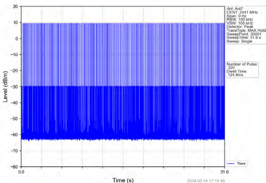
Pi/4DQPSK_2DH1_HOPP_Ant7_NTNV
