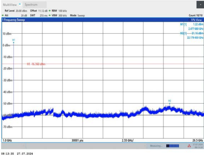
BLE_2M_Ant1_2478_1000~26500
