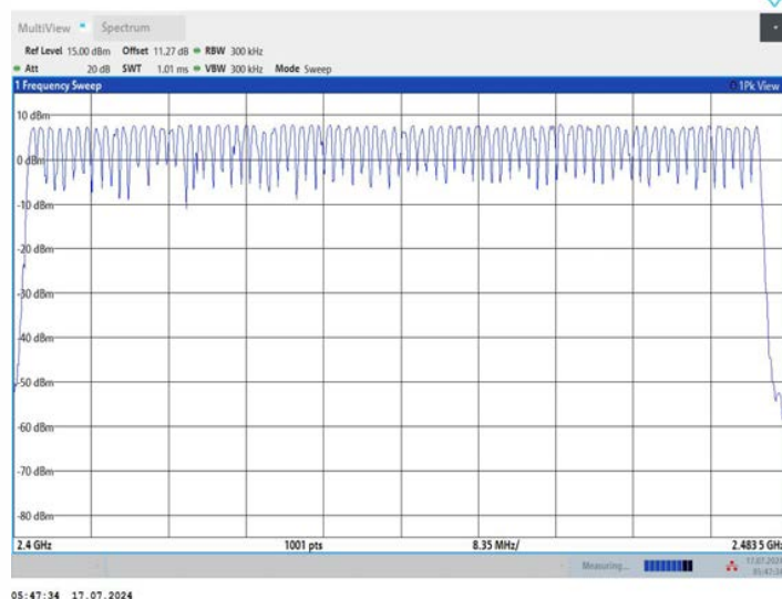
2DH5_Ant1_Hop
