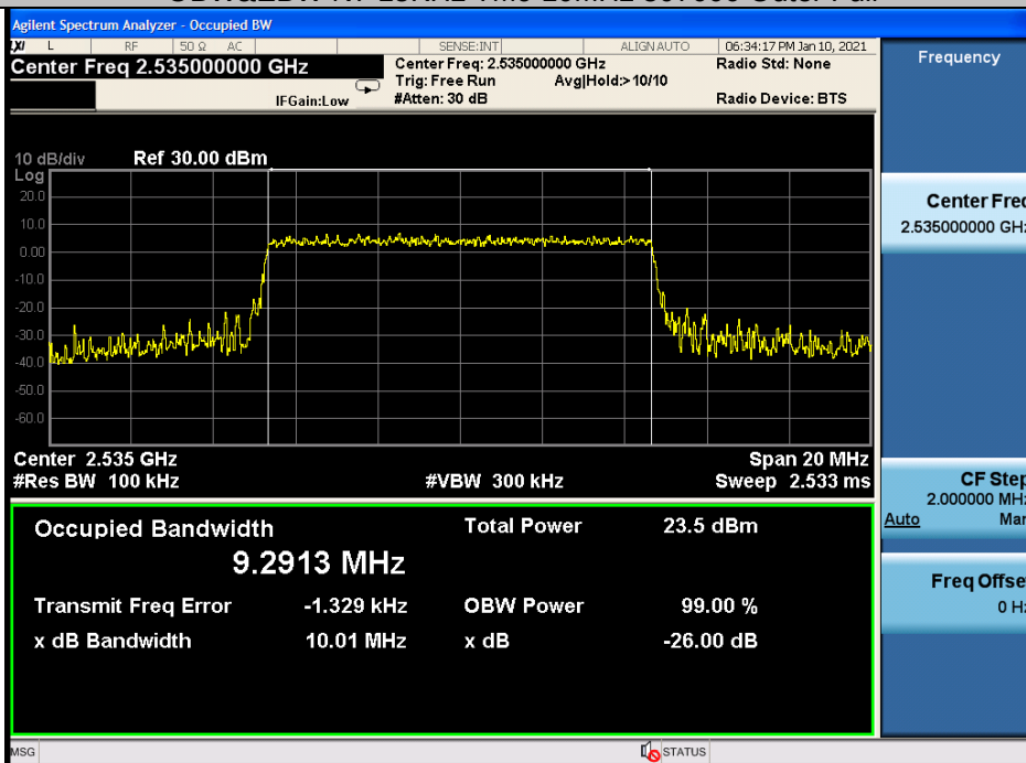
OBW&amp;EBW N7 15KHz TM9 10MHz 507000 Outer Full
