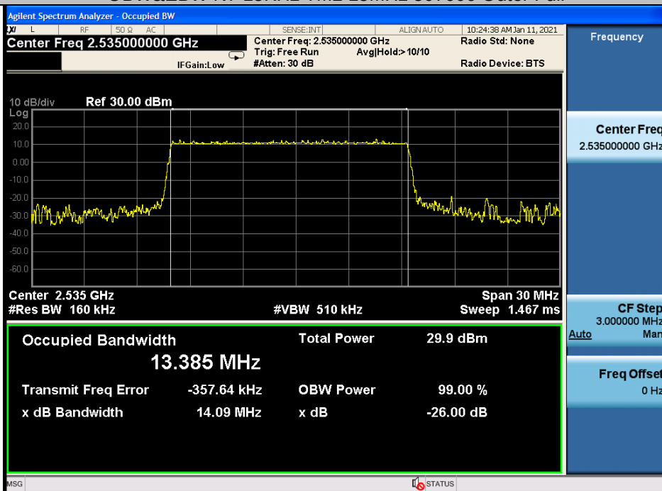
OBW&amp;EBW N7 15KHz TM2 15MHz 507000 Outer Full
