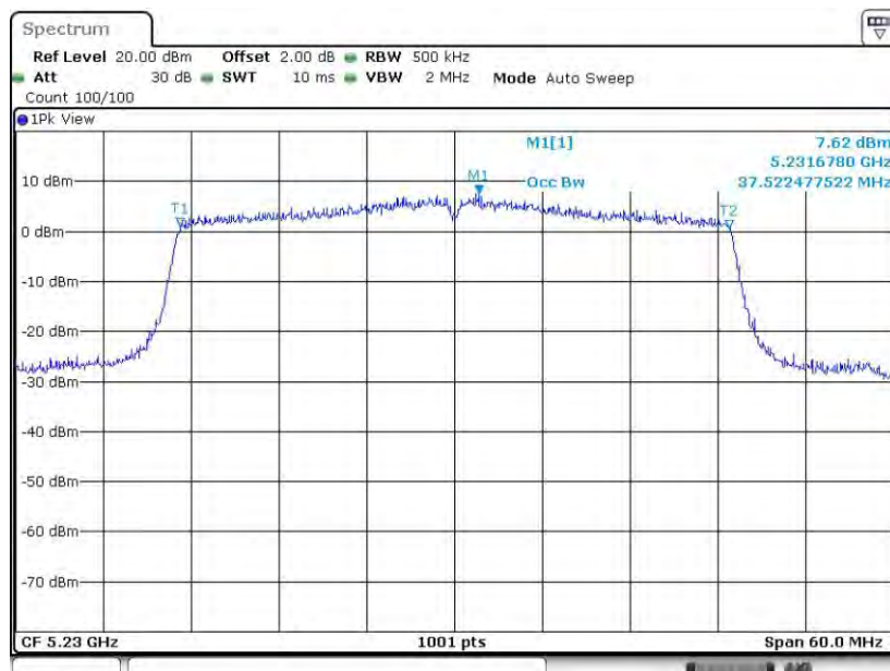
11AX40MIMO-484T Ant1 5230
