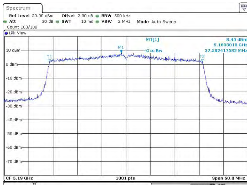
11AX40MIMO-484T Ant2 5190
