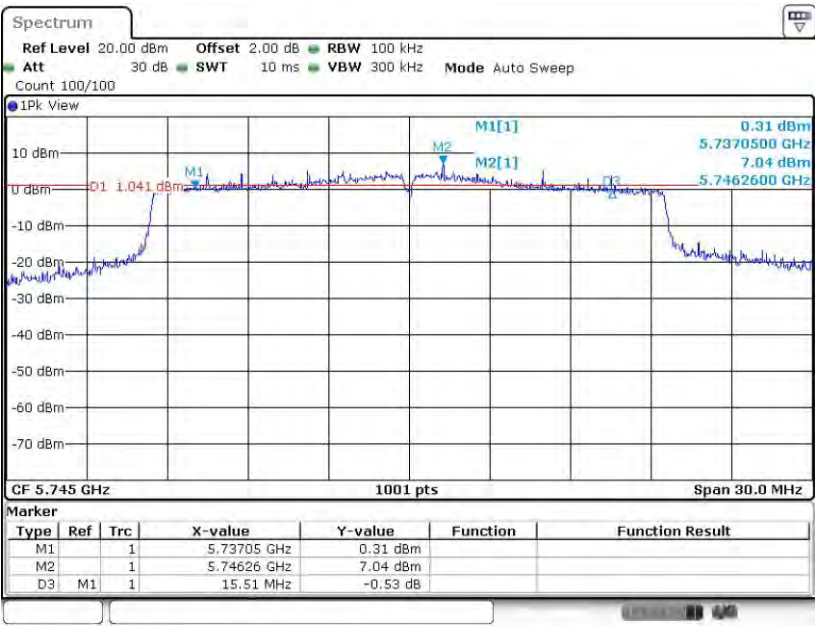
11AX20MIMO-242T_Ant1_5745
