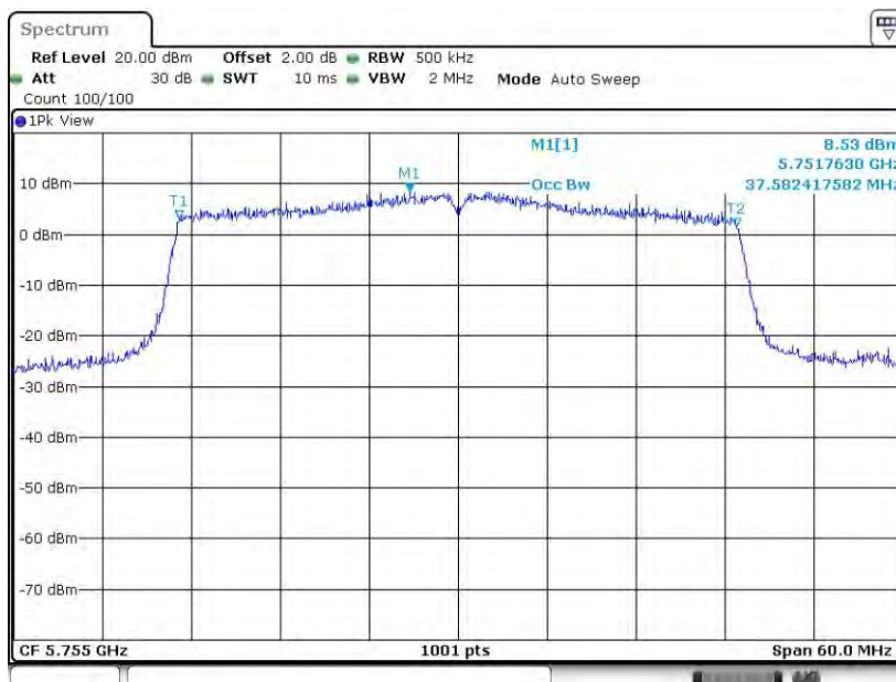
11AX40MIMO-484T_Ant1_5755
