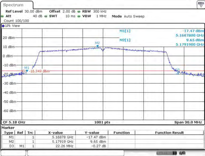
11AX20MIMO-242T_Ant1_5180
