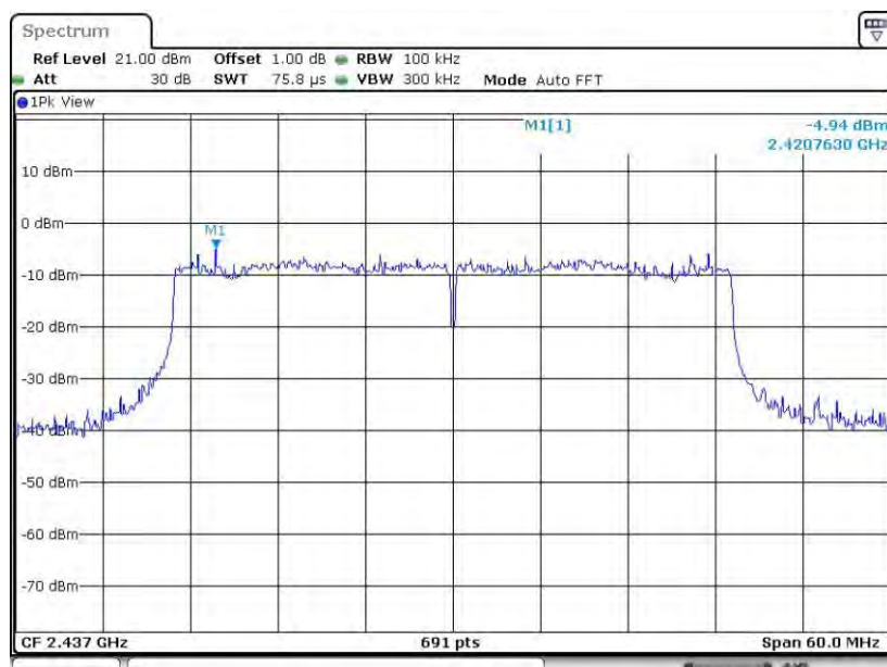
11AX40MIMO-484T Ant1 2437 0~Reference
