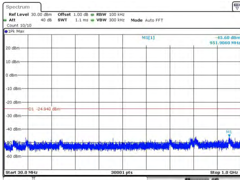
11AX40MIMO-484T Ant1 2437 30~1000
