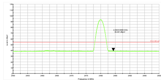
BLE Channel 39 Average
