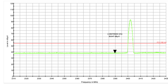
BLE Channel 0 Average
