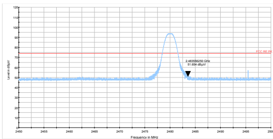
BLE Channel 39 Peak
