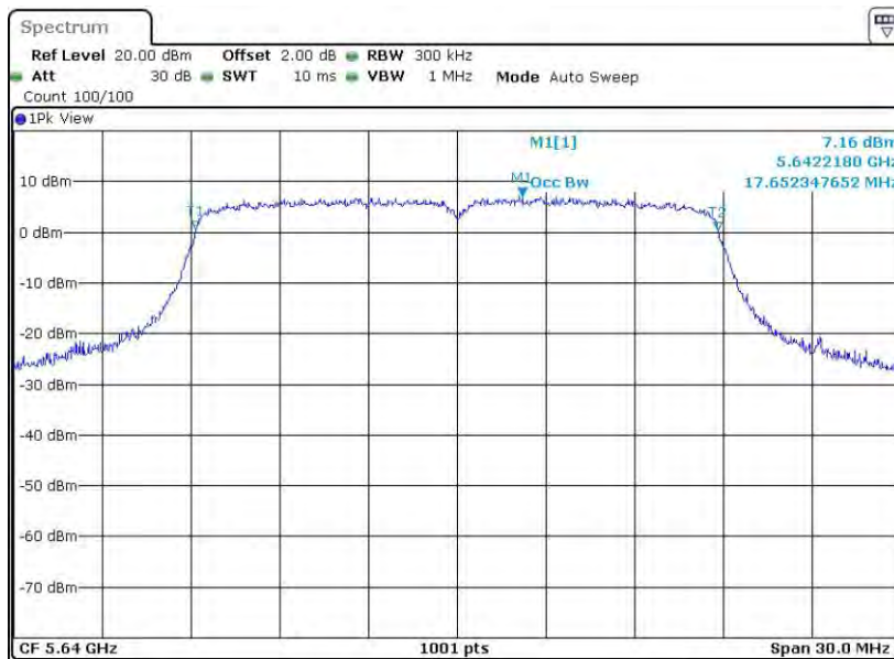
11N20MIMO_Ant2_5640
