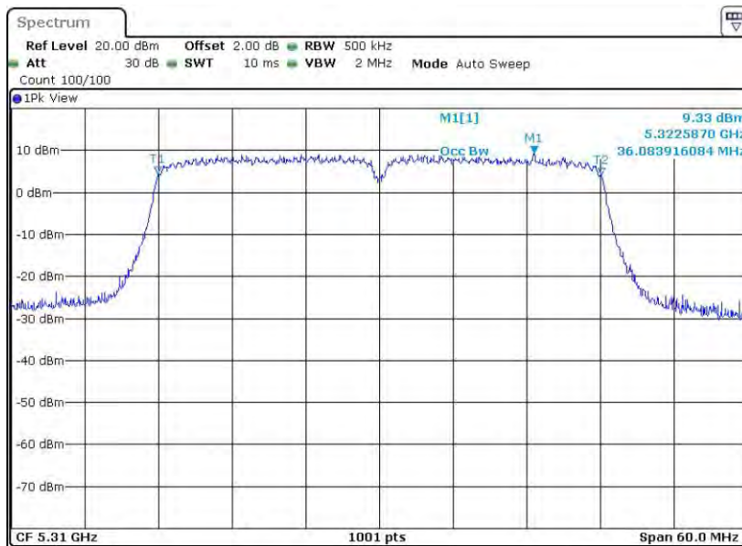
11N40MIMO_Ant2_5310
