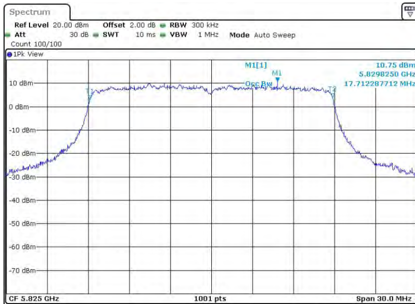
11AC20MIMO_Ant1_5825
