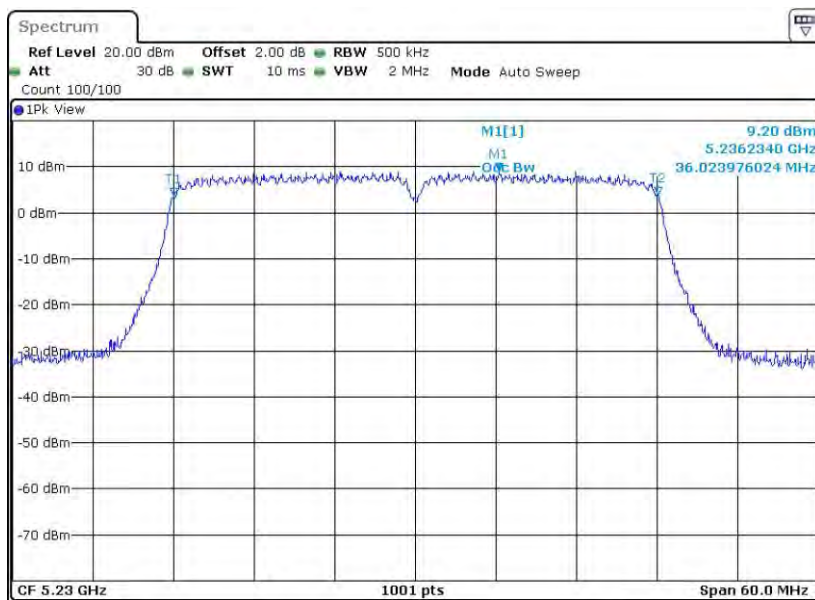
11N40MIMO_Ant2_5230
