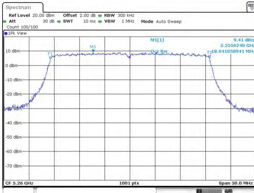
11AX20MIMO_Ant2_5260
