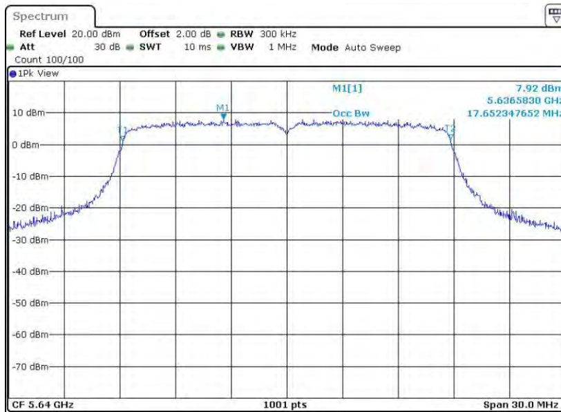
11N20MIMO_Ant1_5640
