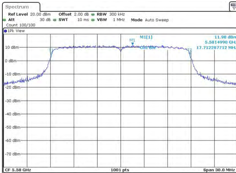
11N20MIMO_Ant1_5580
