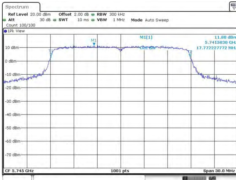
11N20MIMO_Ant1_5745
