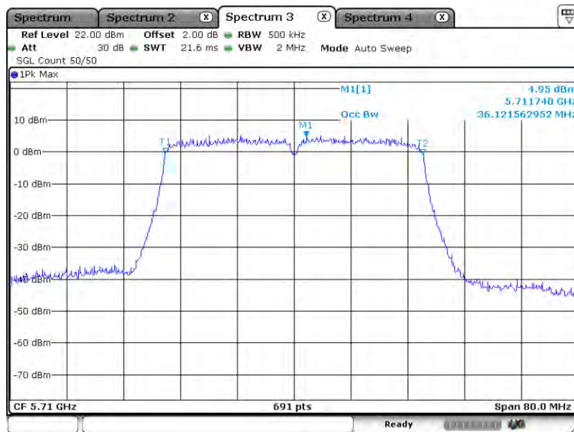
11N40MIMO_Ant2_5710
