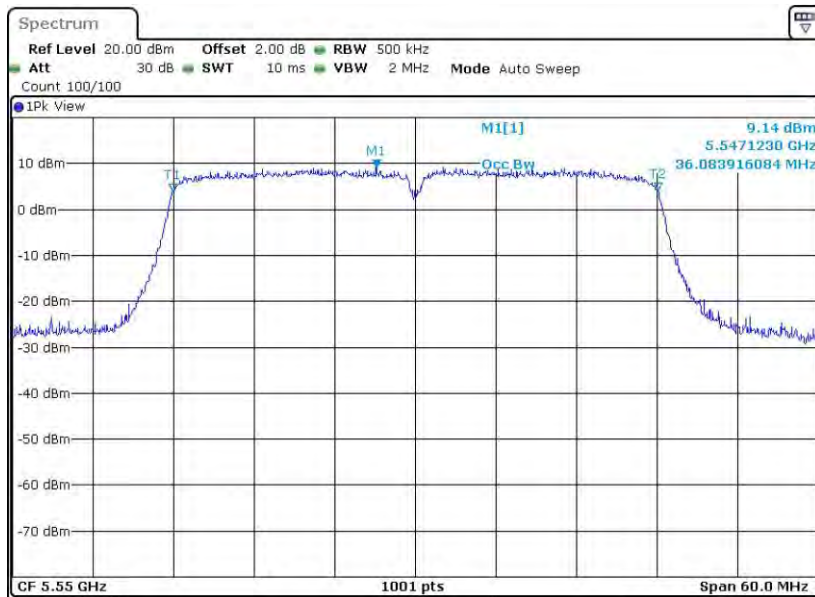
11N40MIMO_Ant1_5550
