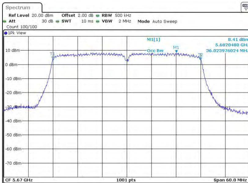
11N40MIMO_Ant2_5670
