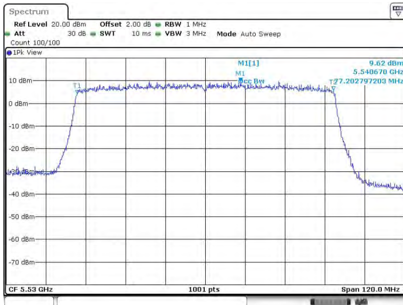
11AC80MIMO_Ant1_5530
