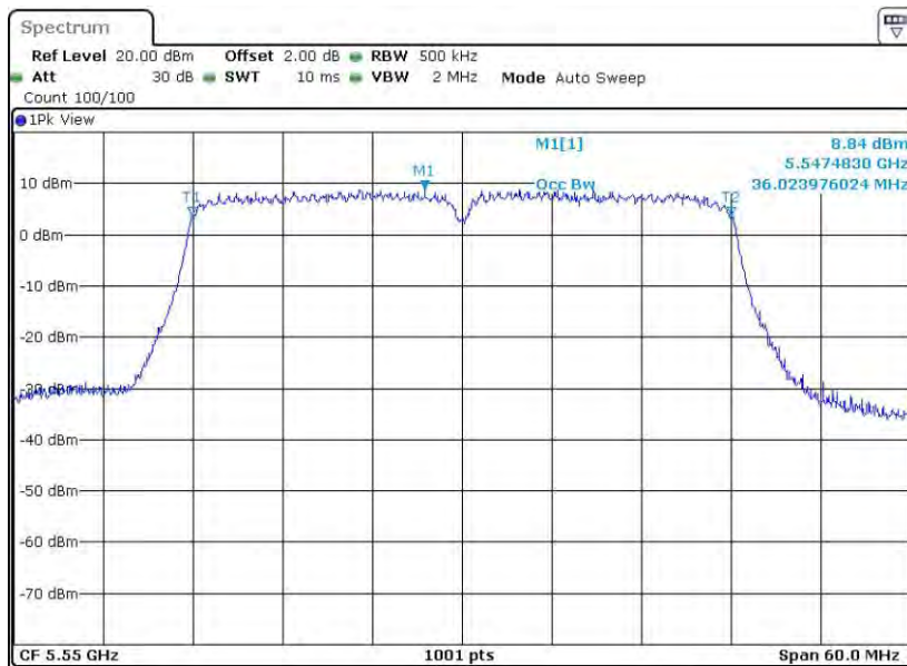
11N40MIMO_Ant2_5550
