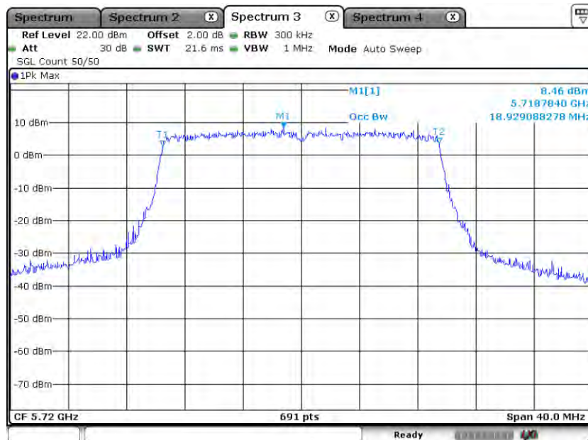
11AX20MIMO_Ant2_5720
