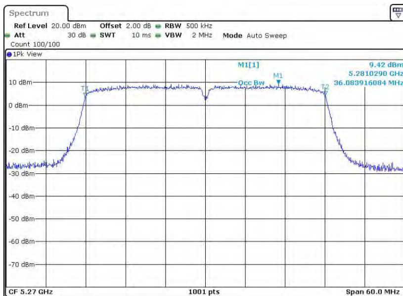
11N40MIMO_Ant1_5270
