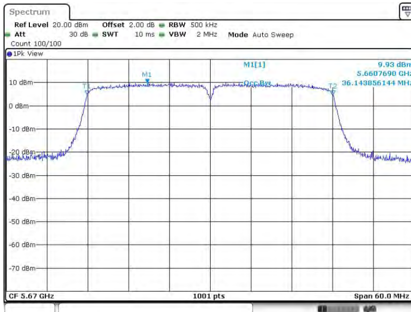
11N40MIMO_Ant1_5670
