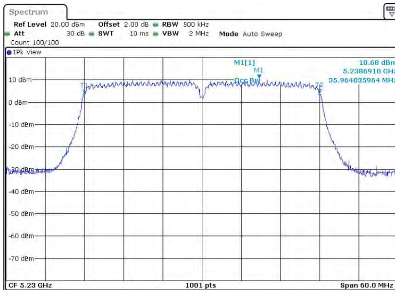
11AC40MIMO_Ant2_5230
