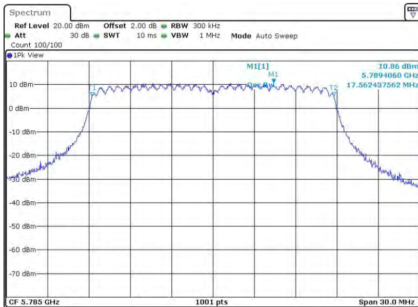
11AC20MIMO_Ant2_5785
