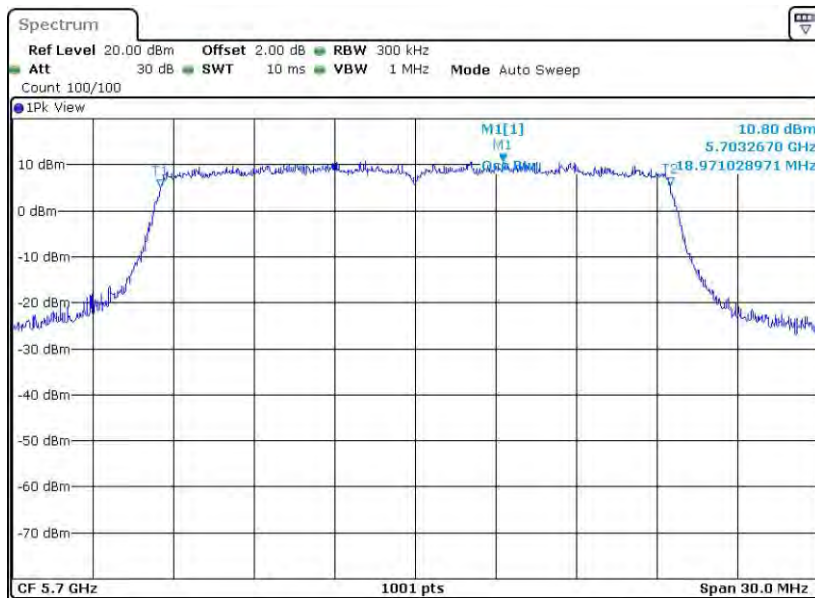
11AX20MIMO_Ant1_5700
