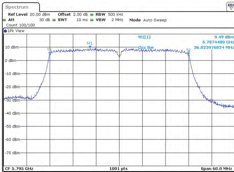
11N40MIMO_Ant2_5795
