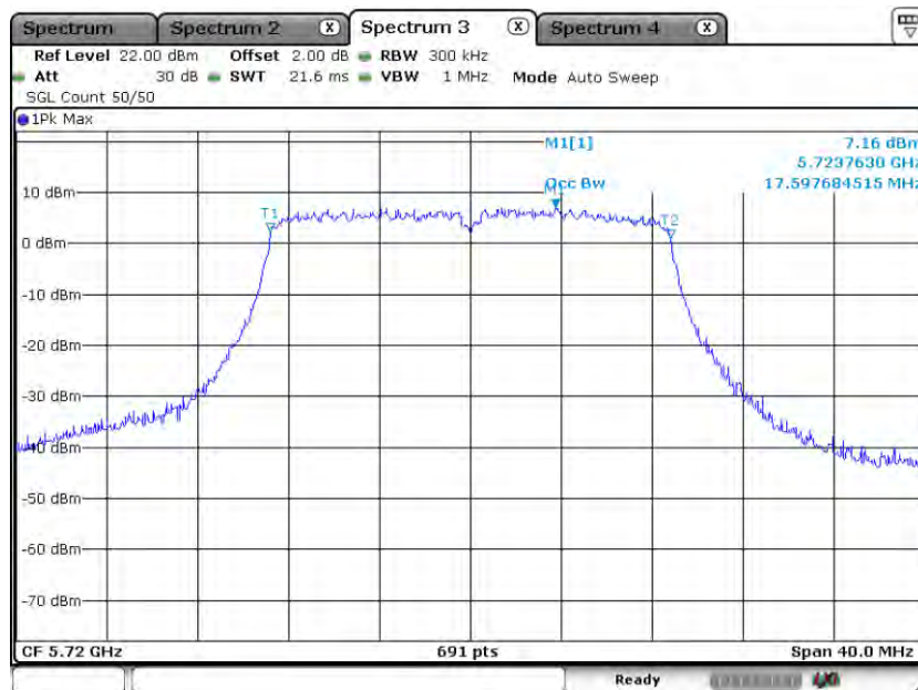
11N20MIMO_Ant2_5720
