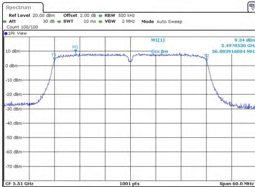
11N40MIMO_Ant1_5510
