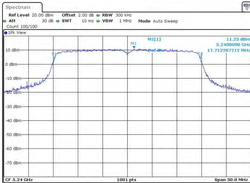
11N20MIMO_Ant1_5240
