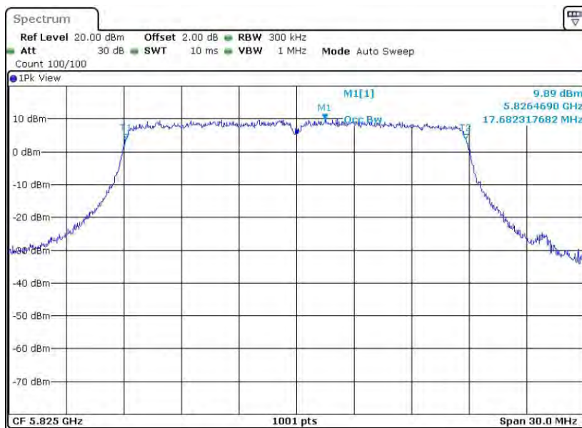
11N20MIMO_Ant2_5825
