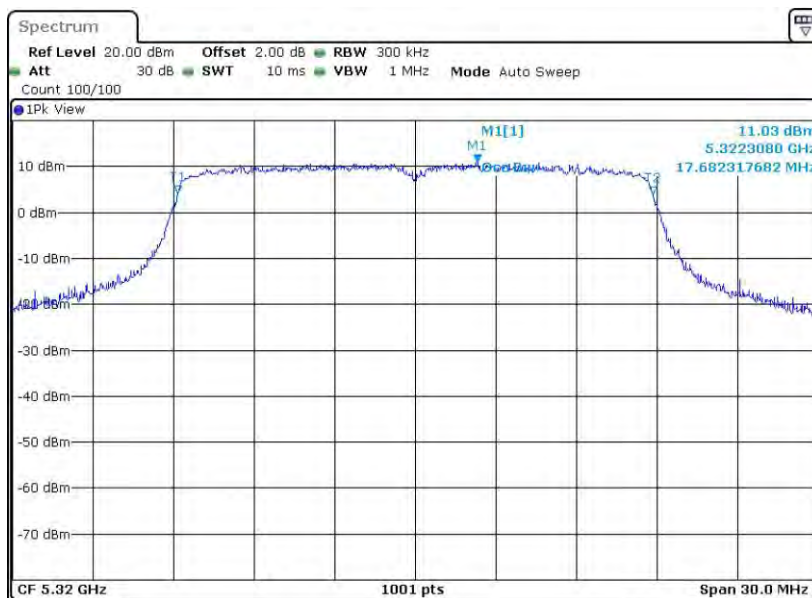
11N20MIMO_Ant1_5320
