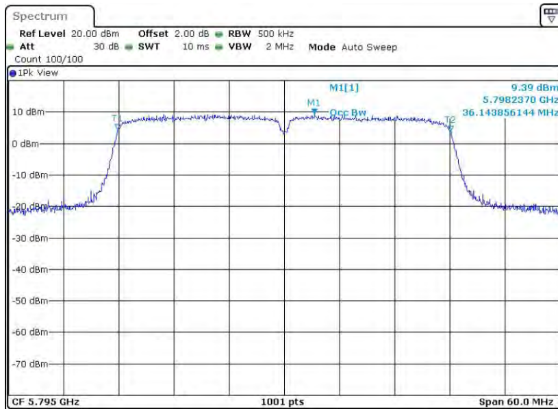
11N40MIMO_Ant1_5795
