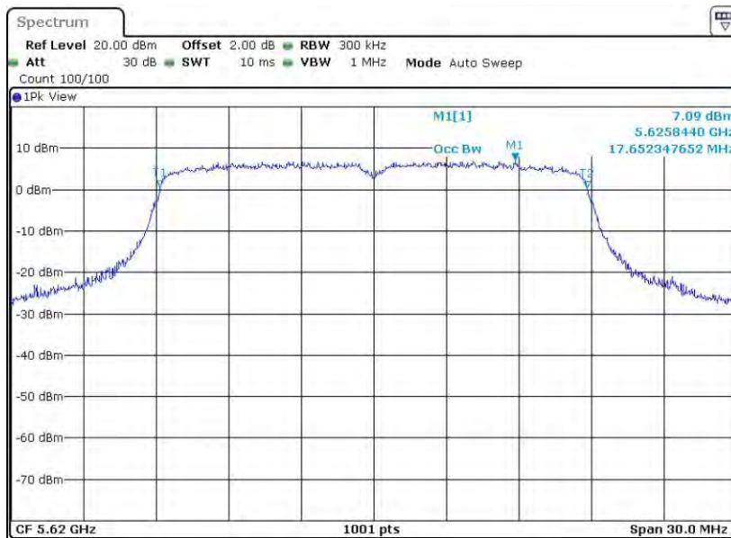
11N20MIMO_Ant2_5620
