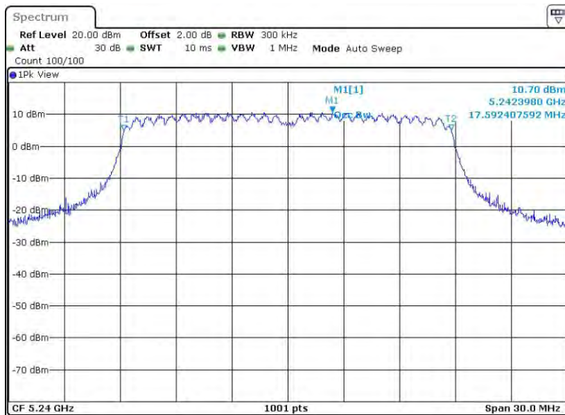
11AC20MIMO_Ant2_5240
