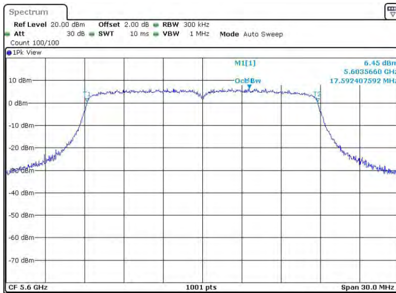
11N20MIMO_Ant2_5600
