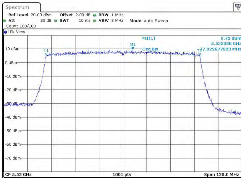
11AC80MIMO_Ant2_5530
