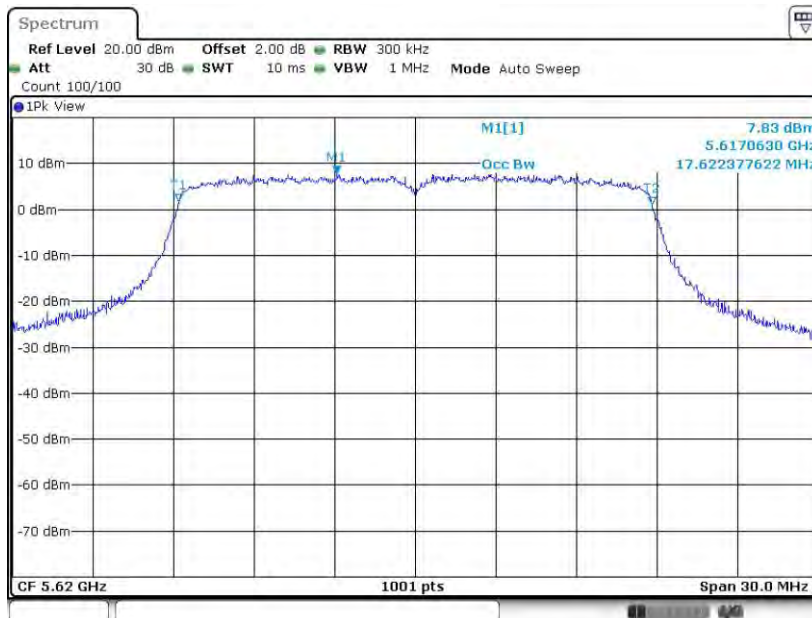
11N20MIMO_Ant1_5620
