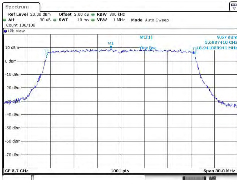
11AX20MIMO_Ant2_5700
