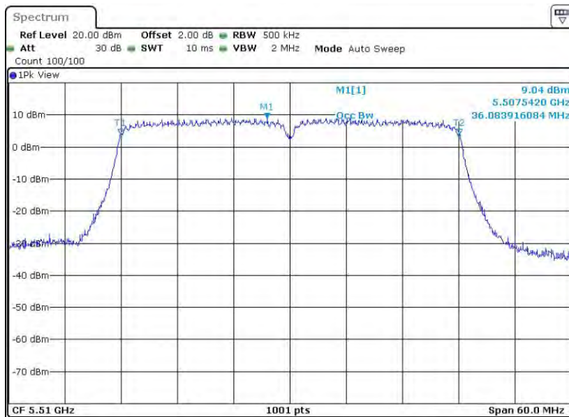
11N40MIMO_Ant2_5510
