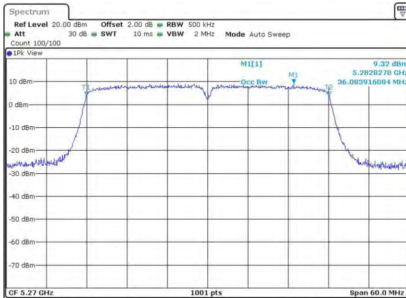
11AC40MIMO_Ant1_5270
