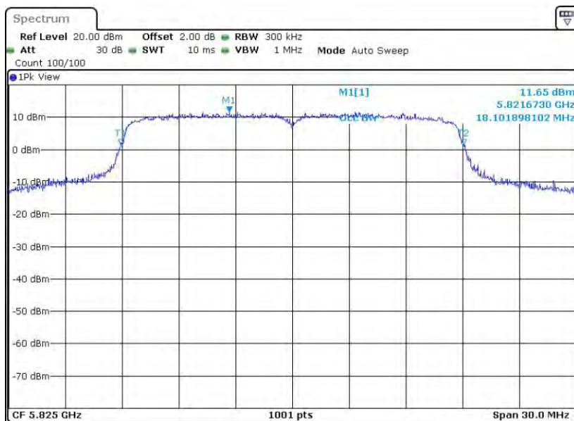
11N20MIMO_Ant1_5825
