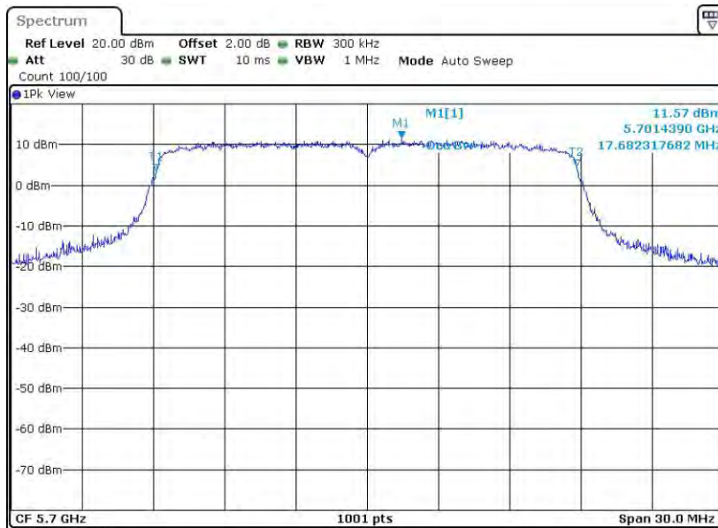
11N20MIMO_Ant1_5700
