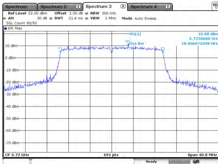
11AX20MIMO_Ant1_5720
