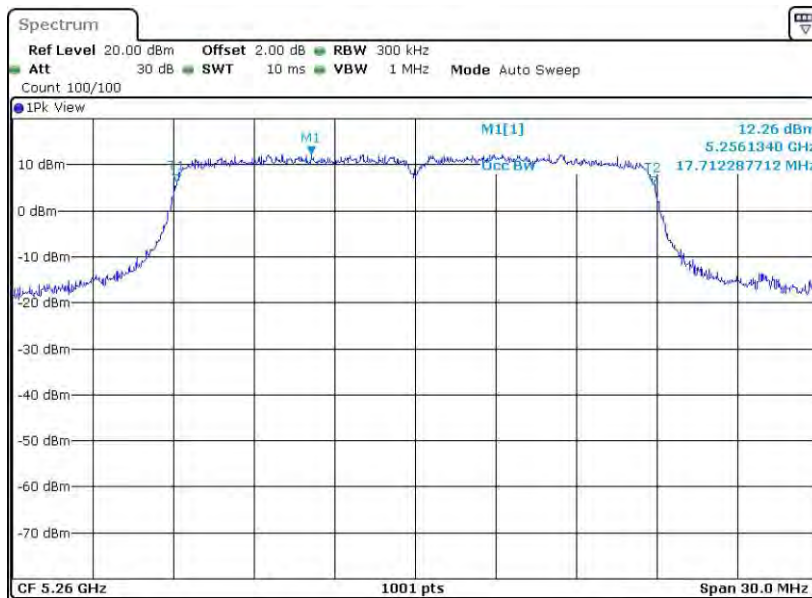
11N20MIMO_Ant2_5260
