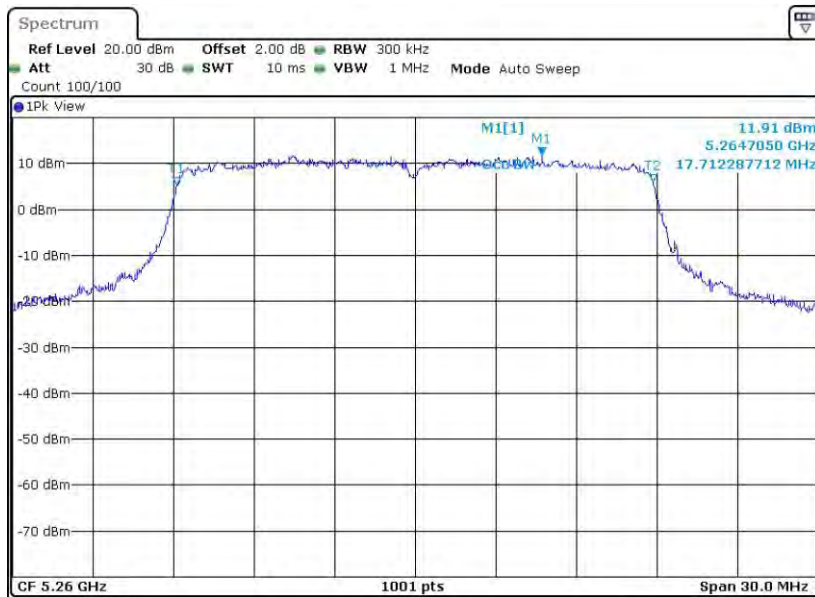
11AC20MIMO_Ant1_5260
