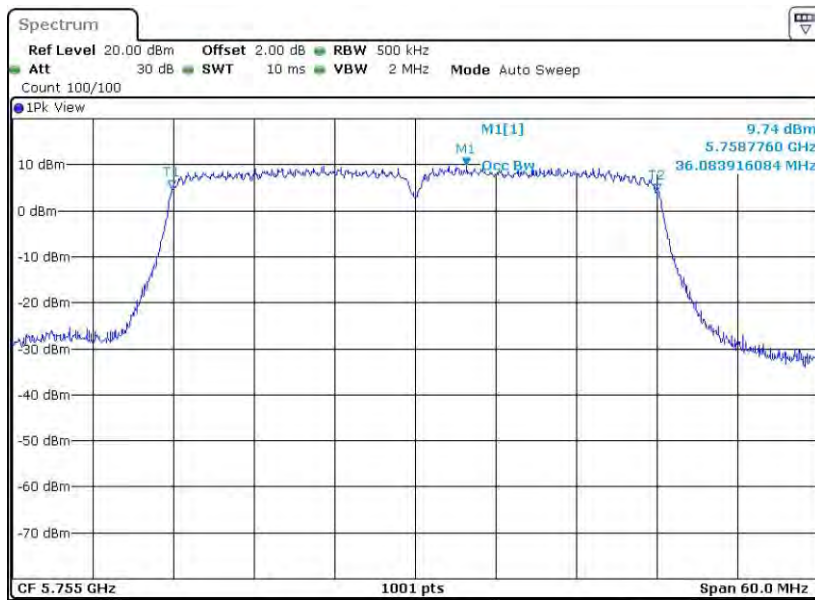
11N40MIMO_Ant2_5755
