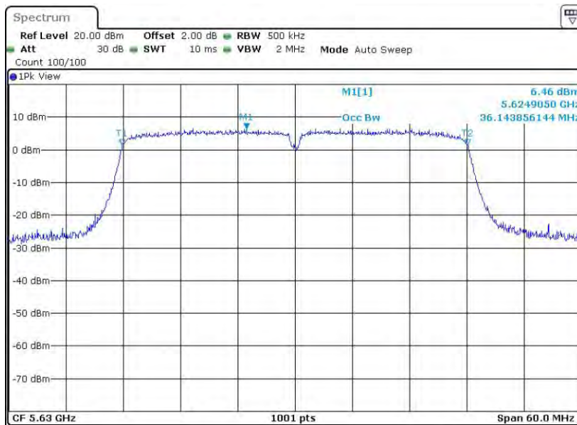
11N40MIMO_Ant2_5630
