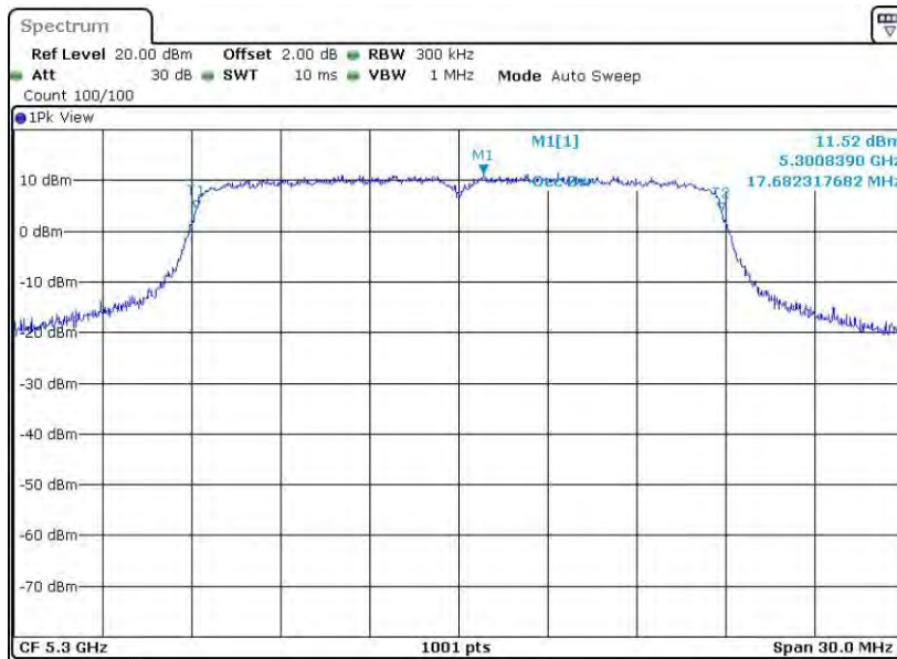
11N20MIMO_Ant1_5300
