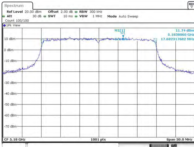
11AC20MIMO_Ant1_5180
