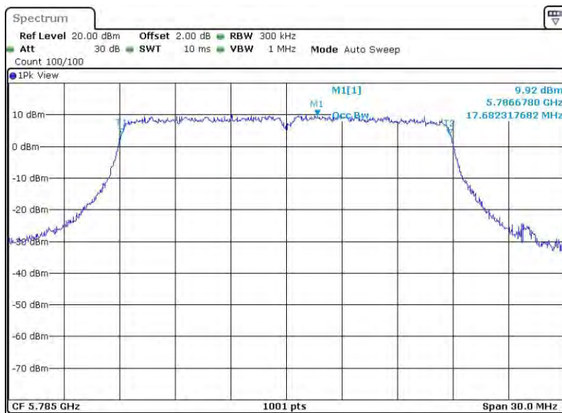
11N20MIMO_Ant2_5785
