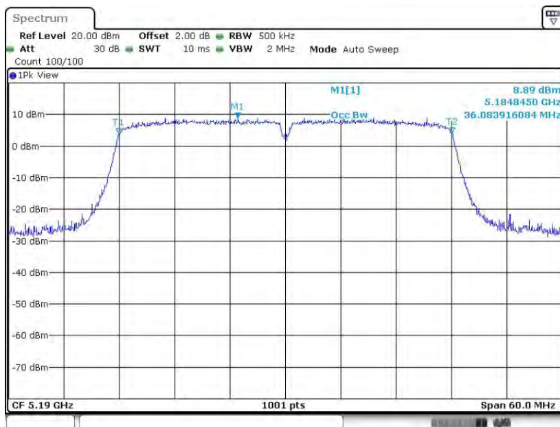
11N40MIMO_Ant1_5190
