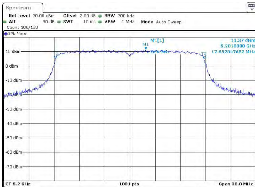
11N20MIMO_Ant2_5200
