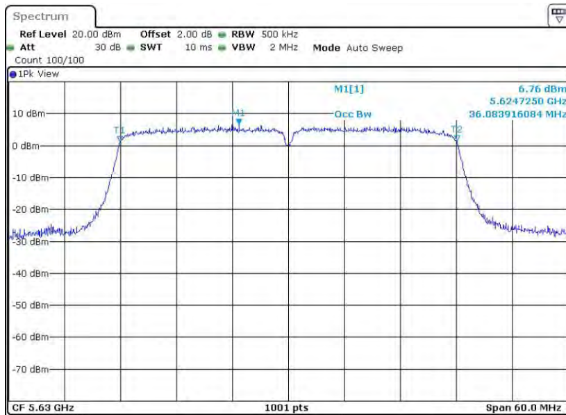
11N40MIMO_Ant1_5630
