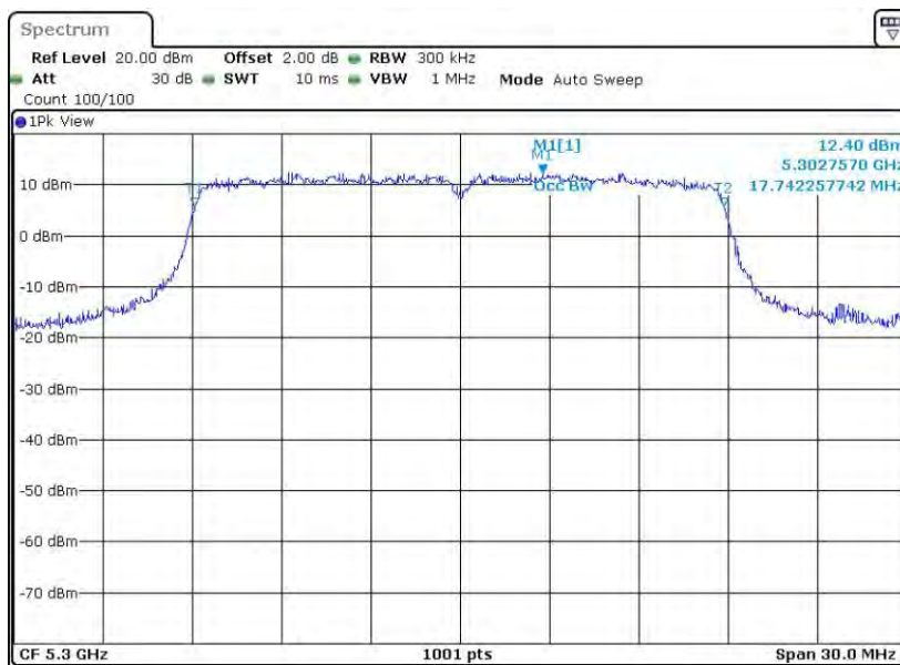
11N20MIMO_Ant2_5300
