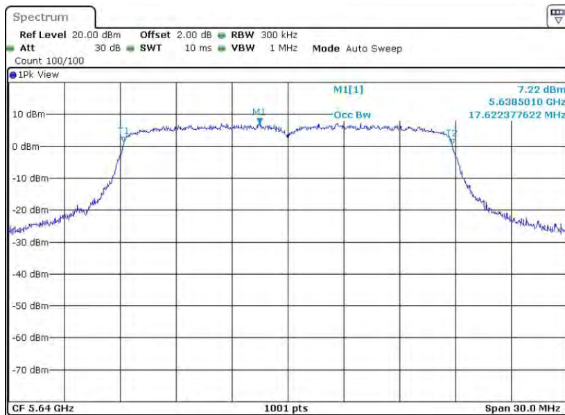
11AC20MIMO_Ant2_5640
