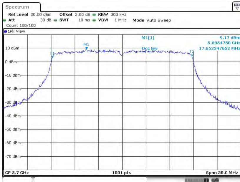
11AC20MIMO_Ant1_5700
