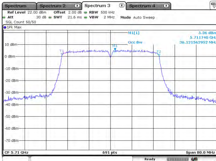
11N40MIMO_Ant1_5710
