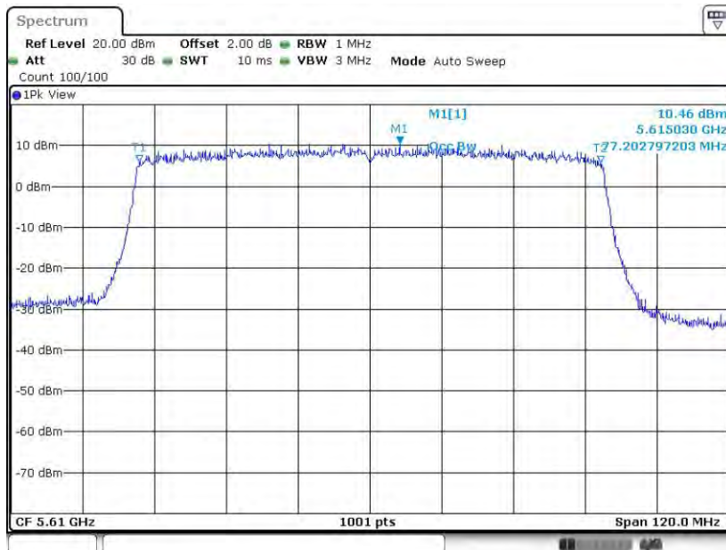
11AC80MIMO_Ant1_5610
