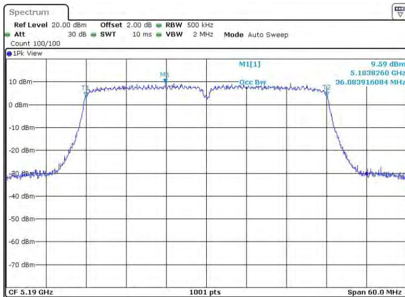
11N40MIMO_Ant2_5190
