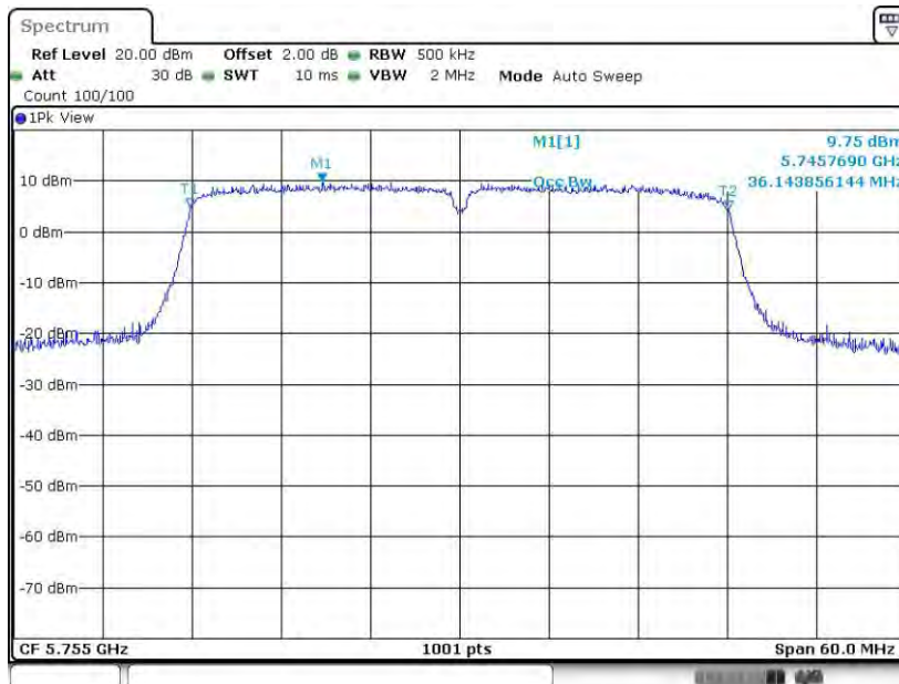
11N40MIMO_Ant1_5755
