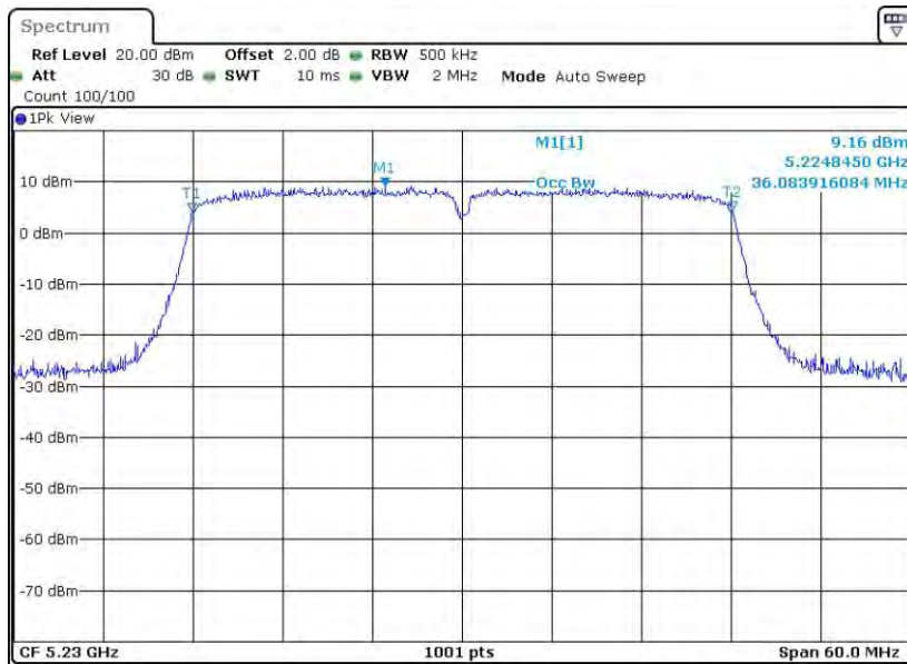
11N40MIMO_Ant1_5230
