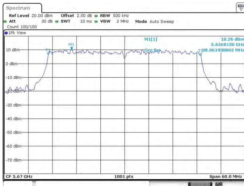
11AX40MIMO-484T Ant1 5670
