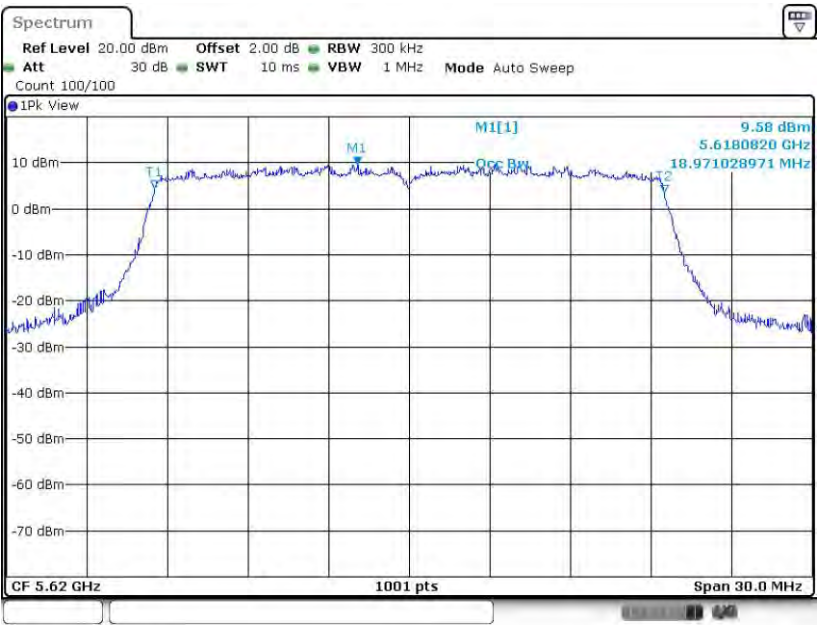
11AX20MIMO-242T_Ant2_5620
