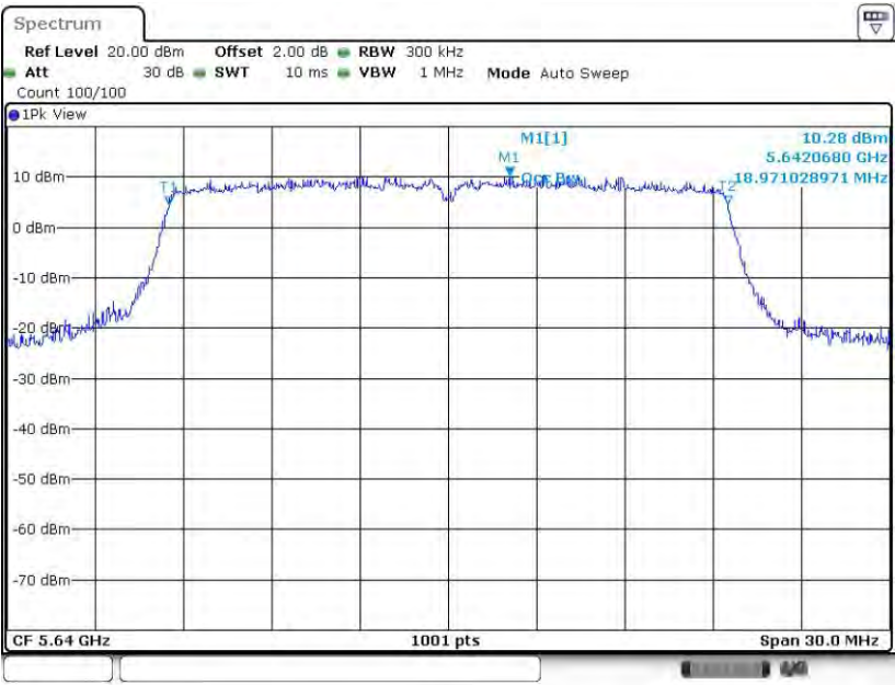
11AX20MIMO-242T_Ant1_5640
