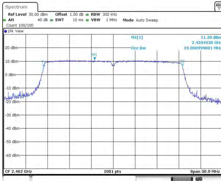
11AX20MIMO-242T Ant1 2462
